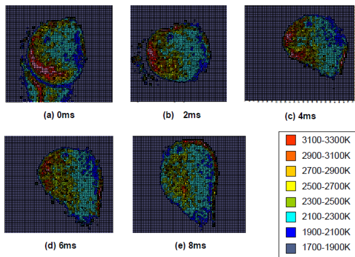
FIGURE 1.26 – Champ de température d’une gouttelette dans un arc MAG (330A) [64]
