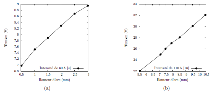
FIGURE 1.15 – Relation entre la hauteur d'arc ( mm ) et la tension ( V ) obtenues par Binard et al. [30] (a) et Evans et al. [31] (b) (figure de [32])
