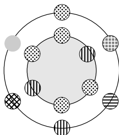
FIG. III.21. Une solution avec un cercle extérieur composé de 6 couleurs.
