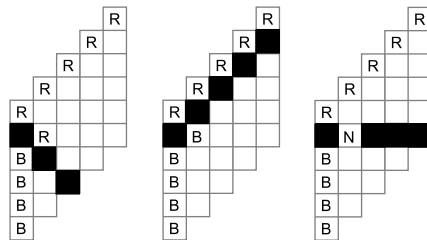
FIG. B.17. Frontières en fonction de la couleur du point horizontalement adjacent
