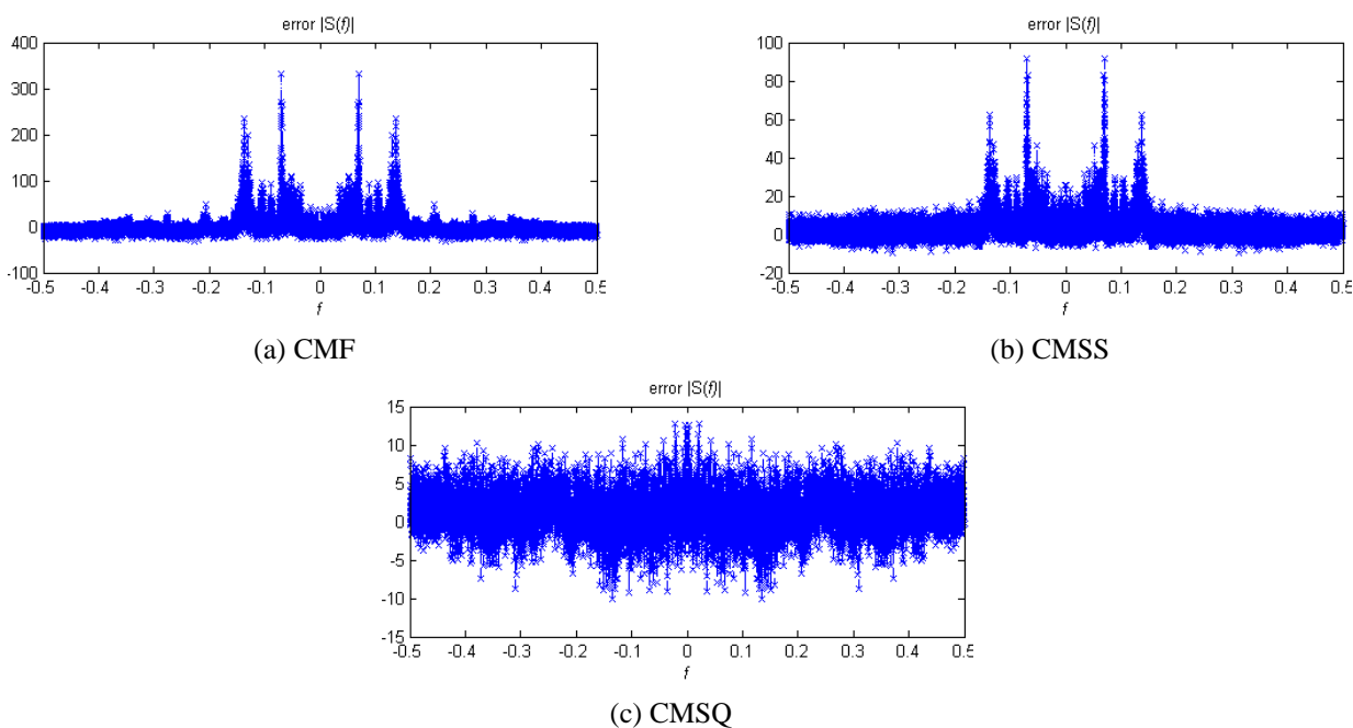
Figure 3-22 L'erreur entre la TF du signal reconstruit compressé à 0.05 bpp par JPEG2000 et la TF du signal initiale.
