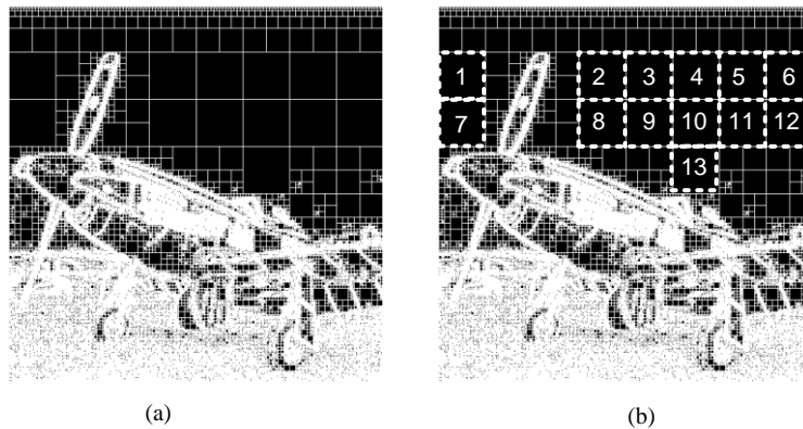
Figure 2-27 (a) La décomposition en quadtree de l'image d'erreur (b) les nœuds voisins de même taille ont été choisis (64x64 pixels) pour construire la LR_0 comme région d'insertion.
