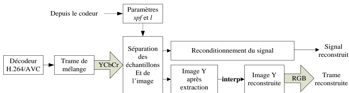
Figure 4-9 Schéma de bloc résumant la procédure de décodage
