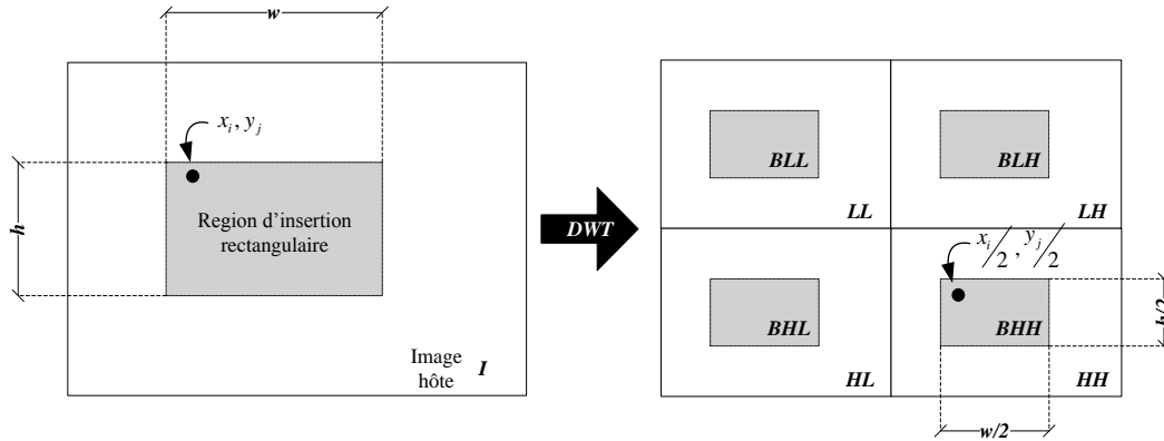
Figure 2-11 Présentation de quatre-bandes de fréquences de la décomposition en ondelette. La région d'insertion sélectionnée correspond aux régions ( BLL , BLH , BHL et BHH ) sur la décomposition dyadique
