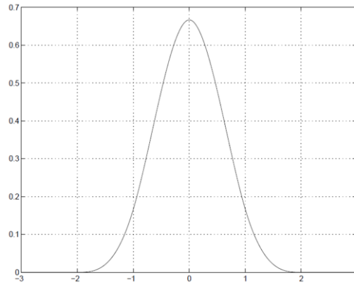
Figure A-2 La fonction de synthèse B-spline cubique.
