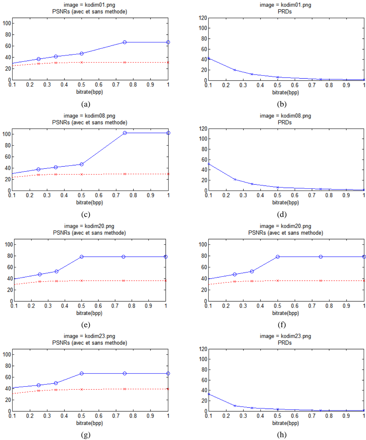
Figure 3-11 Evaluation de la méthode CMSS avec la compression seule de l'image par JPEG2000 pour des différents bitrate choisis. (a)-(b) kodim01, (c)-(d)- kodim08, (e)-(f) kodim20, (g)-(h) kodim23. Sur la Figure (o) dénote le PSNR direct et (x) le PSNR méthode
