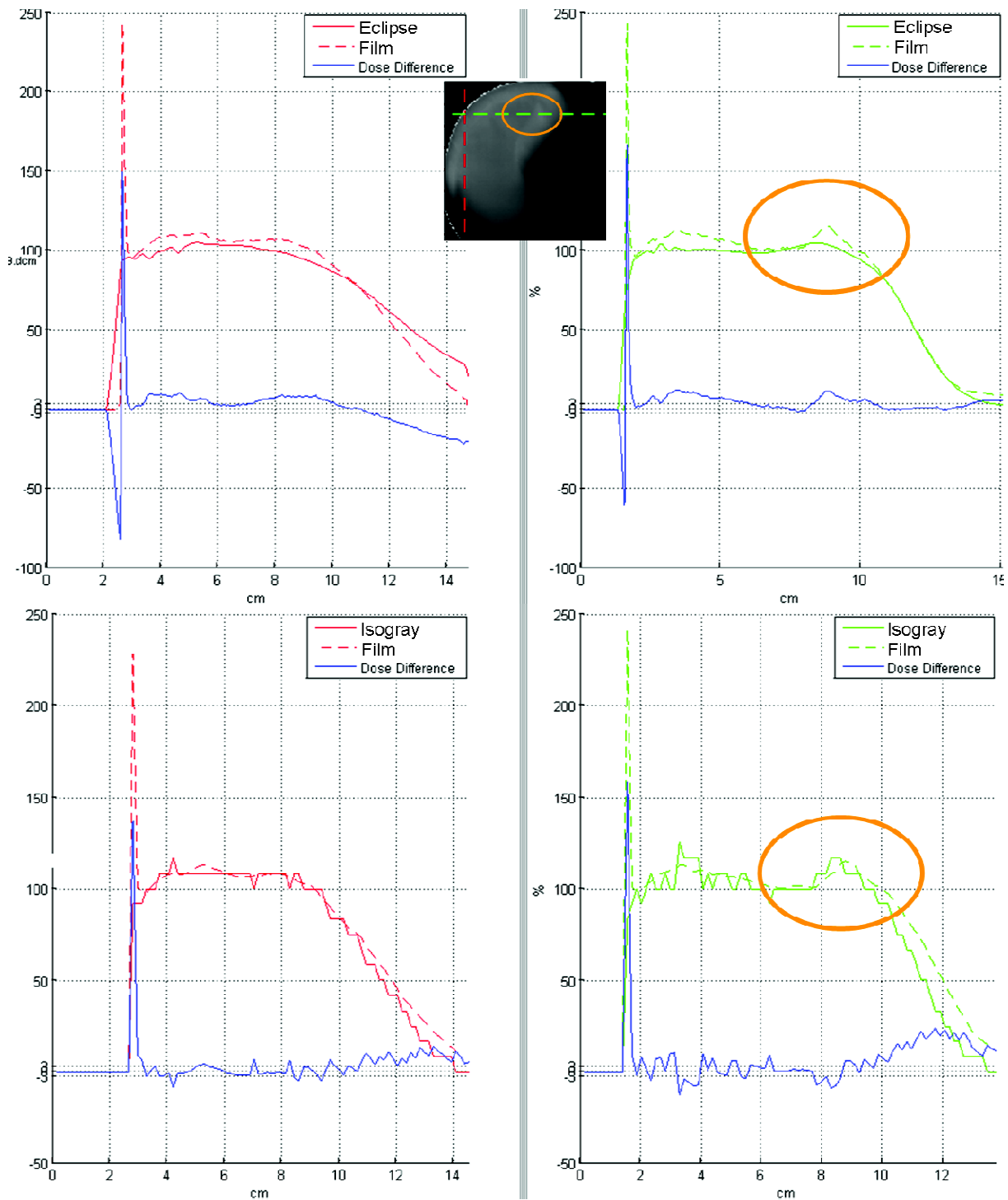
Figure 53 : Comparaison 1 des profils de dose mesurés (film EBT) et calculés (PB Eclipse et MC Isogray) du test CIRS – Paroi - niveau 3 – 12 MeV. Les pics de dose sont dus au découpage imparfait du film en bordure du fantôme.
