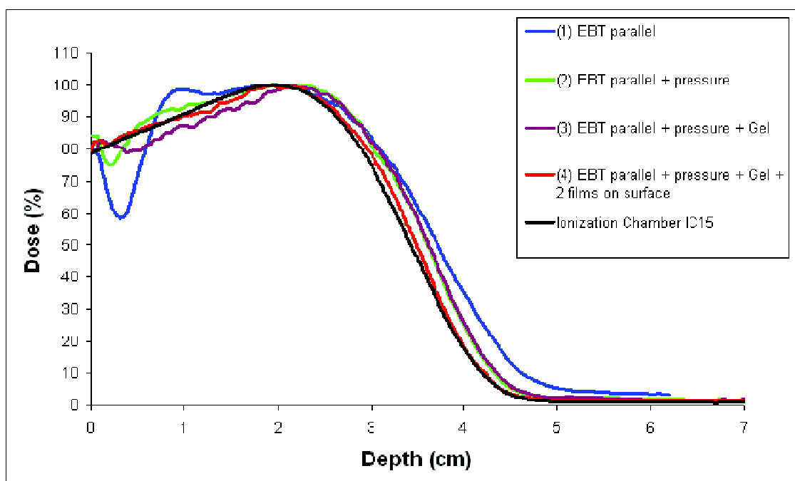
Figure 9 : Rendements en profondeur mesurés avec les films Gafchromic® EBT positionnés parallèlement à un faisceau d'électrons de 9 MeV pour différents montages. Le champ fait 10 × 10 cm 2 et la DSP 100 cm.
