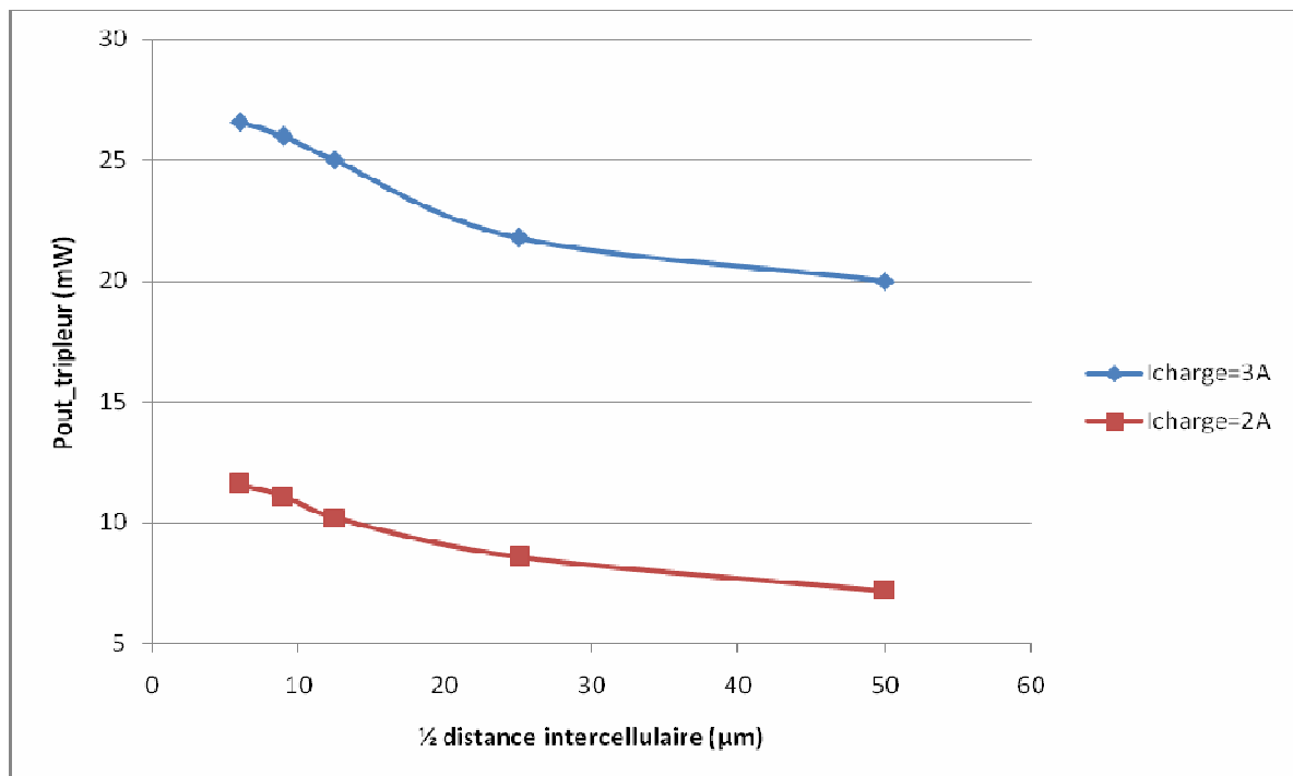
figure 9: Puissance de sortie du tripleur en fonction de la \frac{1}{2} distance intercellulaire
