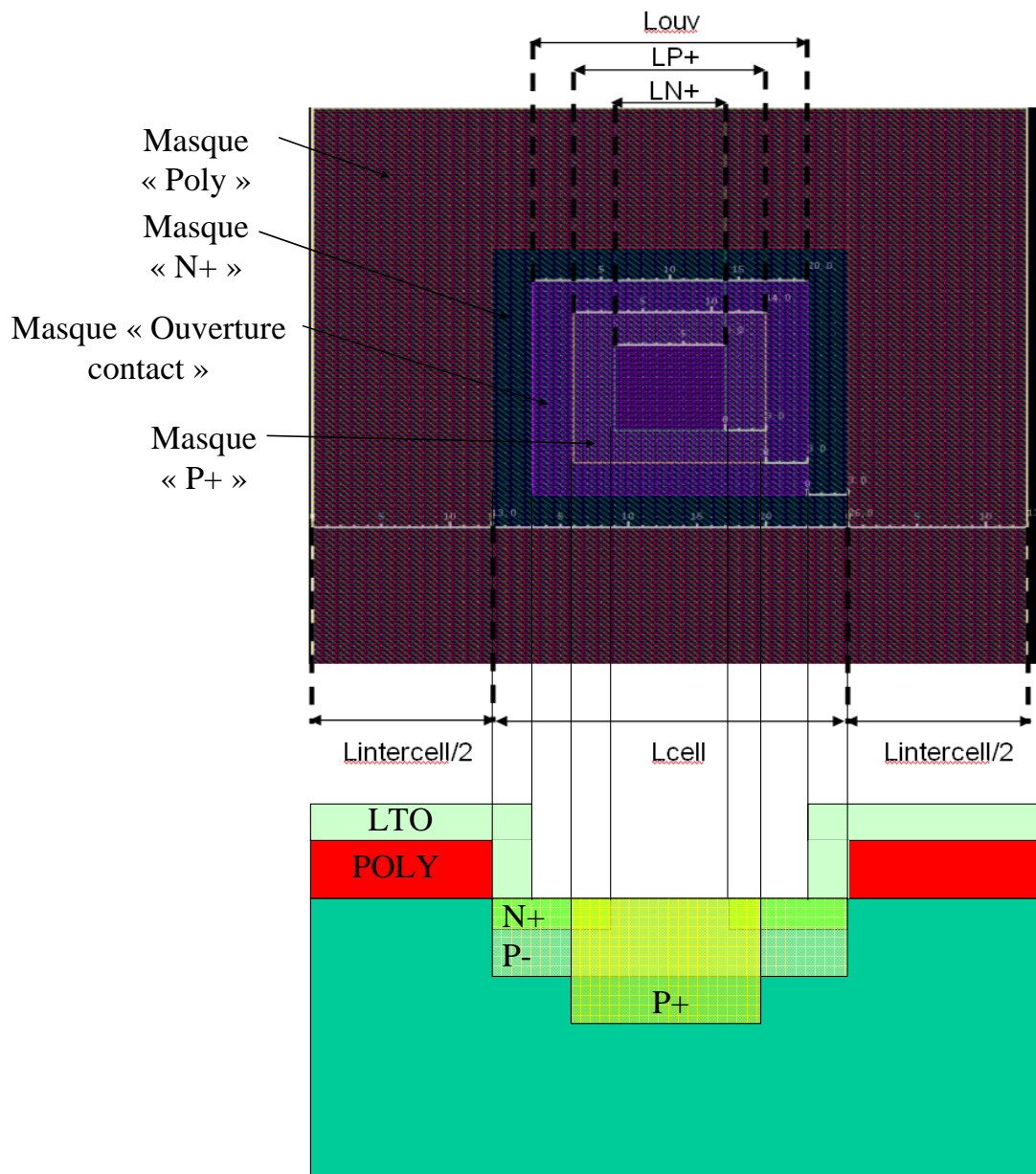
figure 6: Vue des masques de la cellule élémentaire et de ses dimensions et vue en coupe correspondante
