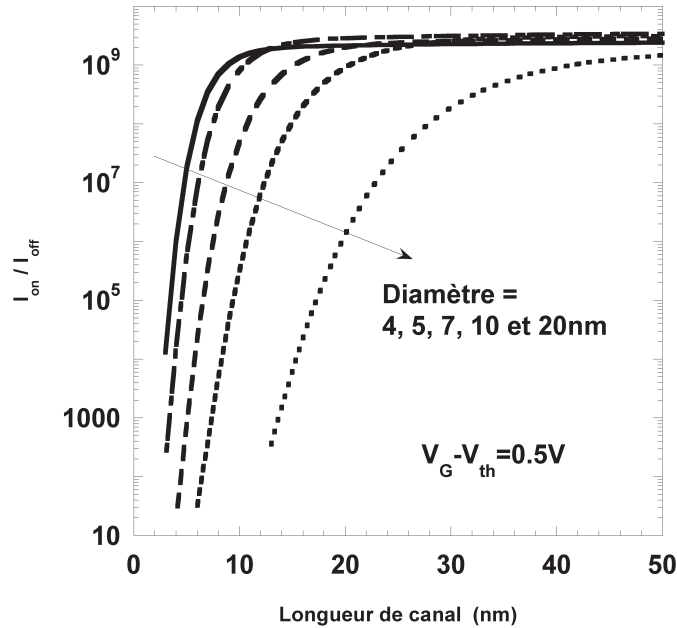
FIGURE 7.11: Ratio I_{ON}/I_{off} en fonction de la longueur de canal pour différents diamètres de fils en régime d'inversion forte (pour le I_{ON} ).
