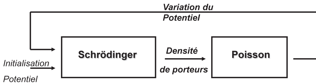
FIGURE 1.2: Principe de résolution numérique auto-cohérente des équations de Schrödinger et de Poisson
