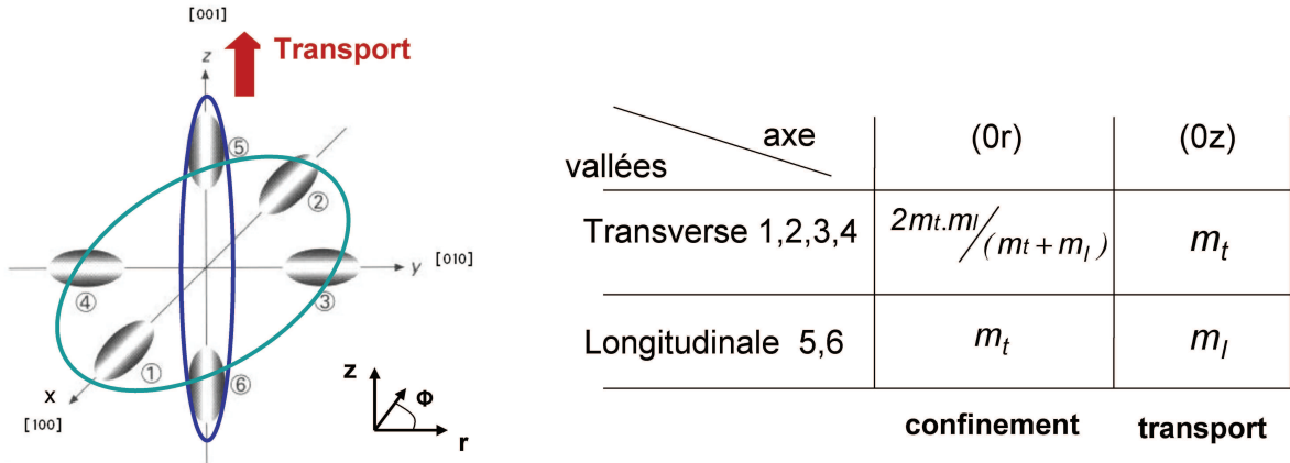
FIGURE 4.7: Définition des masses longitudinales et transverses pour les six vallées du silicium orienté \langle 100 \rangle dans l'approximation d'un système isotropique.
