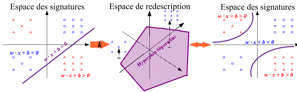
FIGURE 4.1 – Classification linéairement séparable entre les \triangle (exemples de classe positive) et les \square (exemples de classe négative). L'hyperplan séparateur est défini par w \cdot x + b = 0 . La décision est donnée par le signe de w \cdot x + b . Les exemples situés sur les deux lignes discontinues sont des vecteurs support (SV). La marge \sigma est la distance minimale des SV à l'hyperplan.
