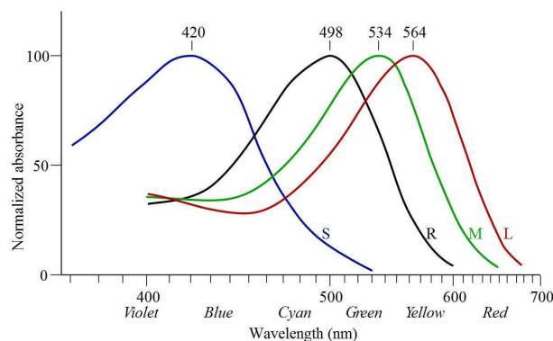
FIGURE 3.4 – Courbes d'absorbance des cônes et des bâtonnets pour l'Homme. Source wikipedia..
