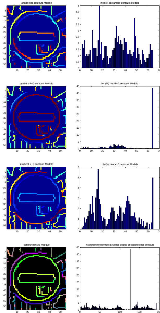
FIGURE 5.7 – Création de la signature des angles et couleurs dans la fenêtre du modèle de la Fig. 5.3. Les trois premières lignes correspondent respectivement à l'angle du gradient, au gradient R - G et au gradient Y - B , contenus dans l'image de gauche. La colonne de gauche montre les plans correspondants. Celle de droite montre l'histogramme normalisé de ces valeurs. Sur la dernière ligne : à gauche, les trois plans forment une image ; à droite l'histogramme qui représente la signature finale, concaténation des trois histogrammes précédents.
