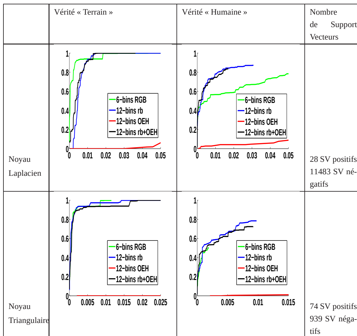
FIGURE 5.24 – Comparaison des courbes ROC obtenues sur l'image originale de la Fig. 5.5, avec différents types de signatures : Histogramme des couleurs RGB ( 6^3 -bins), Histogramme des couleurs normalisées rb ( 12^2 -bins), Histogramme des orientations du contour (12-bins), Histogramme de la concaténation des couleurs rb ( 12^2 -bins) et des orientations du contour (12-bins). Dans la colonne de gauche, la carte de vérité est celle des panneaux de « sens interdit » tandis que à droite, c'est celle des détections en tâche de recherche issue de l'expérimentation. Sur la première ligne, le noyau Laplacien est utilisé, tandis que dans la seconde, c'est le noyau triangulaire.
