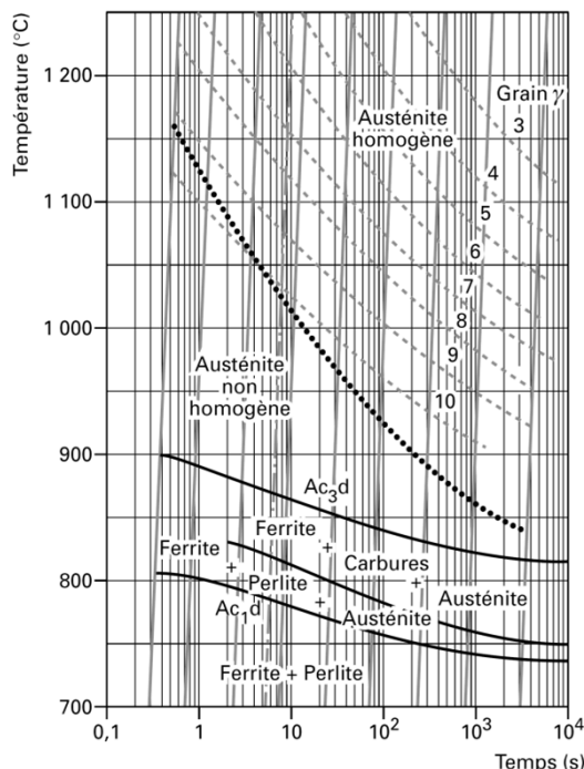
Figure 2-7 Diagramme de transformation en chauffage continu d'un acier du type 35 CrMo4 (Orlich, et al. , 1973).
