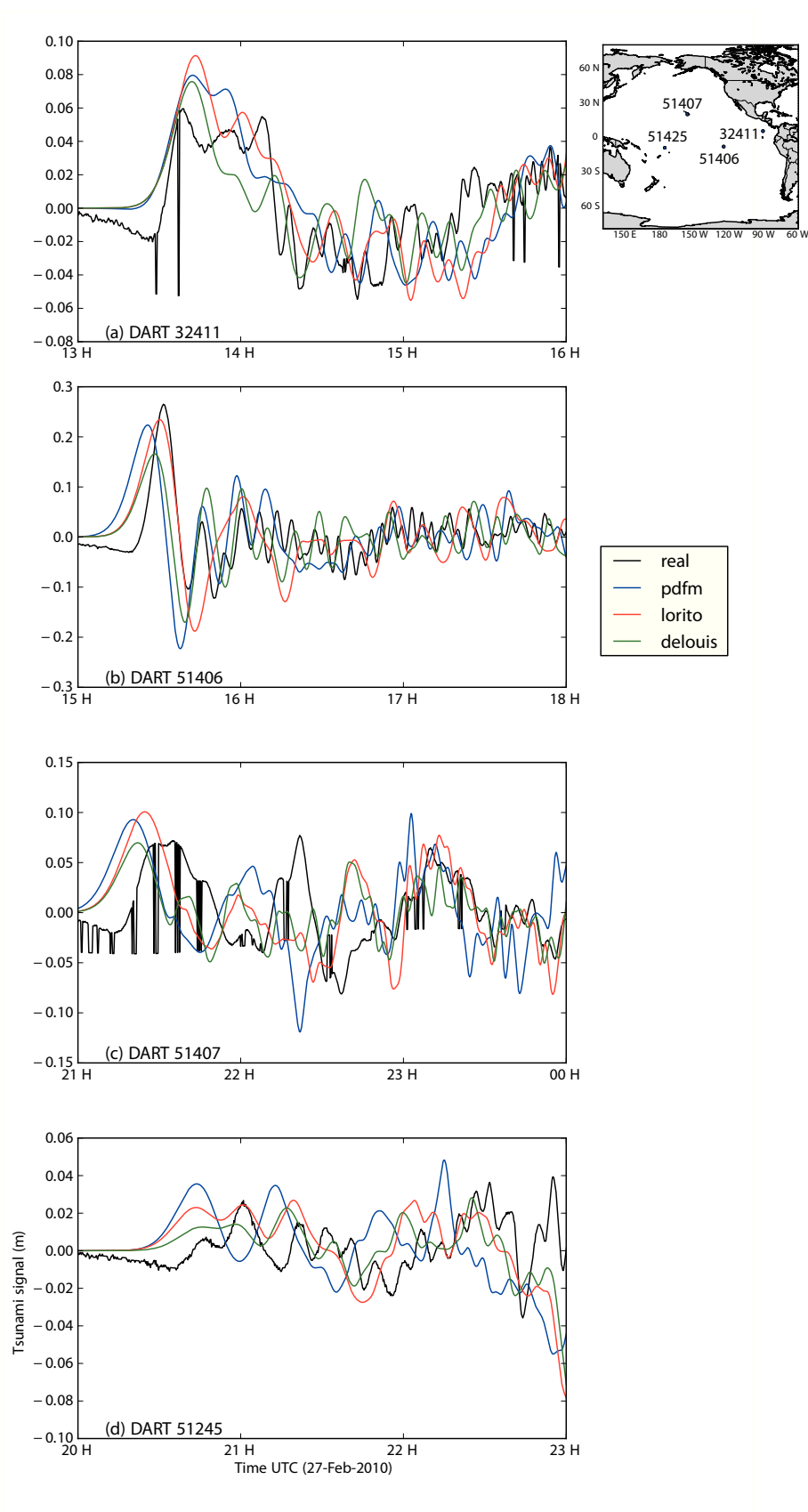
Figure 3.3 ► Comparaison entre les signaux DART observés et simulés pour 4 stations, (a) Nord du Pérou, (b) Polynésie française, (c) Hawaii, (d) Nouvelle Zélande.
