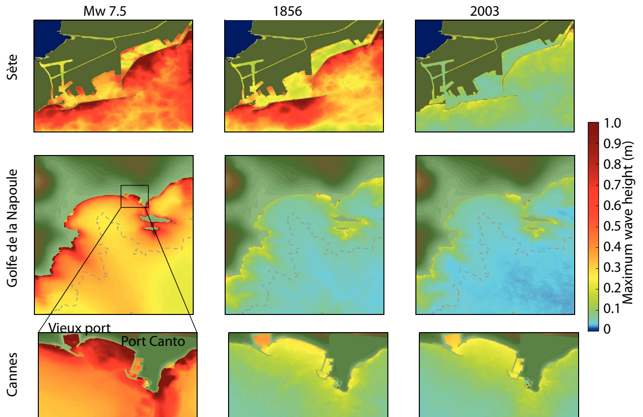
Figure 4.10 ► Détail sur les sites de Sète et de Cannes pour les trois évènements étudiés.
