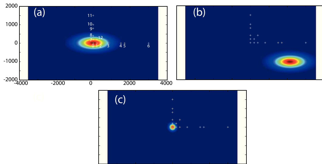
Figure 2.14 ► Représentation du bassin de calcul de modes de résonance (bassin rectangulaire de dimension 7 km x 4 km et 100 m de profondeur) la position des différents capteurs est représentée par des "+". Trois simulations ont été effectuées avec trois configurations de surface initiale de déformation : (a) source centrée, (b) source décentrée, (c) source centrée de faible taille comme le préconise Yalciner & Pelinovsky (2007)
