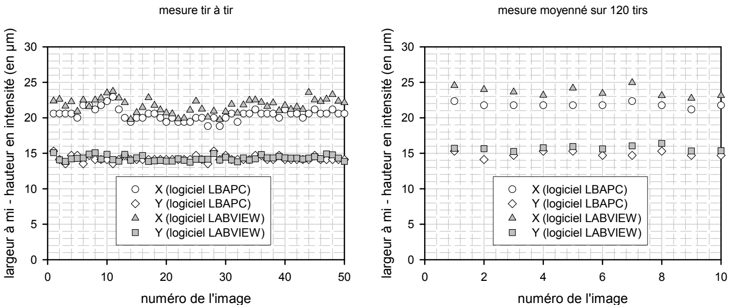
Figure C-2 : Largeur à mi – hauteur de la tâche focale pour une énergie IR de 5 mJ.
