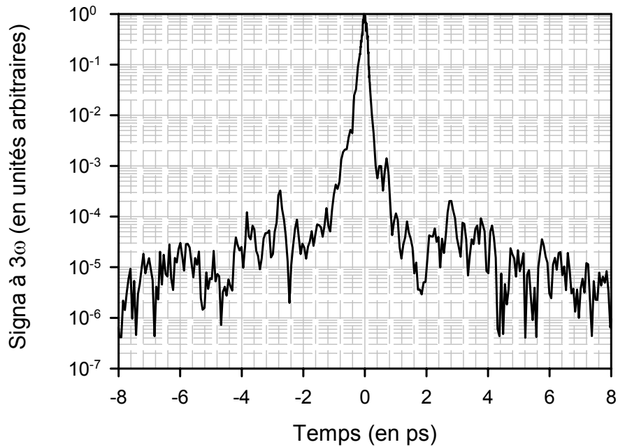
Figure II-20 : Trace de corrélation obtenue sur la voie femto 2 du LUCA par le cross corrélateur du DRECAM début 2002.
