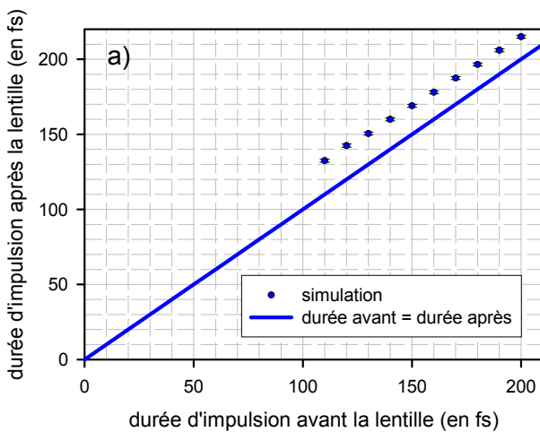
Figures II-12 : Estimation de la durée d'impulsion après la lentille (a) ainsi que de la correction (en %) qui en résulte (b) en fonction de la durée d'impulsion initiale pour une longueur d'onde de 400 nm.
