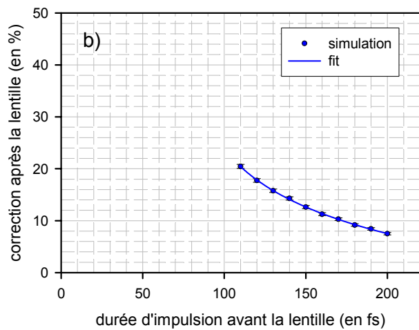
Figures II-12 : Estimation de la durée d'impulsion après la lentille (a) ainsi que de la correction (en %) qui en résulte (b) en fonction de la durée d'impulsion initiale pour une longueur d'onde de 400 nm.
