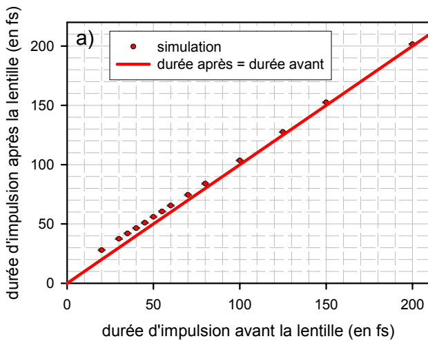
Figures II-11 : Estimation de la durée d'impulsion après la lentille (a) ainsi que de la correction (en %) qui en résulte (b) en fonction de la durée d'impulsion initiale pour une longueur d'onde de 800 nm.
