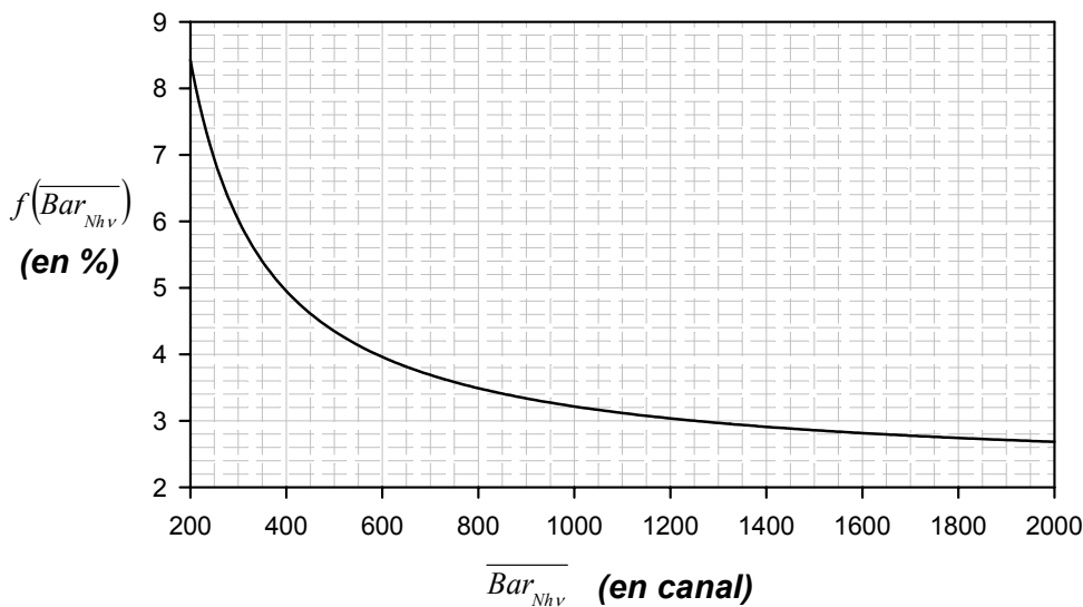
Figure III-23 : Incertitude relative sur le taux moyen de photons X détectés f(\overline{Bar}_{Nh\nu}) en fonction du barycentre de l'empilement sur le détecteur Si(Li) (1).
