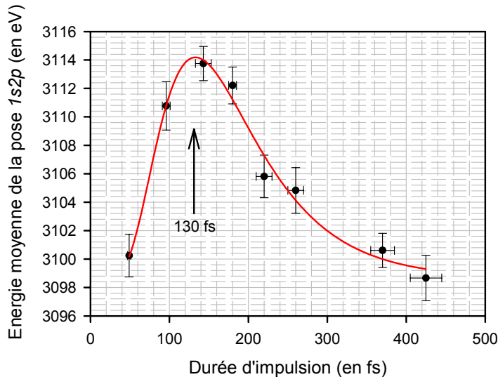
Figure IV-37 : Évolution de l'énergie moyenne des poses 1s2p lors des études en fonction de la durée d'impulsion à éclairement constant ( P_0 = 30 \text{ bars} , \lambda = 800 \text{ nm} I \sim 8 \times 10^{15} \text{ W/cm}^2 ).
