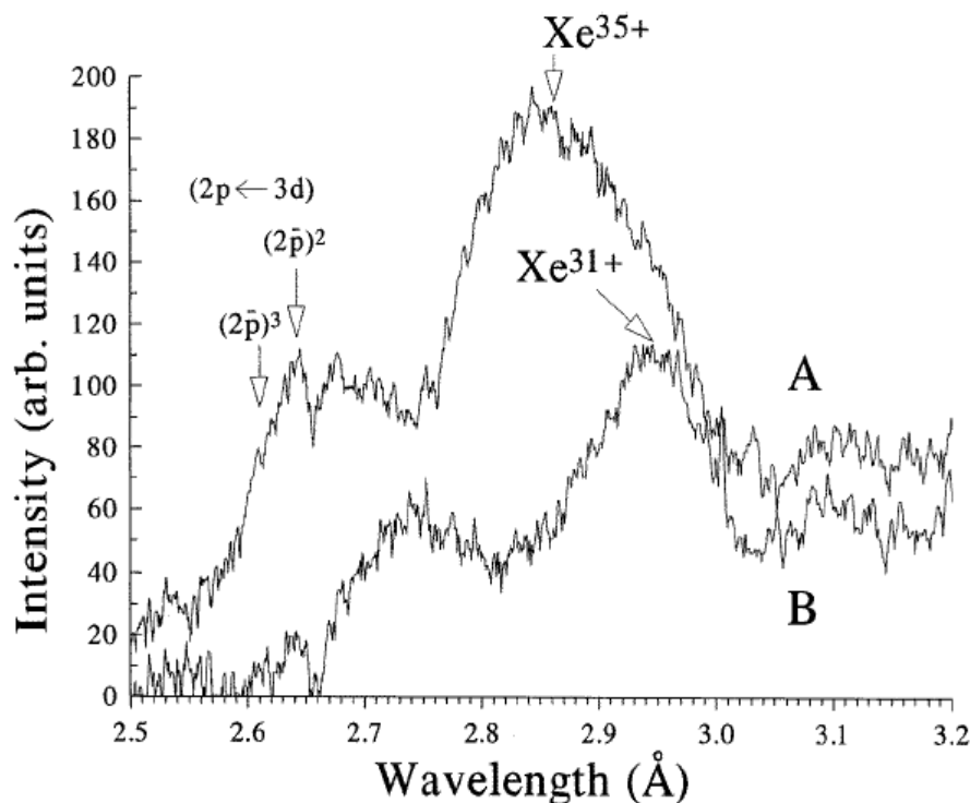
Figure I-61 : Spectre d' X_L dans la région 2,4 – 3,3 Å (soit 3,8 – 5,2 keV) pour \lambda = 248 nm et pour deux intensités différentes : I_A \sim 8 \times 10^{18} W/cm 2 et I_B \sim 4 \times 10^{18} W/cm 2 [Borisov et al., 1996].
