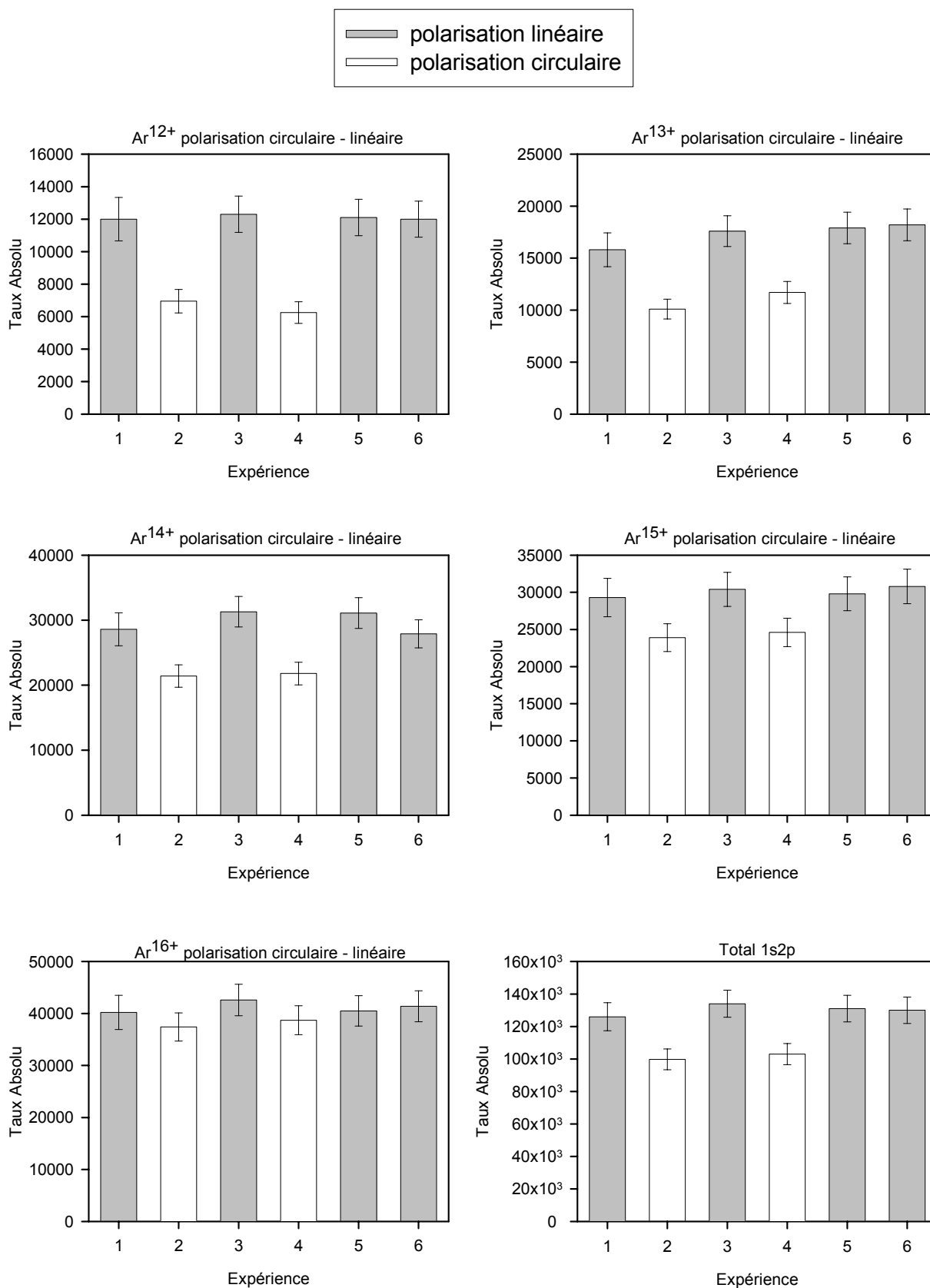
Figure IV-4 : Taux absolu (en nombre de photons X dans 4\pi et par tir laser) des différents états de charge pour les expériences réalisées en polarisation linéaire et circulaire dans le cas des agrégats d'argon.
