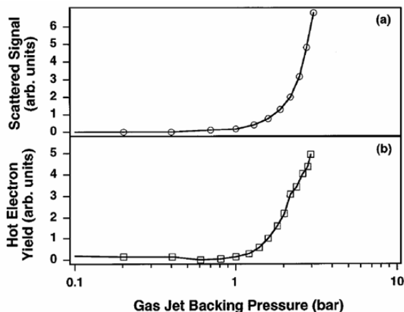
Figure I-25 : a) Signal Rayleigh diffusé en fonction de la pression amont de Xe b) Taux d'électrons énergétiques en fonction de la pression amont pour un éclairement de 10^{16} W/cm 2 [Shao et al., 1996].
