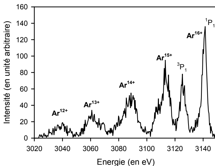
Figure III-24 : Exemple de spectre brut haute résolution obtenu lors de l'irradiation d'agrégats d'argon : transitions 1s2pnl \rightarrow 1s^2nl de l'Ar 12+ à l'Ar 16+ ( N_{\text{tirs laser}} = 20\,000 ).
