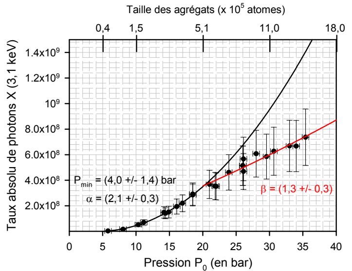
Figure IV-19 : Évolution du taux absolu de photons X_K de l'argon en fonction de la pression en amont de la buse condensation (pour les conditions expérimentales voir le Tableau IV-11).
