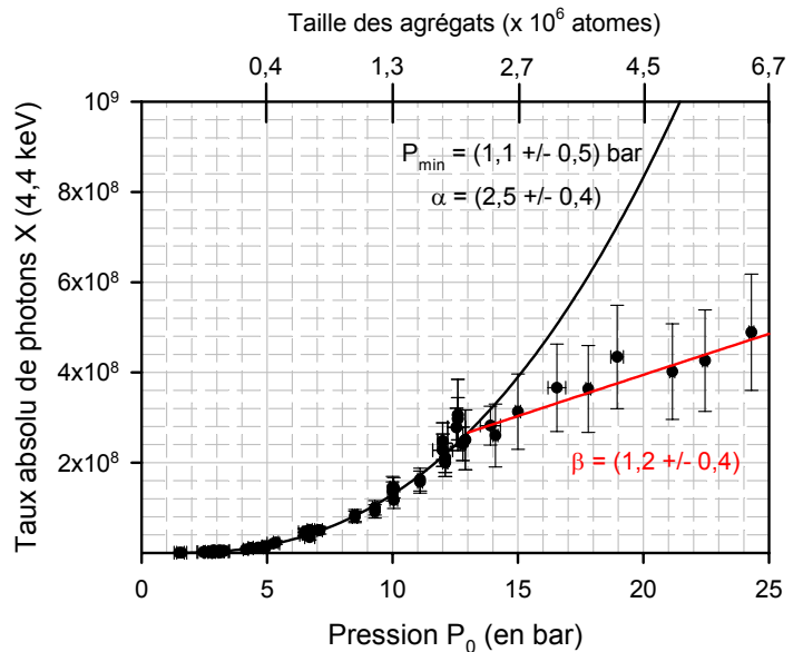
Figure IV-20 : Évolution du taux absolu de photons X_L du xénon en fonction de la pression en amont de la buse condensation (pour les conditions expérimentales voir le Tableau IV-11).
