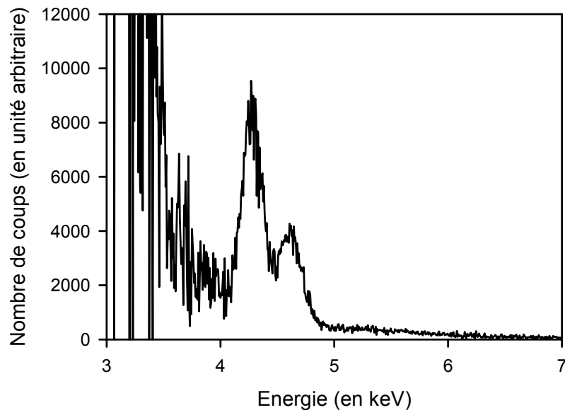
Figure III-20 : Spectre monophotonique sur le détecteur Si(Li) (1) corrigé de la transmission du filtre d'inox de 23,20 µm (2 feuilles de 11,60 µm). Agrégats de xénon ( P_0 = 10,7 bars - E = 5 mJ - \lambda = 400 nm).
