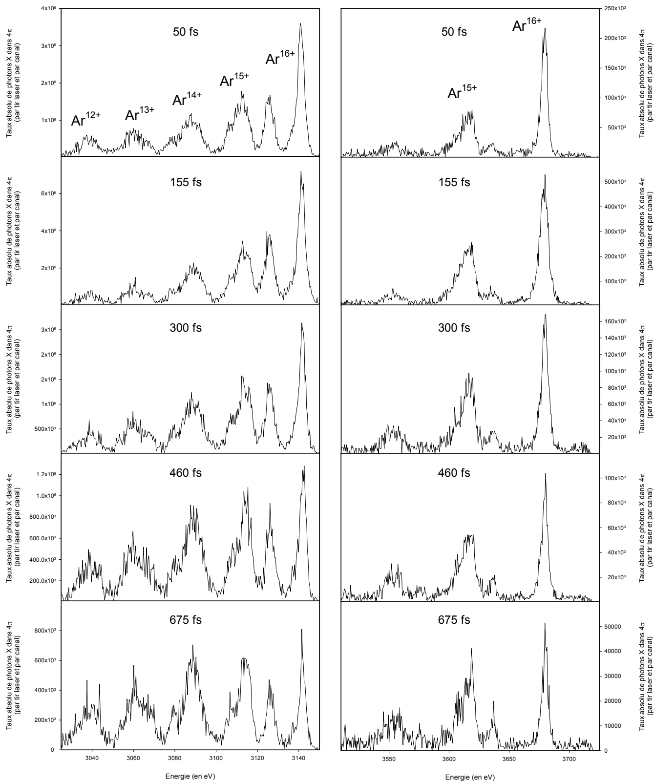
Figure IV-33 : Spectres X haute résolution (poses 1s2p et 1s3p) obtenus lors de l'irradiation d'agrégats d'argon en fonction de la durée d'impulsion ( P_0 = 30 bars, E = 20 mJ et \lambda = 800 nm).
