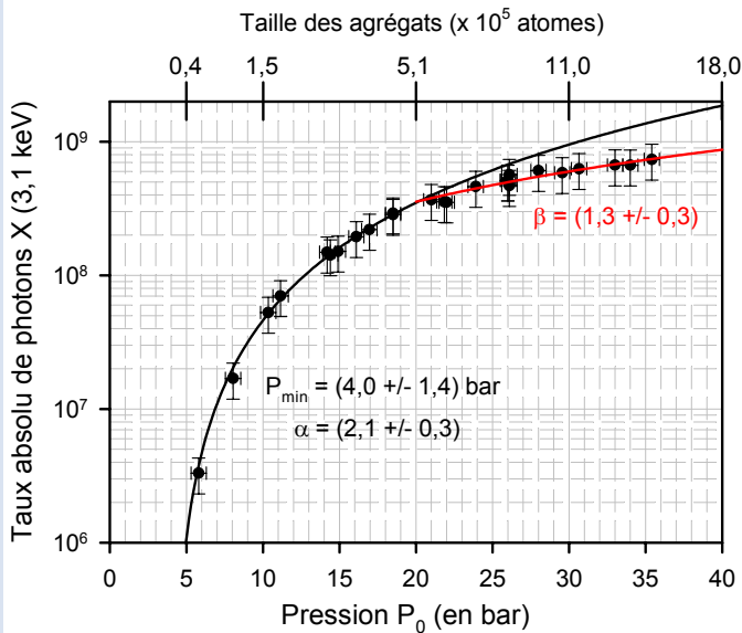
Figure IV-19 : Évolution du taux absolu de photons X_K de l'argon en fonction de la pression en amont de la buse condensation (pour les conditions expérimentales voir le Tableau IV-11).
