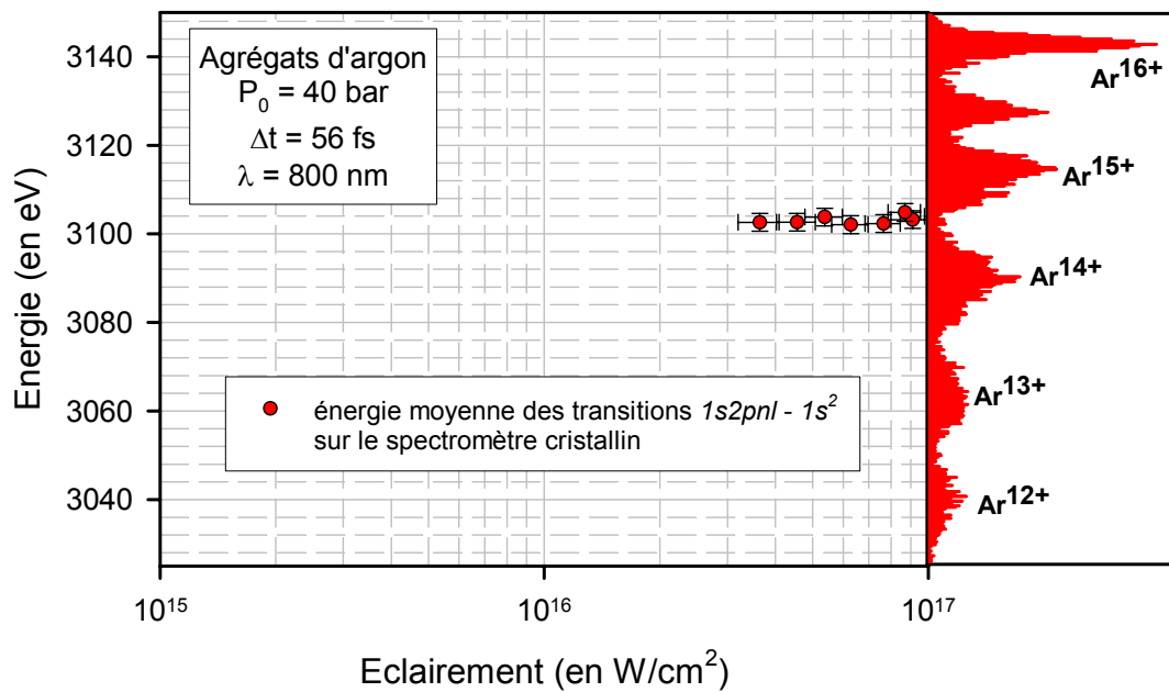
Figure IV-7 : Énergie moyenne des transitions 1s2pnl \rightarrow 1s^2 pour les ions argon ayant un état de charge compris entre 12+ et 16+ et pour un éclairement laser supérieur à quelques 10^{16} \text{ W/cm}^2 (les conditions expérimentales sont présentées dans le Tableau IV-7).
