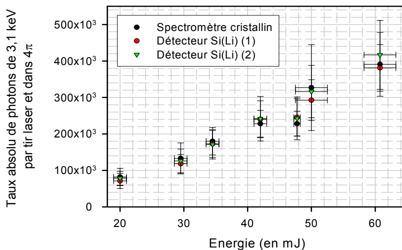
Figure III-37 : Comparaison des taux absolus de photons X calculés à l'aide des trois détecteurs (Si(Li) (1) + Si(Li) (2) + spectromètre cristallin) – Agrégats d'argon, P_0 = 40 bars, \tau = 55 fs et \lambda = 800 nm.
