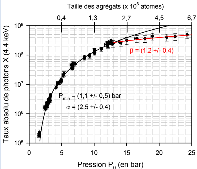
Figure IV-20 : Évolution du taux absolu de photons X_L du xénon en fonction de la pression en amont de la buse condensation (pour les conditions expérimentales voir le Tableau IV-11).
