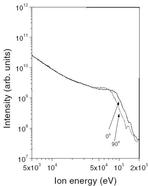
Figure I-42 : Spectre en énergie des ions issus de l'explosion d'agrégats d'argon (contenant de l'ordre de 40 000 atomes soumis à une impulsion de quelques 10^{15} \text{ W/cm}^2 ) pour une direction parallèle et perpendiculaire à l'axe de polarisation du laser [Kumarappan et al., 2001].
