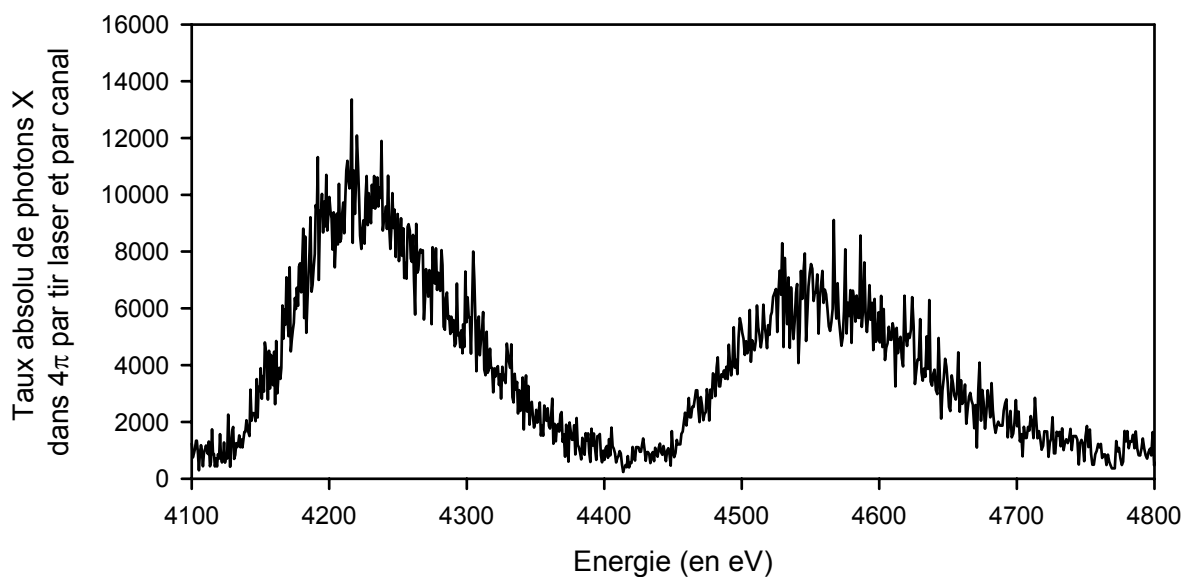
Figure III-36 : Spectre X en absolu issu de l'irradiation d'agrégats de xénon.
