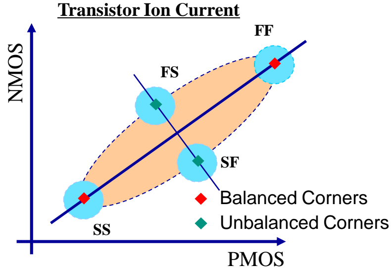
Fig. III: Courant transistor dans la mode saturation pour NMOS et PMOS
