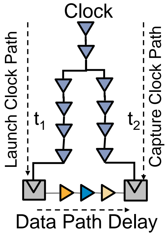
Fig. I: Typiques système synchrone avec les chemins d'horloge et de donne
