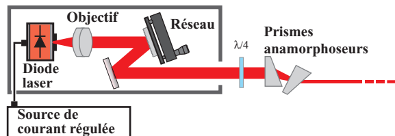
FIG. 1.21 – Diode laser montée avec un réseau.
