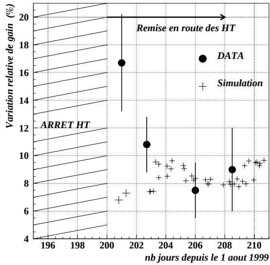
FIG. 3.62 – Variations relatives de la calibration d'anode mesurée et du gain simulé, après remise en route de la Haute Tension d'anode.
