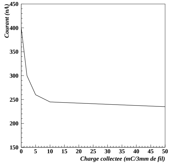
FIG. 3.63 – Vieillissement de fils d'anode dans du CF_4 mesuré par J. Va'vra [50] et [51]
