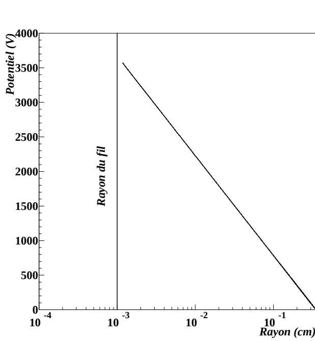
FIG. 3.44 – Potentiel (en volts) en fonction du rayon par rapport au centre du fil d'anode
