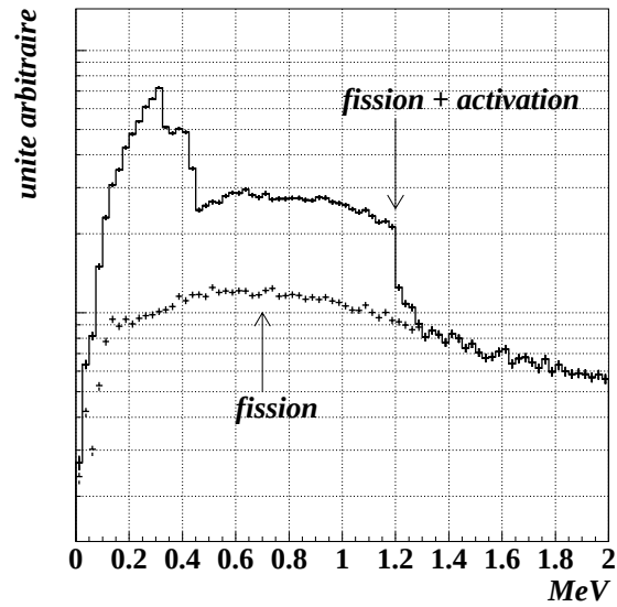
FIG. 2.4 – Spectre global (désintégration des produits de fission + activation) des neutrons pour un burn-up moyen entre 0 et 2 MeV.
