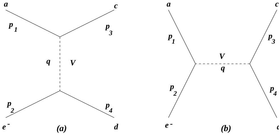
FIG. 1.1 – Diagrammes du premier ordre pour la diffusion a + e^- \rightarrow c + d via le canal t (a) et le canal s (b)
