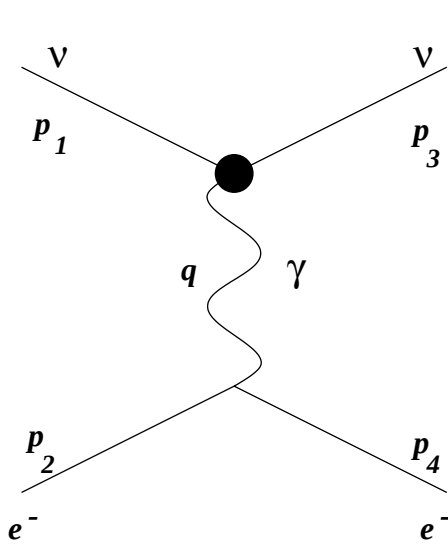
FIG. 1.2 – Diagramme du premier ordre pour la diffusion \nu + e^- \rightarrow \nu + e^- via un courant électromagnétique
