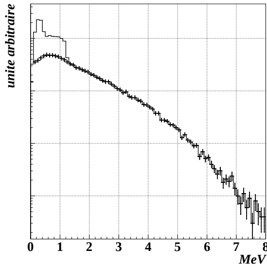
FIG. 2.3 – Spectre global (désintégration des produits de fission + activation) des neutrons pour un burn-up moyen entre 0 et 8 MeV.
