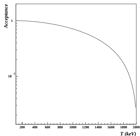
FIG. 2.10 – Acceptance de la TPC aux électrons de reculs provenant d'interaction de neutrinos du réacteur
