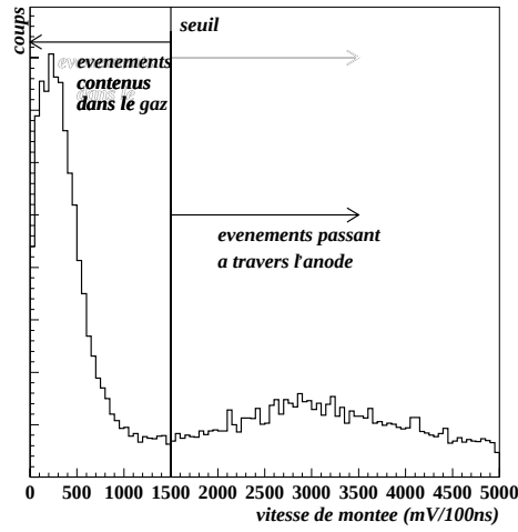
FIG. 5.27 – Distribution des vitesses de montée du signal d'avalanche en lumière pour des électrons simples et des électrons passant à travers l'anode
