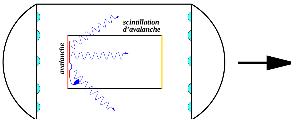
FIG. 4.21 – Signal et caractérisation d'un électron issu d'une diffusion Compton par un gamma externe
