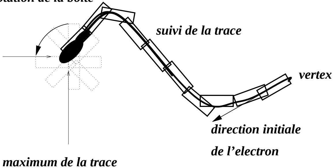
FIG. D.5 – Illustration de l'algorithme existant de recherche de l'angle de diffusion
