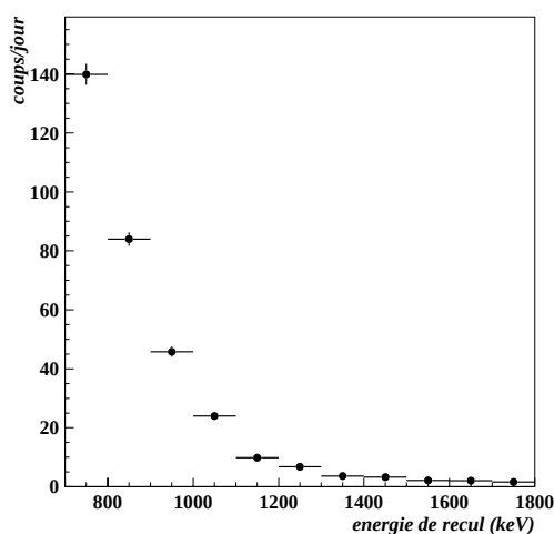
FIG. 5.31 – Spectre des électrons sortant ou entrant sur la paroi latérale de la TPC (entre 09/1999 et 03/2000)
