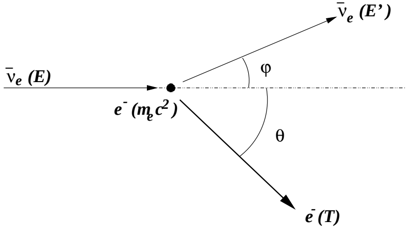
FIG. 1.4 – Schéma de principe de la diffusion neutrino électron
