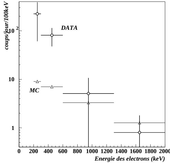
FIG. 1.8 – Spectre des électrons (réacteur ON - réacteur OFF) obtenu en différentiant les quatre mesures fournies dans [11]
