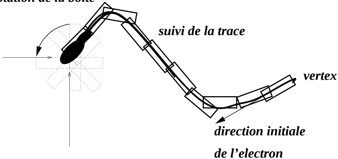
FIG. D.5 – Illustration de l'algorithme existant de recherche de l'angle de diffusion
