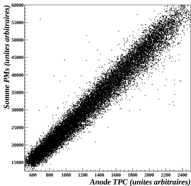
FIG. 3.54 – Comparaison entre les signaux en charge et en lumière d'avalanche pour des électrons de recul dans la TPC.
