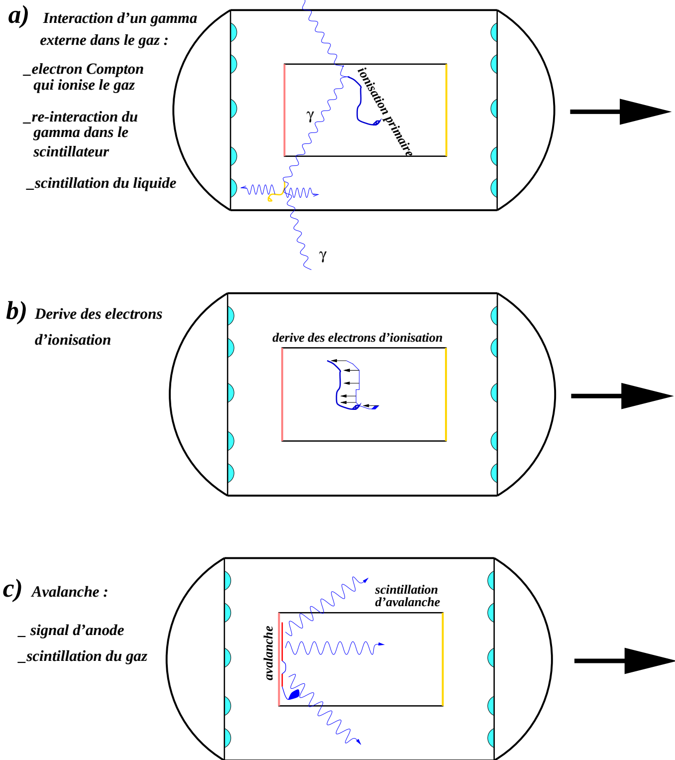
FIG. 4.21 – Signal et caractérisation d'un électron issu d'une diffusion Compton par un gamma externe
