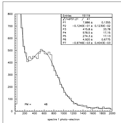
FIG. 3.14 – Spectre fortuit typique d'un PM
