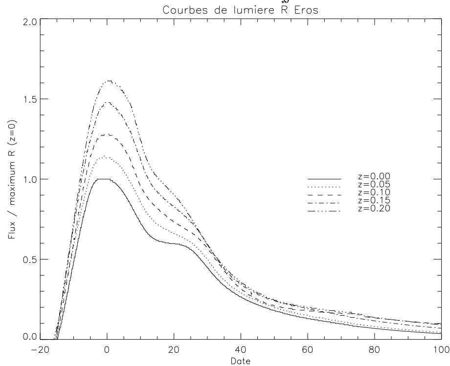
FIG. 6.12 – Courbes de lumière en R_{\text{EROS}} de supernovæ à différents redshifts : Les courbes de lumière sont exprimées en nombre de photons et sont normalisées par rapport au nombre de photons reçu en R_{\text{EROS}} pour une supernova à z = 0 . La normalisation relative des courbes traduit donc l'effet de la correction K .
