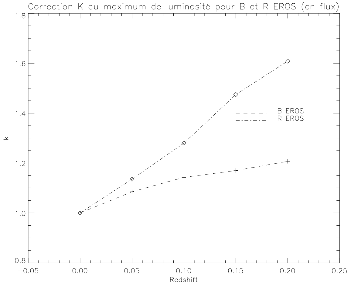
FIG. 6.15 – Corrections K en flux pour B_{\text{EROS}} et R_{\text{EROS}} en fonction de z pour une supernova au maximum de luminosité: La correction K est très faible pour le filtre B_{\text{EROS}} .
