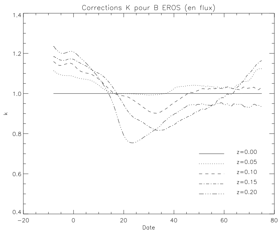
FIG. 6.13 – Corrections K en flux de photons pour B_{\text{EROS}} en fonction de l'âge de la supernova :
