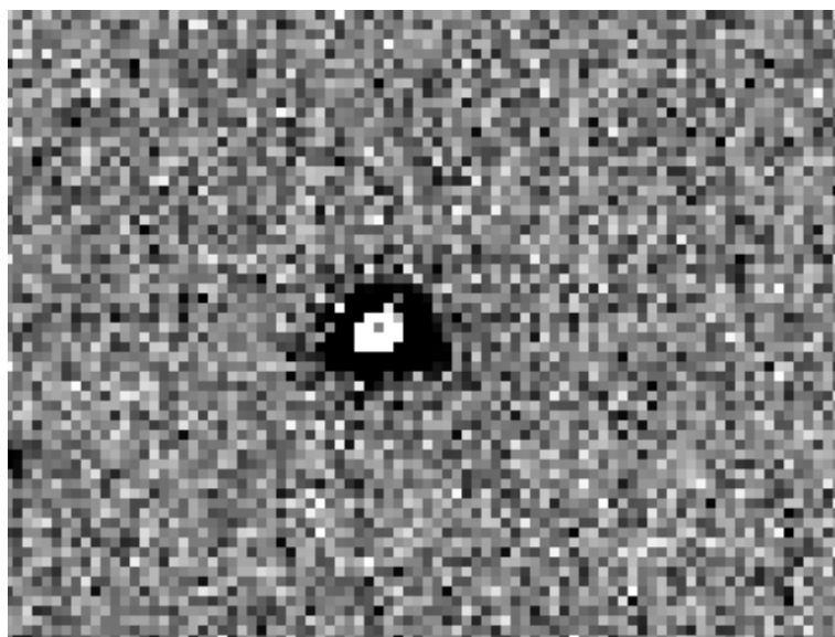
FIG. 4.4 – Mauvaise soustraction
