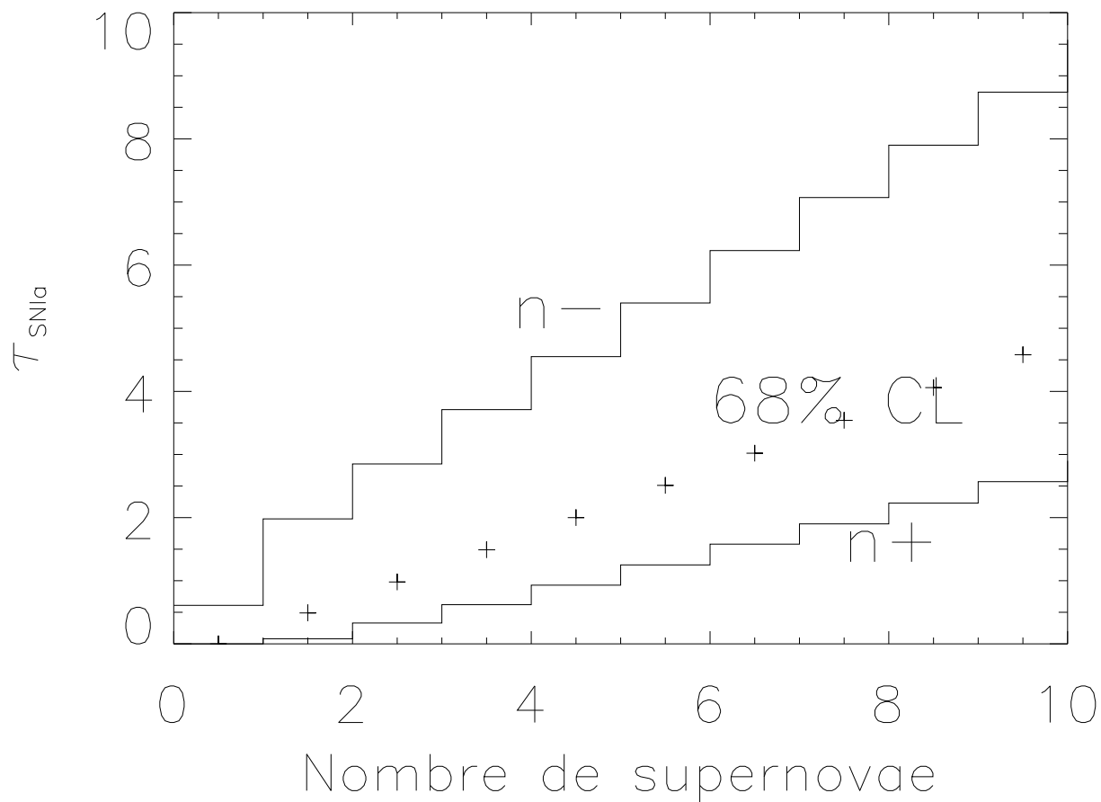
FIG. 7.17 – Région à 68% de niveau de confiance dans le plan (n, \tau) définie par la ceinture de Poisson :
