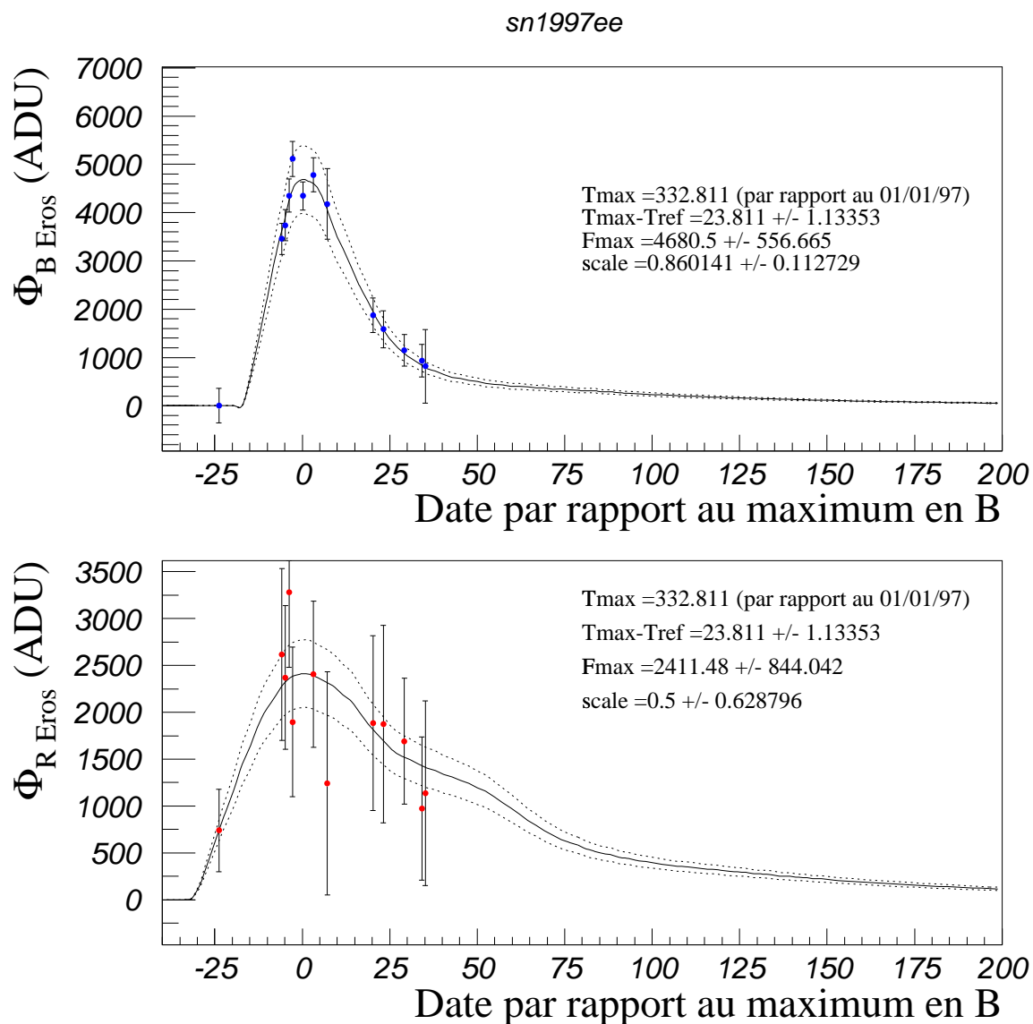
FIG. 6.23 – Courbe de lumière de SN1997ee: Le flux est très bas en R_{EROS} , l'ajustement est donc très peu contraint par cette couleur. Les courbes en pointillés indiquent l'incertitude ( 1\sigma ) sur le patron utilisé.
