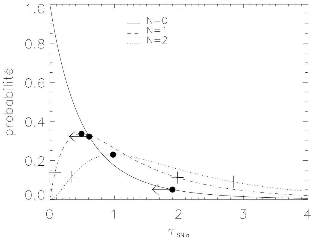
FIG. 7.18 – Distribution de probabilité du nombre observé de supernovæ de type Ia à N donné en fonction de \tau : en trait plein dans le cas où aucun de nos candidats n'est une SNIa; en tirets dans le cas où l'un des deux candidats est une SNIa et en pointillés si les deux candidats sont des SNIa. Les cercles noirs indiquent les valeurs obtenues (limite supérieure pour N = 0 , valeur la plus probable pour N = 1 et N = 2 ). Les croix indiquent les limites des intervalles de confiance à 68% pour N = 1 et N = 2 calculées par la méthode de la ceinture de Poisson.
