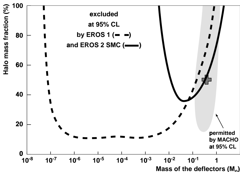
FIG. 3.5 – Contours d'exclusion pour les masses des objets compacts du halo de notre Galaxie : en pointillés les résultats d'EROS1 sur le Grand Nuage de Magellan [Renault et al., 1997], en traits pleins ceux d'EROS2 sur le Petit Nuage de Magellan (2 ans d'analyse) [Afonso et al., 1998] et en grisé les résultats de MACHO [Alcock et al., 1997] donnant une zone permise.
