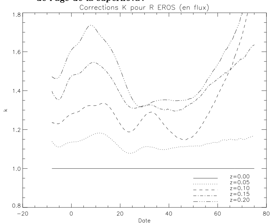
FIG. 6.14 – Corrections K en flux de photons pour R_{\text{EROS}} en fonction de l'âge de la supernova :
