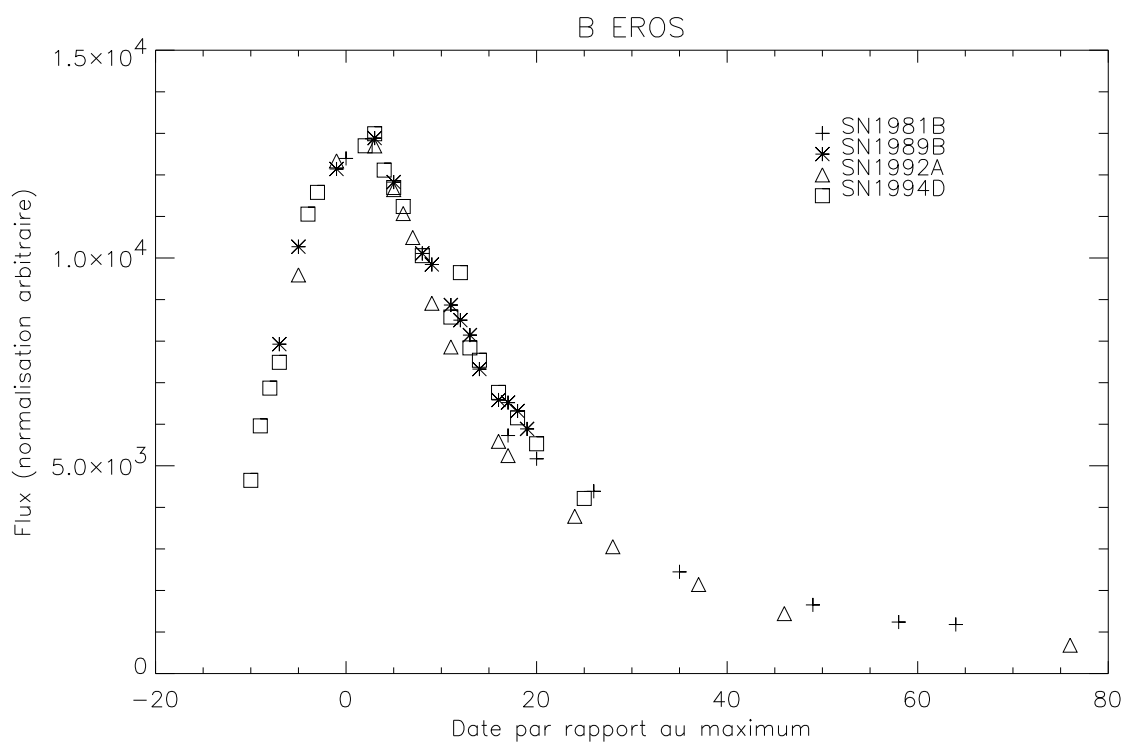
FIG. 6.7 – Courbe B_{\text{EROS}} obtenue pour les 4 supernovæ utilisées
