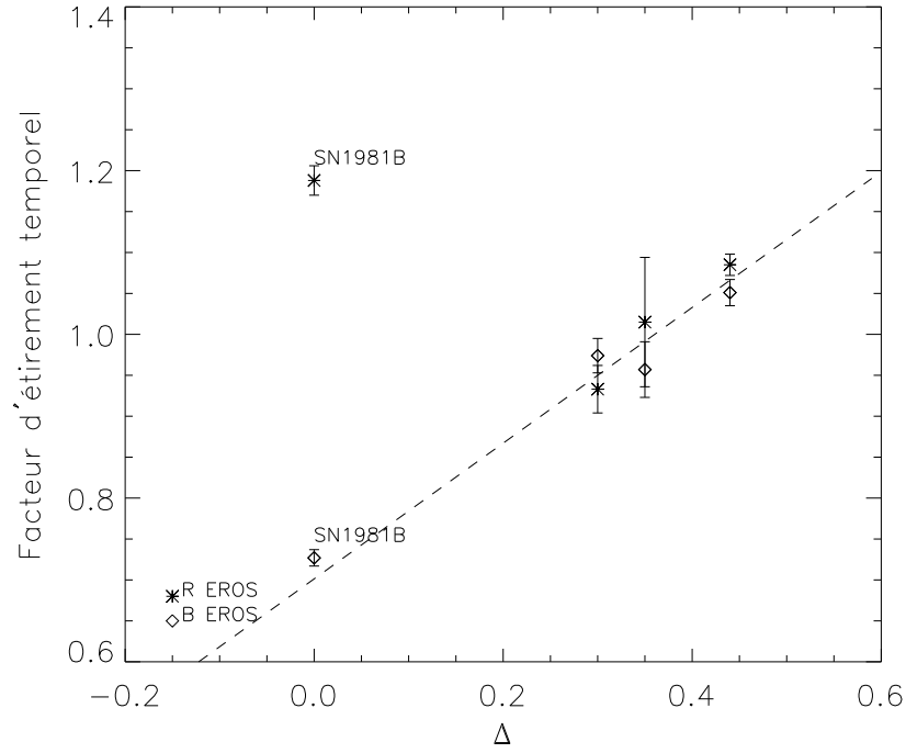
FIG. 6.17 – Comparaison entre le facteur d'étirement temporel obtenu en ajustant les courbes de lumière des 4 supernovæ en B_{\text{EROS}} et R_{\text{EROS}} et le paramètre \Delta déterminé par [Riess et al., 1996] : Les étoiles correspondent au facteur d'étirement en R_{\text{EROS}} et les croix à celui déterminé en B_{\text{EROS}} . Si l'on rejette les points concernant SN1981B pour laquelle on a trop peu de mesures pour déterminer efficacement le facteur d'étirement (les deux points sur la gauche), les points s'alignent sur une droite que l'on a superposé en tirets sur la figure.
