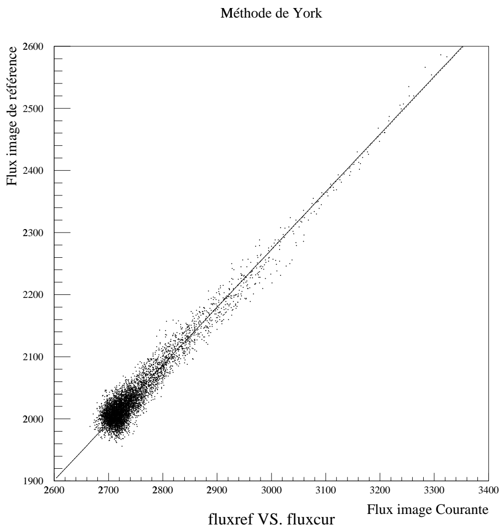
FIG. 5.12 – Sur ce graphe, le flux des pixels de l'image de référence est représenté en fonction de leur flux sur l'image courante (simulation). On a représenté la relation linéaire obtenue avec la méthode de York en traits pleins et la véritable relation linéaire en pointillés. Les deux courbes sont pratiquement confondues.
