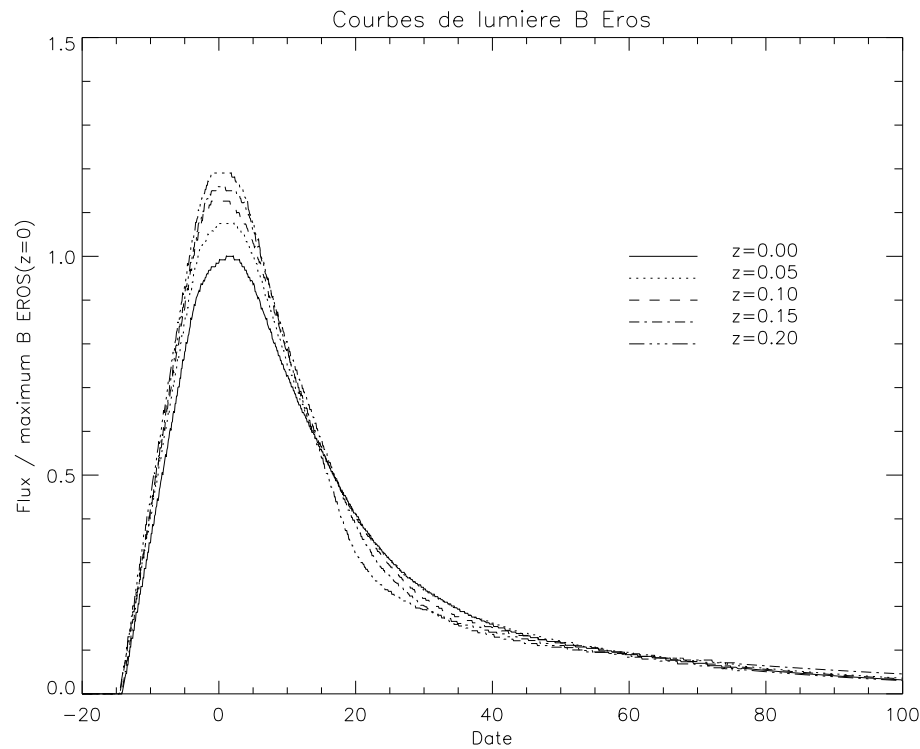
FIG. 6.11 – Courbes de lumière en B_{\text{EROS}} de supernovæ à différents redshifts : Les courbes de lumière sont exprimées en nombre de photons et sont normalisées par rapport au nombre de photons reçu en B_{\text{EROS}} pour une supernova à z = 0 . La normalisation relative des courbes traduit donc l'effet de la correction K .
