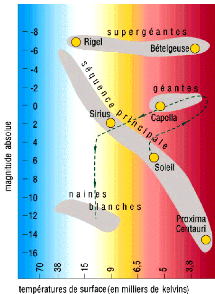
FIG. 2.1 – Diagramme de Hertzsprung-Russel : On représente la magnitude absolue des étoiles en fonction de leur température (donnée par la couleur). La bande diagonale est appelée la Séquence Principale, c'est dans cette bande que les étoiles passent la plus grande partie de leur vie. Les autres zones sont occupées par des étoiles en fin de vie.
