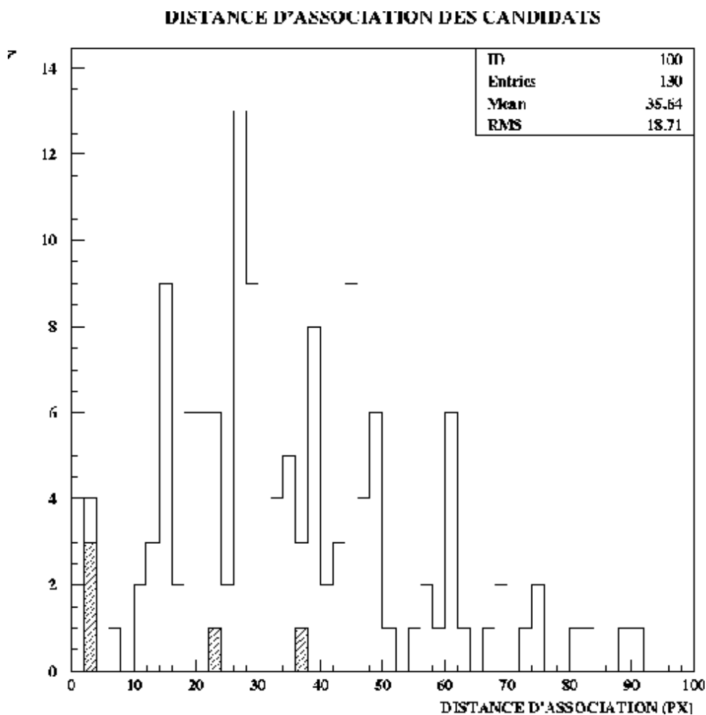
FIG. 4.7 – Distribution en distance des candidats avant rejet des cosmiques en blanc et après en hachuré. On voit bien que pratiquement toute la bosse à grande distance d'association à disparu. Le graphe est tracé ici pour un seul champ pour lequel le nombre de candidats est passé de 130 à 5.
