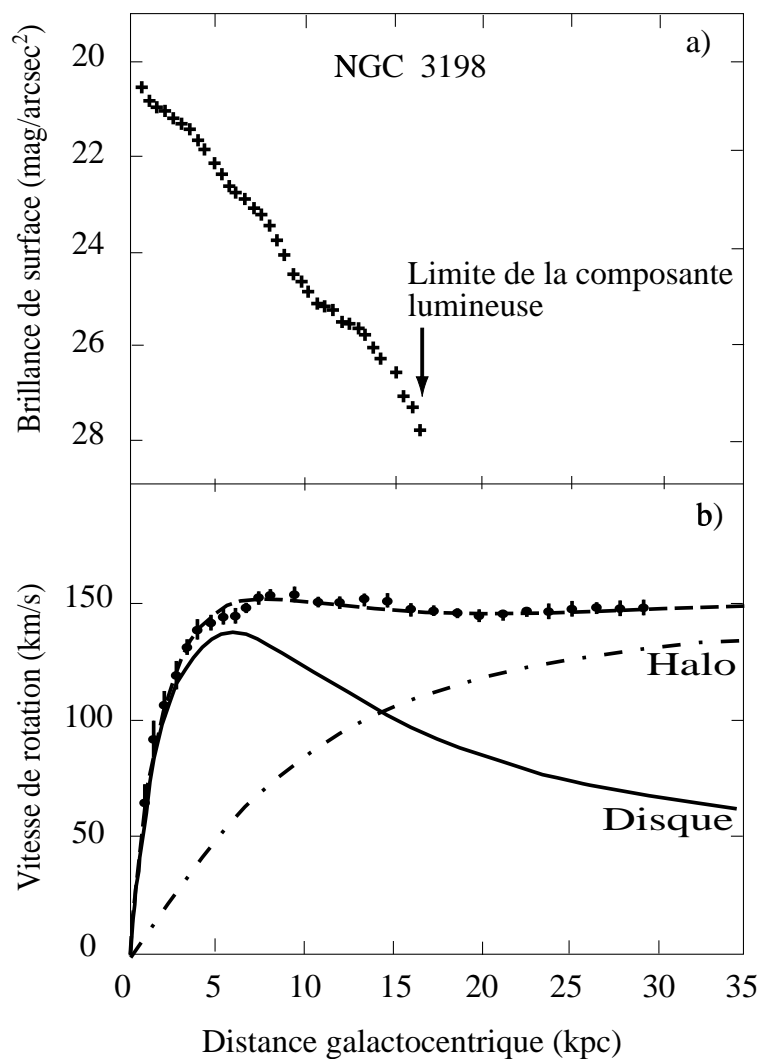
FIG. 3.1 – En haut : profil de luminosité de la galaxie NGC3198, on voit bien que la quantité de matière lumineuse décroît avec la distance au centre.
