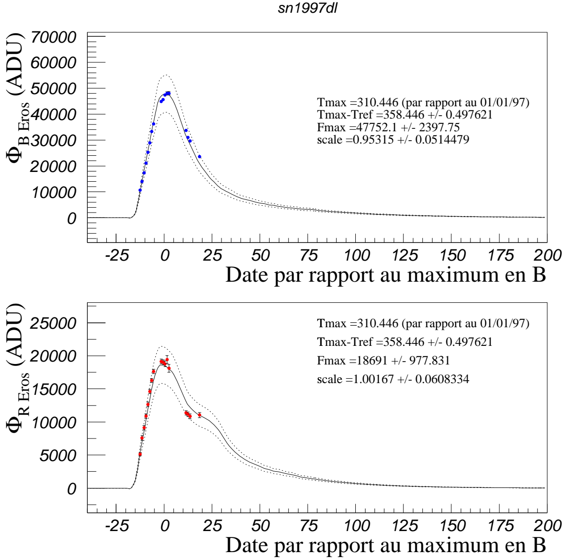
FIG. 6.22 – Courbe de lumière de SN1997dl: On remarque que l'ajustement n'est pas très bon en R_{\text{EROS}} , cependant, nous disposons de suffisamment de points au moment du maximum de luminosité pour que celui-ci soit bien contraint. Les courbes en pointillés indiquent l'incertitude ( 1\sigma ) sur le patron utilisé.
