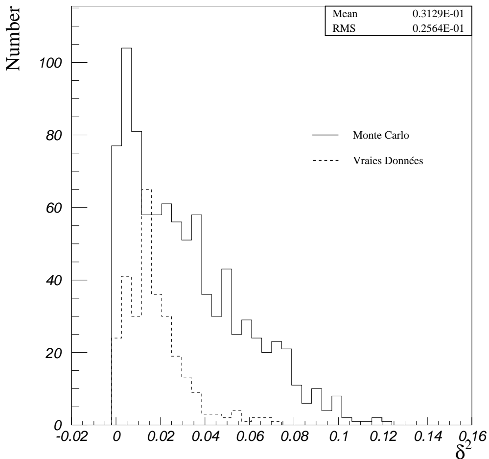
FIG. 5.4 – Valeur de \delta^2 utilisée lors de la convolution (en \text{pixel}^2 ): La différence entre la simulation et les données réelles provient de ce que la simulation ne reproduit pas les distributions des paramètres de forme sur les images réelles. La simulation est pessimiste par rapport à la réalité.
