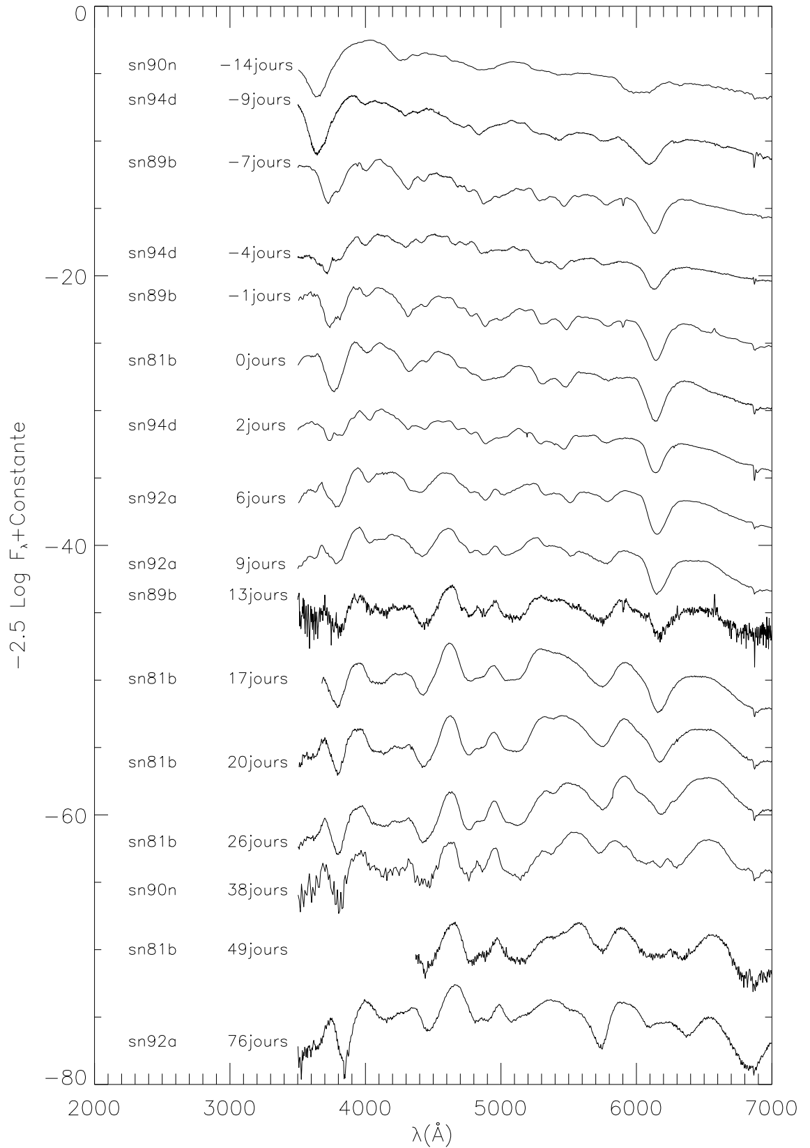
FIG. 2.7 – Spectres de supernovæ de type Ia à différentes dates par rapport au maximum : On remarque l'évolution temporelle du spectre, des raies en absorption se creusent d'abord pour finir par disparaître et des raies en émission apparaissent quelque temps après le maximum.
