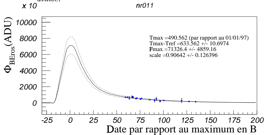
FIG. 6.20 – Courbe de lumière de nr011 : On n'a de point qu'en B_{\text{EROS}} , l'ajustement n'a donc été fait que sur cette couleur. Les courbes en pointillés indiquent l'incertitude ( 1 \sigma ) sur le patron utilisé.
