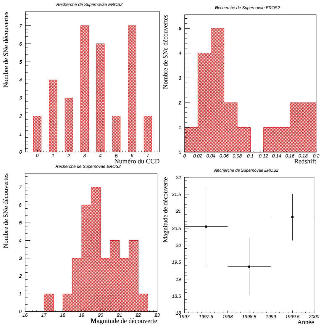
FIG. 3.11 – Résultats des campagnes de recherche de supernovæ d'EROS2 :
