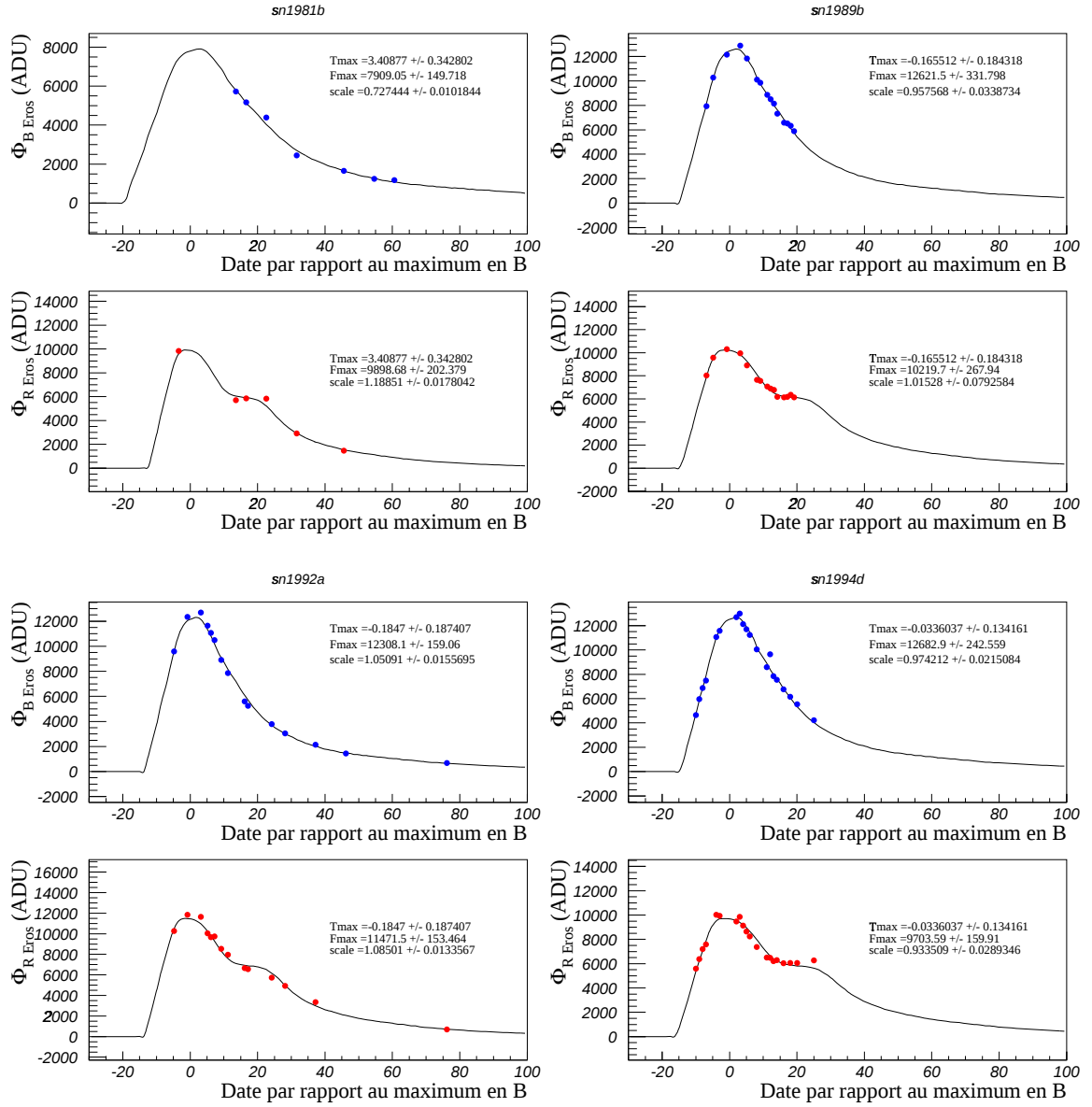
FIG. 6.16 – Ajustement en B_{\text{EROS}} et R_{\text{EROS}} des supernovæ utilisées pour fabriquer les patrons de courbes de lumière : les points de mesures ont été fabriqués à partir des spectres normalisés les uns par rapport aux autres par les courbes de lumière données par [Riess et al., 1996]. Notons que les ajustements sont bons excepté pour SN1981B pour laquelle on ne dispose pas de suffisamment de points de mesure pour que la courbe de lumière soit bien contrainte.
