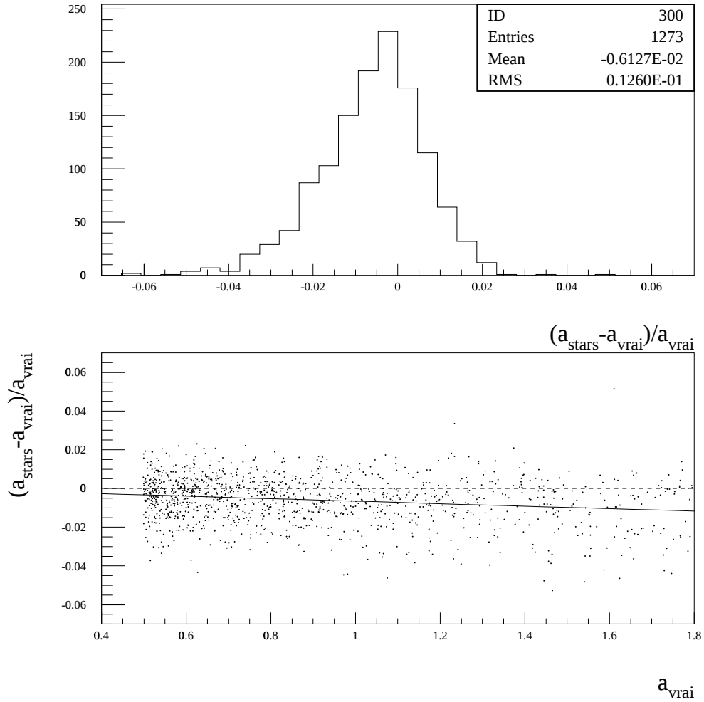
FIG. 5.10 – Résultats de la méthode des étoiles sur une simulation. On a représenté en haut l'histogramme de l'écart à la valeur véritable du coefficient photométrique (a_{stars} - a_{vrai})/a_{vrai} . Le graphe du dessous représente ce même écart en fonction de la valeur du coefficient photométrique.
