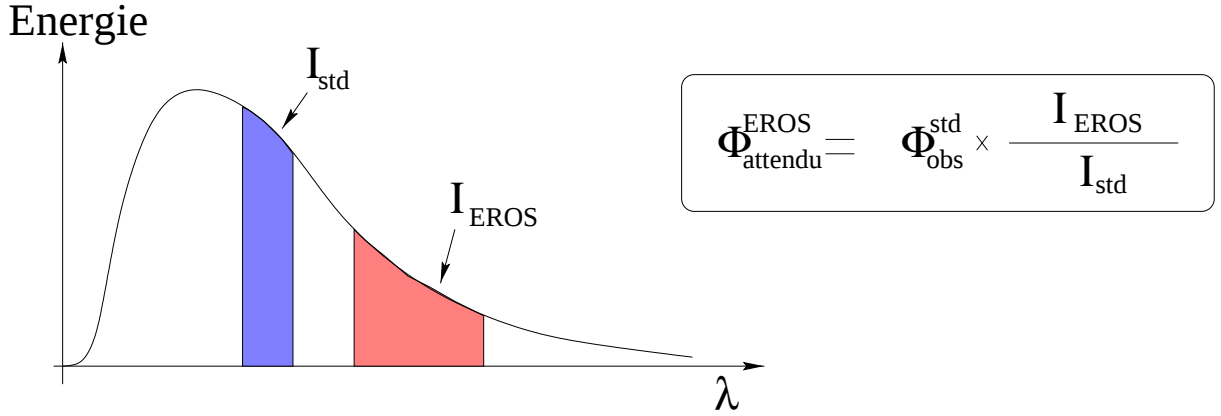
FIG. 6.1 – Calcul de transformations de couleur pour les courbes de lumière : On fabrique des observations synthétiques dans les bandes d'EROS2 à partir des observations dans les autres bandes et des spectres des supernovæ. Le flux attendu dans la bande d'EROS \phi_{\text{attendu}}^{\text{EROS}} est à un facteur de normalisation près l'intégrale sur notre bande passante I_{\text{EROS}} du spectre la supernova. La normalisation est donnée par le rapport entre le flux réellement observé dans une bande standard \phi_{\text{obs}}^{\text{std}} et l'intégrale du spectre sur la bande passante du filtre standard I_{\text{std}} .
