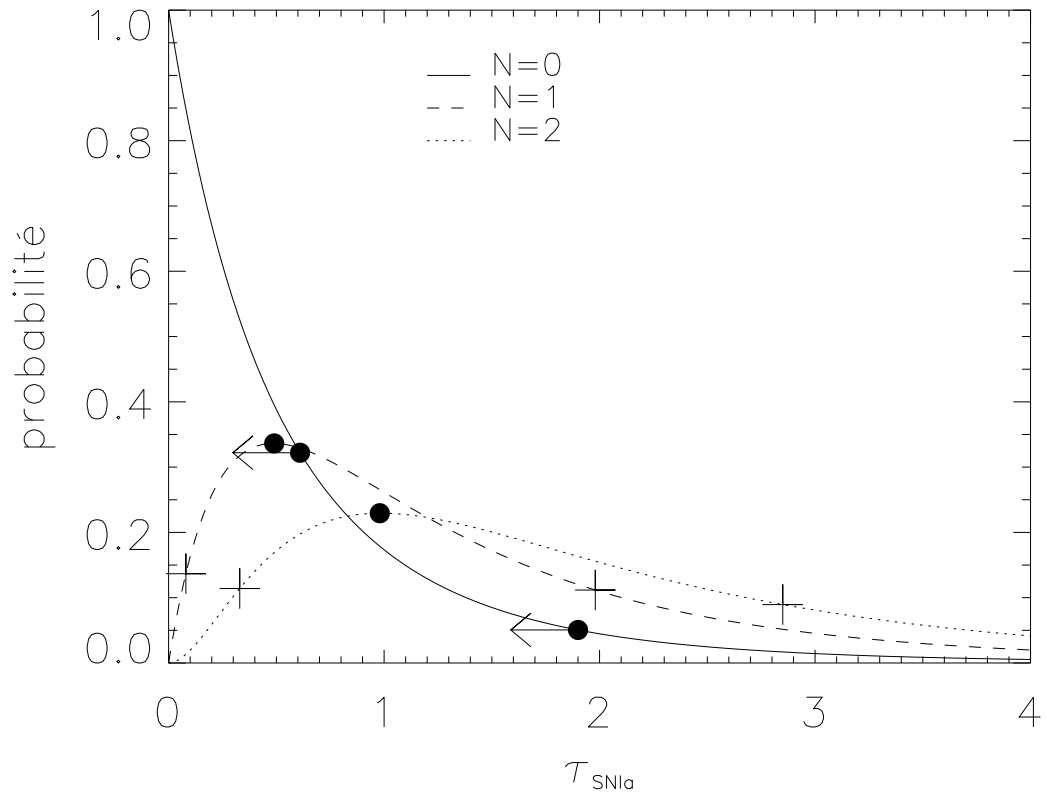
FIG. 7.18 – Distribution de probabilité du nombre observé de supernovæ de type Ia à N donné en fonction de \tau :
