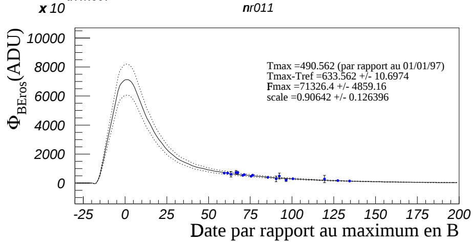
FIG. 6.20 – Courbe de lumière de nr011 : On n'a de point qu'en B_{\text{EROS}} , l'ajustement n'a donc été fait que sur cette couleur. Les courbes en pointillés indiquent l'incertitude ( 1\sigma ) sur le patron utilisé.
