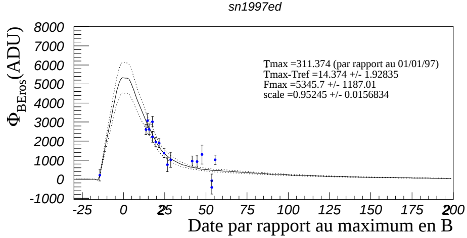
FIG. 6.19 – Courbe de lumière de SN1997ed : On n'a de point qu'en B_{\text{EROS}} , l'ajustement n'a donc été fait que sur cette couleur. Les courbes en pointillés indiquent l'incertitude ( 1\sigma ) sur le patron utilisé.
