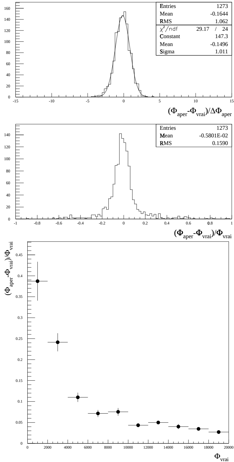
FIG. 5.20 – Résultats de la photométrie d'ouverture. en haut: histogramme de l'écart à la valeur véritable du flux ajusté en nombre d'écart-type sur la simulation.
