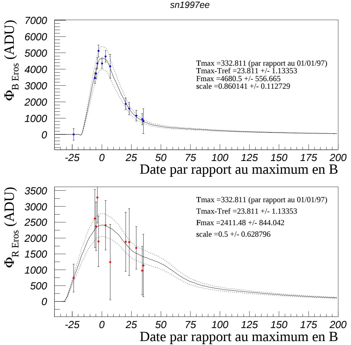
FIG. 6.23 – Courbe de lumière de SN1997ee: Le flux est très bas en R_{\text{EROS}} , l'ajustement est donc très peu contraint par cette couleur. Les courbes en pointillés indiquent l'incertitude ( 1\sigma ) sur le patron utilisé.
