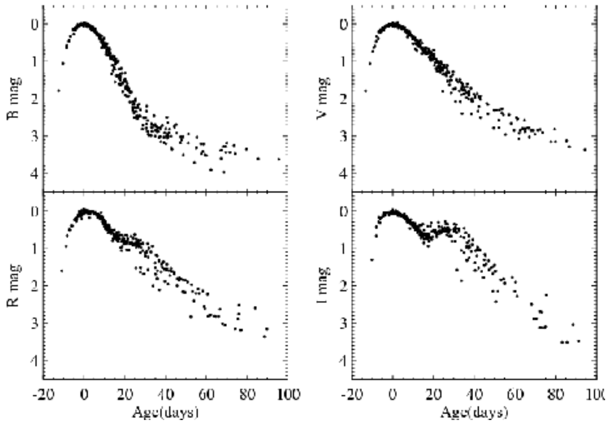
FIG. 2.8 – Superposition des courbes de lumière de 22 supernovæ de type Ia en 4 couleurs :
