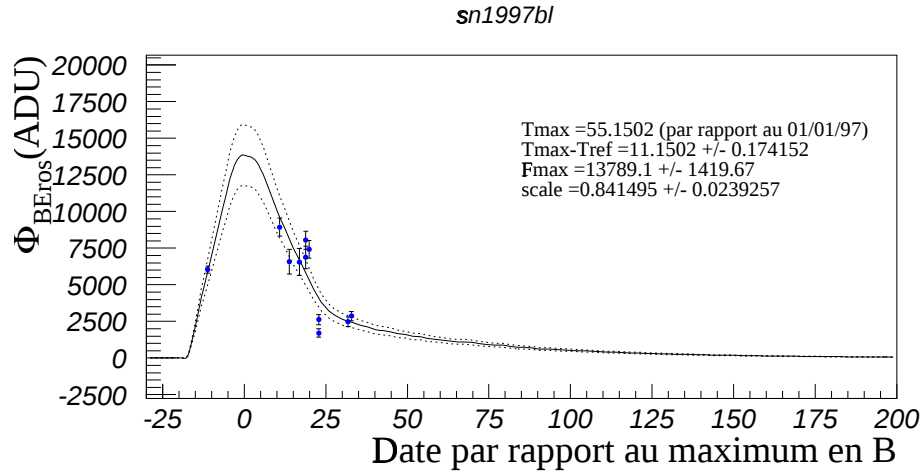
FIG. 6.18 – Courbe de lumière de SN1997bl : On n'a de point qu'en B_{\text{EROS}} , l'ajustement n'a donc été fait que sur cette couleur. Les courbes en pointillés indiquent l'incertitude ( 1\sigma ) sur le patron utilisé.
