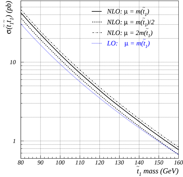
FIG. 2.3 – Section efficace totale de production p\bar{p} \rightarrow \tilde{t}_1\bar{\tilde{t}}_1 en fonction de la masse m_{\tilde{t}_1} dans l'approximation de Born (LO) et au NLO et ceci pour trois choix de l'échelle \mu .
