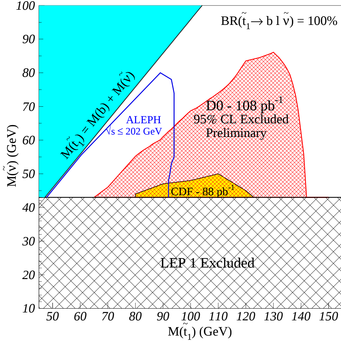
FIG. 7.19 – Régions MSSM exclues dans le plan (m_{\tilde{t}_1}, m_{\tilde{\nu}}) . Les résultats de notre analyse (marqués DØ 108 pb -1 ) sont comparés aux contours d'exclusion obtenus par les expériences ALEPH, CDF et LEP 1 également obtenus dans le canal de désintégration \tilde{t}_1 \rightarrow b \ell \tilde{\nu} .
