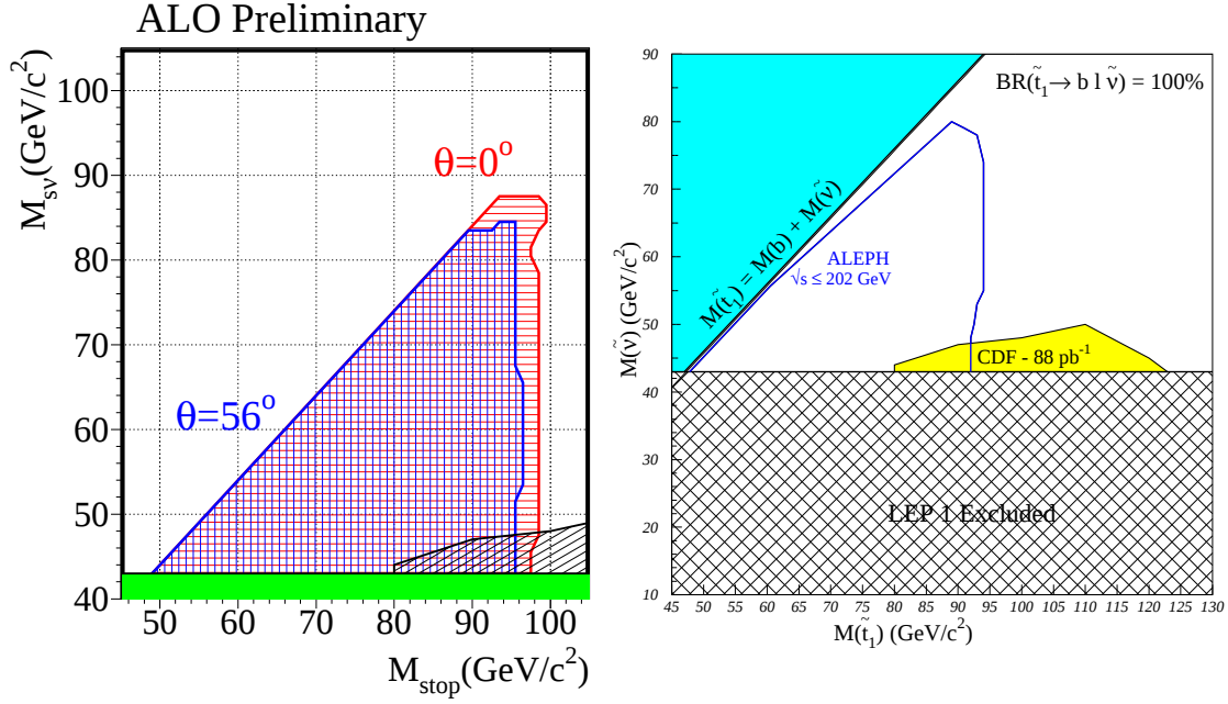
FIG. 2.14 – (a) Régions exclues à 95% de niveau de confiance dans le plan (m_{\tilde{t}_1}, m_{\tilde{\nu}}) par les expériences ALEPH, L3 et OPAL au LEP (résultats préliminaires à \sqrt{s} = 208 \text{ GeV} ) dans le cadre des recherches de désintégrations \tilde{t}_1 \rightarrow b l \tilde{\nu} . (b) Région exclue par l'expérience CDF, comparée aux résultats publiés d'ALEPH à \sqrt{s} = 202 \text{ GeV} et \theta_{\tilde{t}_1} = 0^\circ .
