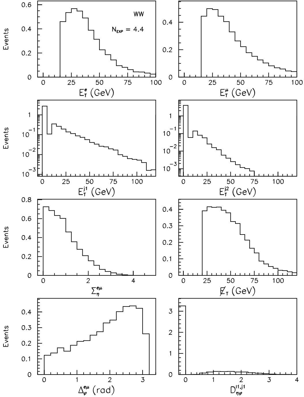
FIG. 7.8 – Distributions après sélection du bruit de fond WW \rightarrow e\mu E_T de l'énergie transverse a) des électrons; b) des muons; c) (d) du (second) jet le plus énergétique; e) valeur absolue de la somme des pseudorapidités des deux leptons; f) énergie transverse manquante; g) différence d'angle azimuthal entre les deux leptons; h) plus petite distance entre le jet le plus énergétique et chacun des leptons pour une luminosité de 108.3 \text{ pb}^{-1} .
