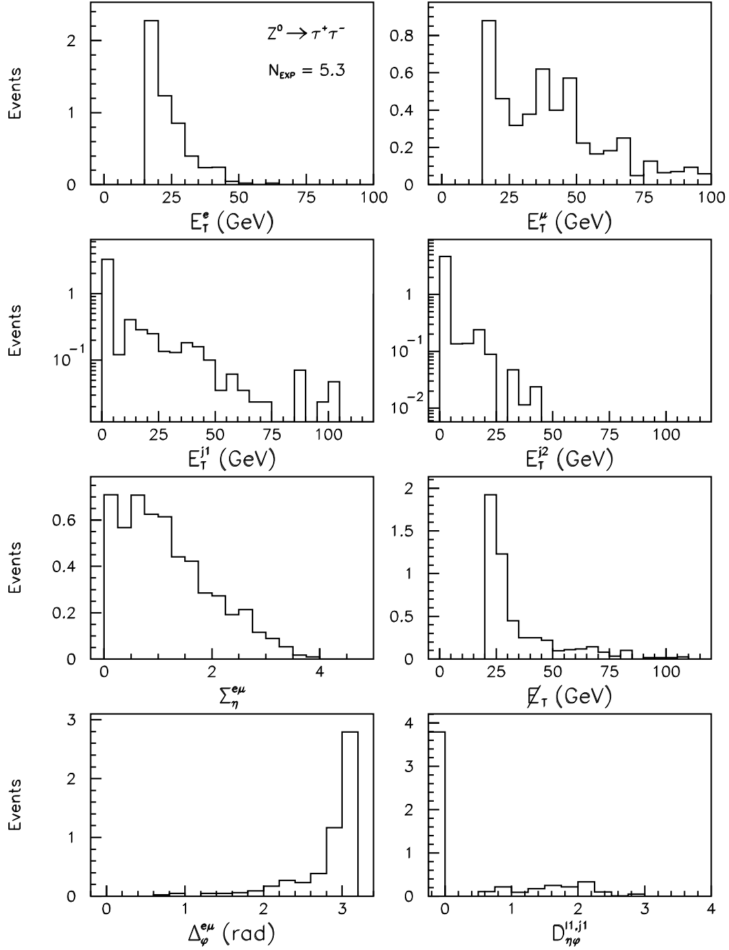
FIG. 7.7 – Distributions après sélection du bruit de fond Z^0 \rightarrow \tau^+ \tau^- \rightarrow e\mu \cancel{E}_T de l'énergie transverse a) des électrons; b) des muons; c) (d) du (second) jet le plus énergétique; e) valeur absolue de la somme des pseudorapidités des deux leptons; f) énergie transverse manquante; g) différence d'angle azimuthal entre les deux leptons; h) plus petite distance entre le jet le plus énergétique et chacun des leptons pour une luminosité de 108.3 \text{ pb}^{-1} .
