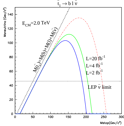
FIG. 8.3 – Limites attendues au Run II pour le canal \tilde{t}_1 \rightarrow b l \tilde{\nu} et pour différentes luminosités intégrées. Les rapports d'embranchement du sTop en bl\tilde{\nu}_l sont supposés de 33.3% ( l = e, \mu, \tau ).
