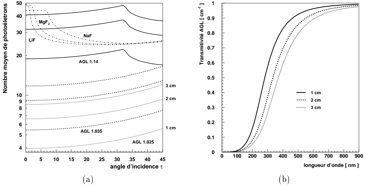
FIG. 3.12: (a) Nombre moyen de photoélectrons produits pour différents radiateurs. Les radiateurs en NaF , LiF et MgF_2 ont 1 cm d'épaisseur; les courbes pour les AGL sont proposées pour trois épaisseur : 1, 2 et 3 cm. (b) Transmittivité Rayleigh intégrée sur l'épaisseur d de l'AGL exprimé par unité d'épaisseur en fonction de la longueur d'onde \lambda . Les 3 courbes correspondent à des radiateurs de 1, 2 et 3 cm d'épaisseur.
