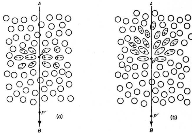
FIG. 3.2: Polarisation induite par le passage d'une particule chargée : (a) à basse vitesse (b) à grande vitesse, d'après Jelley [32]
