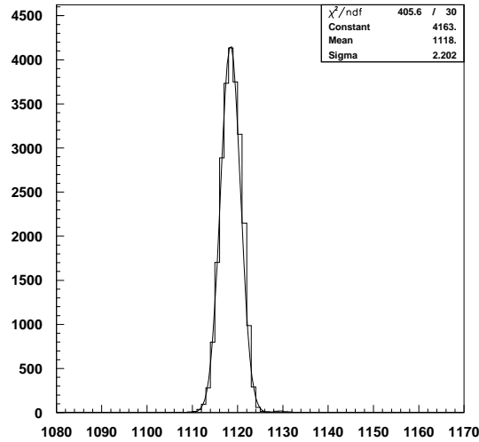
FIG. 4.17: Résolution électronique de la chaîne de mesure du temps de vol, donnée par le signal en temps de S3, déclenché par le Trigger expérimental, qui est son image. La gamme de codage est de 25 ps par canal.
