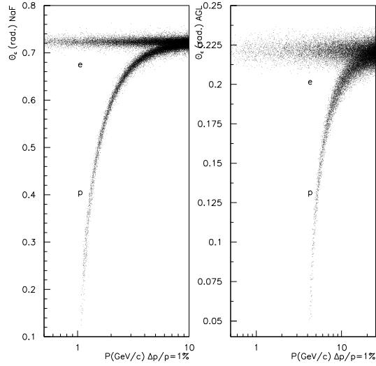
FIG. 2.13: Séparation hadron/lepton étudié avec la simulation. Gauche : résultat pour le NaF. Droite : résultat pour l'AGL d'indice 1.025. Voir texte.
