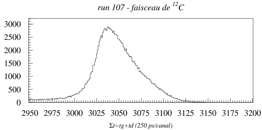
FIG. 4.26: Checksum des chambres I_1, I_2, I_3, I_4 (mélange Argon/Ethane+Freon). La largeur à mi-hauteur vaut \delta t_0 \sim 12ns . Sur ce run, la haute tension était inférieure à la tension nominale, ce qui explique la queue bas canal, associée à une mauvaise reconstruction de la position.
