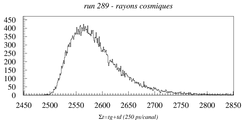
FIG. 4.28: Checksum des chambres C_1, C_2, C_3 (mélange Argon/Ethane/Freon). La largeur à mi-hauteur vaut \delta t_0 \sim 20ns
