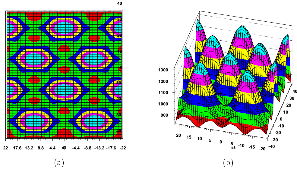
FIG. 7.4: Variation de la surface d'intersection des photocathodes du prototype (en \text{mm}^2 ) avec un anneau de diamètre interne r_c = 80 \text{ mm} et d'épaisseur 5 mm, en fonction de la position du centre de l'anneau sur la matrice (surface de l'anneau \approx 2590 ) (a) vue de dessus (b) vue en trois dimensions.
