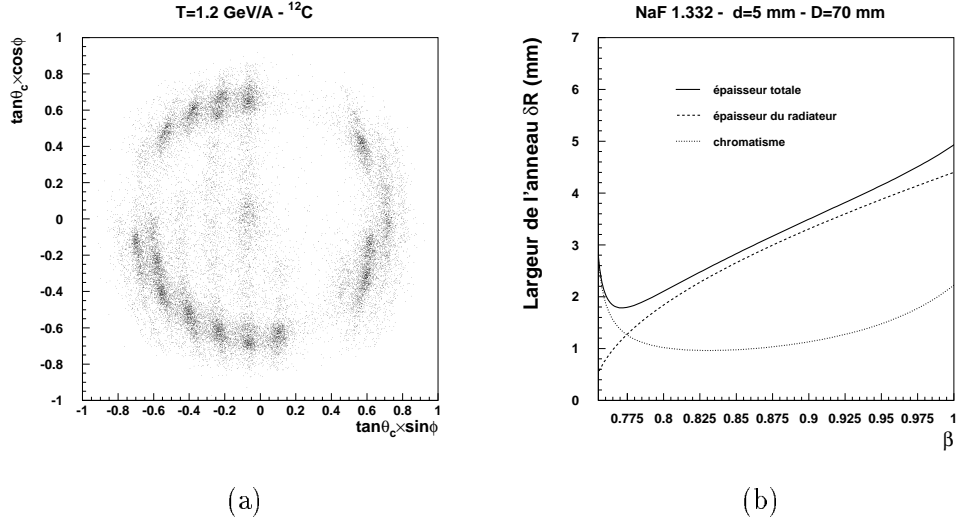
FIG. 7.6: (a) Image brute des anneaux dans le repère de la trajectoire pendant la dernière nuit de prise de données ( T \geq 1.2 \text{ GeV/A} ). On distingue clairement une zone morte importante correspondant à des PM sans haute tension. (b) Variation de l'épaisseur de l'anneau de lumière sur le prototype à incidence nulle en fonction de la vitesse \beta . La courbe tiretée correspond à la contribution de l'épaisseur du radiateur, la courbe pointillée correspond à la contribution du chromatisme du NaF.
