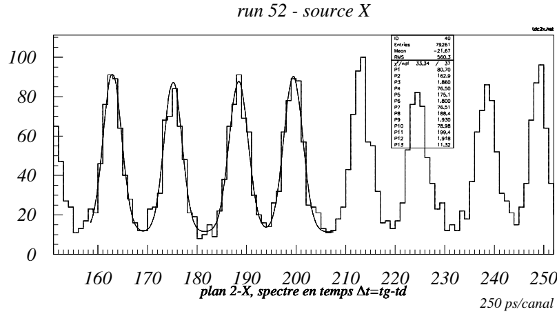
FIG. 4.22: Estimation de la résolution temporelle d'une chambre à fil du minirich sous éclairage X - un ajustement a été réalisé avec 4 gaussiennes et un bruit de fond blanc, qui permet d'améliorer la vraisemblance du fit ( \chi^2 \sim 0.8 ).
