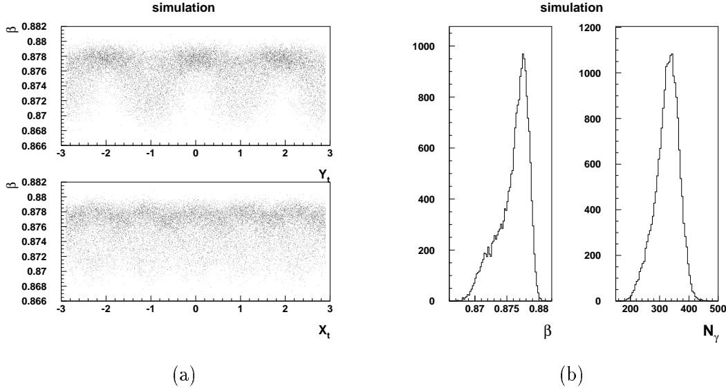
FIG. 7.7: Résultat de la simulation d'un RUN d'ions ^{12}\text{C} d'énergie T = 1 \text{ GeV/A} arrivant à petit angle ( < 0.1^\circ ). A gauche : variation de la mesure de \beta en fonction de la position du centre de l'anneau sur la matrice (X_t, Y_t) . A droite : distribution des vitesses mesurées et du nombre de photoélectrons. Voir texte.
