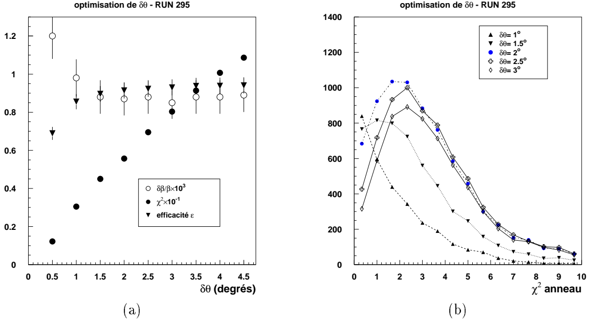
FIG. 5.9: Optimisation de la valeur \Delta\theta utilisée dans la méthode des "écarts" dans le cas d'un RUN cosmique avec un radiateur en NaF de 10 mm et un espace de glissement de 52 mm (RUN 295). (a) Evolution de \frac{\delta\beta}{\beta} (avec coupure sur le \chi^2 < 5 ), \langle\chi^2\rangle (ajustement de l'anneau) et \epsilon (taux de reconstruction) en fonction de \Delta\theta . (b) Variation de la vraisemblance de l'ajustement de l'anneau en fonction de \langle\chi^2\rangle .
