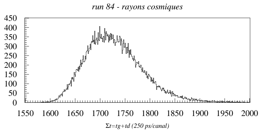
FIG. 4.27: Checksum des chambres C_1, C_2, C_3 (mélange Argon/Ethane). La largeur à mi-hauteur vaut \delta t_0 \sim 32ns
