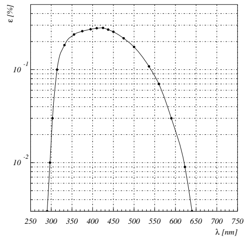
FIG. 4.4: Efficacité quantique de la photocathode du PM Philips XP2802 en fonction de la longueur d'onde \lambda . La courbe est extraite de la notice technique du constructeur.
