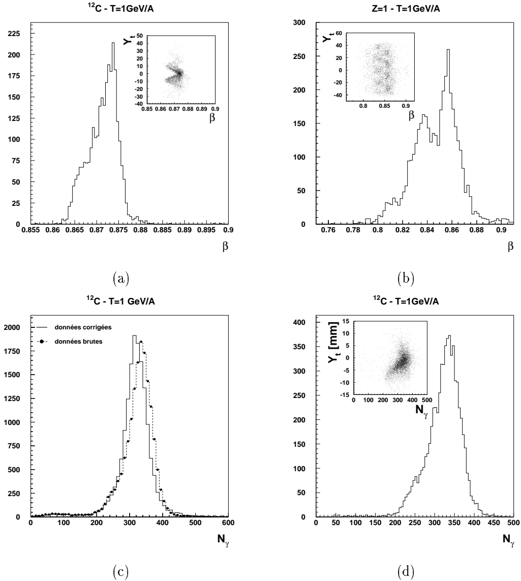
FIG. 7.3: Haut : mesure typique de vitesse \beta du prototype pour un faisceau de ^{12}\text{C} (a) et de Deutérium (b). Bas : (d) mesure du nombre de photoélectrons N_\gamma donné par des ions ^{12}\text{C} pendant le même RUN que la figure (a). (c) Correction de l'erreur systématique sur N_\gamma pour une incidence normale. Voir texte.
