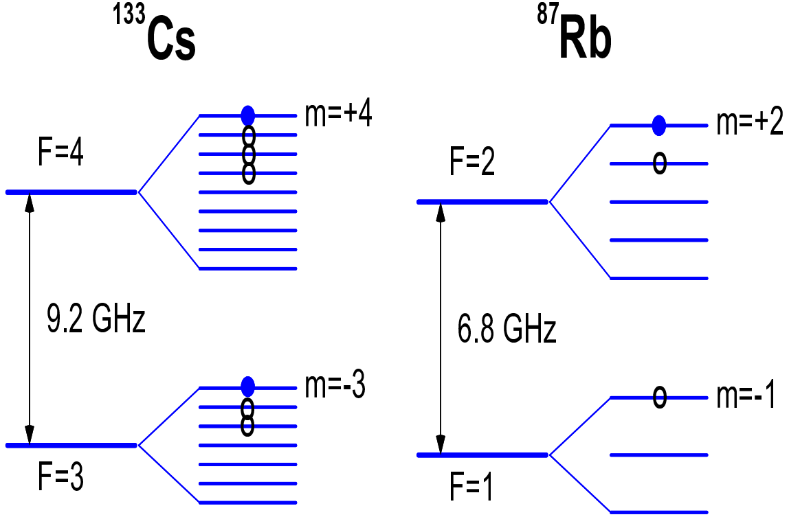
FIG. 1.3 – Représentation schématisée des niveaux Zeeman de la structure hyperfine du niveau fondamental S_{1/2} pour les atomes de ^{133}\text{Cs} et de ^{87}\text{Rb} . Les ● représentent les états utilisés pour les pièges magnétiques. Et les ○, les autres états piégeables par un minimum de module de champ magnétique.
