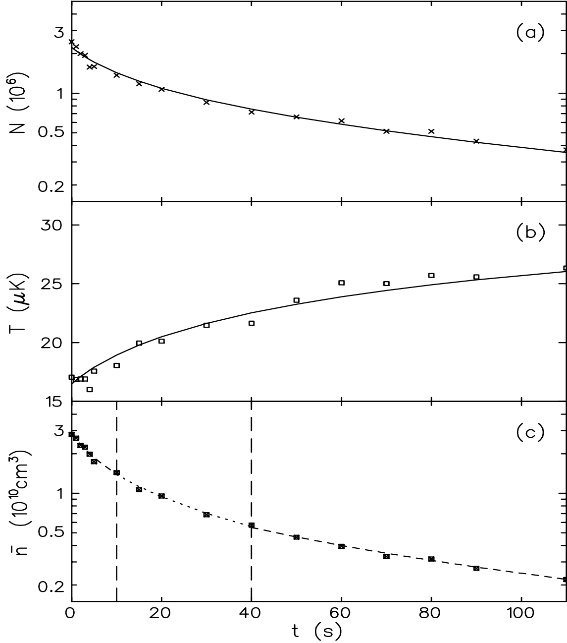
FIG. 4.4 – (a) Evolution clairement non exponentielle du nombre d'atomes dans le piège après un temps de relaxation t . (b) Variation de la température en fonction de t (c) densité atomique en fonction de t . Sur chaque intervalle de (c) la densité est ajustée par la loi (4.8) les courbes ainsi obtenues sont en pointillés. Les courbes en trait plein sur les figures (a) et (b) sont solutions des équations (4.5, 4.6) avec G \propto T^{-0.63} .
