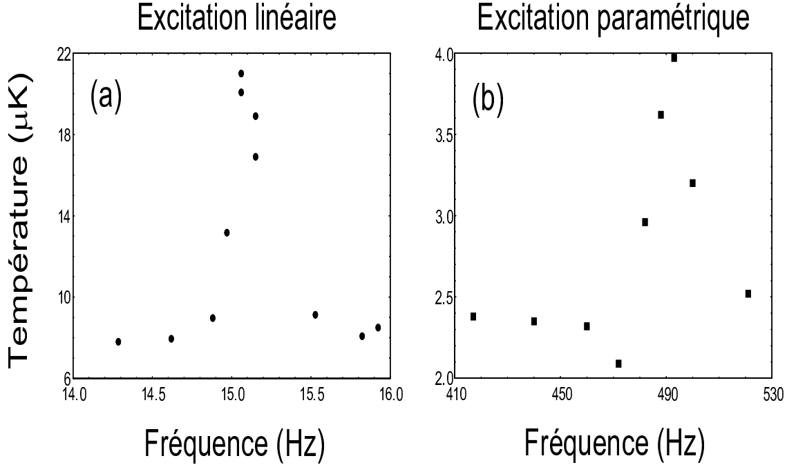
FIG. 6.4 – Evolution de la température lors du balayage de la fréquence d'excitation. (a) Excitation linéaire par déplacement du fond du puits de potentiel selon l'axe longitudinal. (b) Excitation paramétrique par modulation de la raideur transverse du piège.
