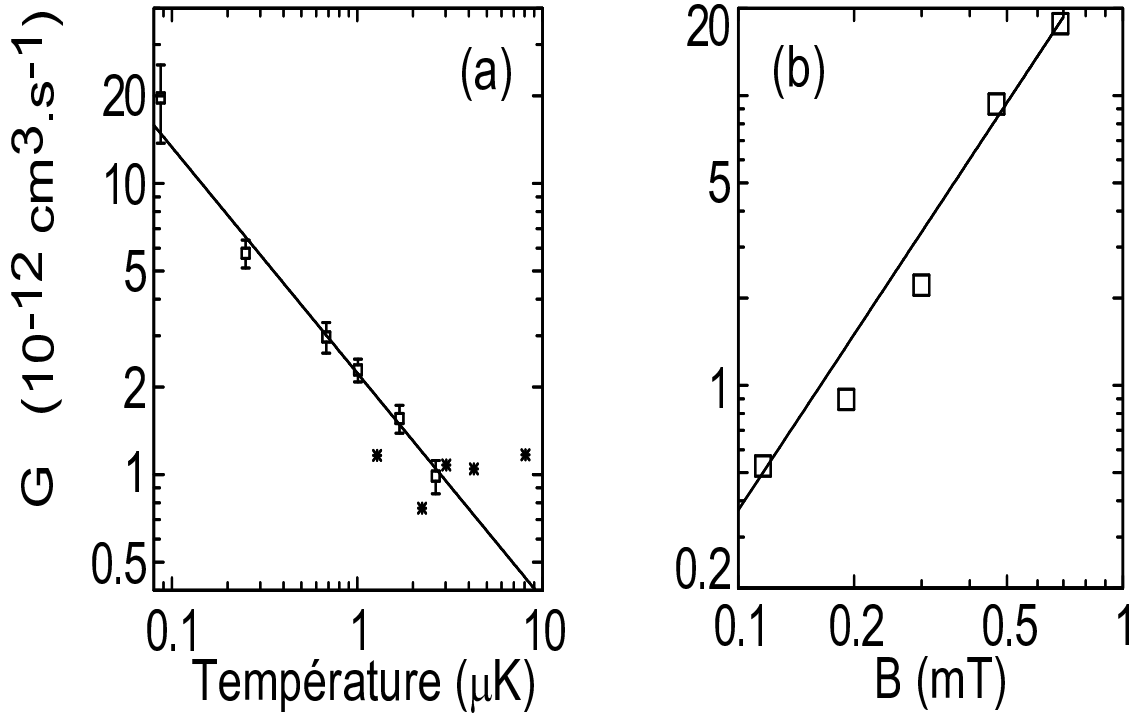
FIG. 5.10 – Variations du taux de pertes à deux corps G(B, T) avec (a) la température T pour une valeur fixe du champ B_0 = 3.02 \text{ Gauss} , (b) le champ magnétique B_0 pour une température fixe T = 1 \mu\text{K} . Dans (a) les carrés (étoiles) correspondent aux données d'expériences de relaxation obtenues en présence (en l'absence) d'un bouclier radiofréquence.
