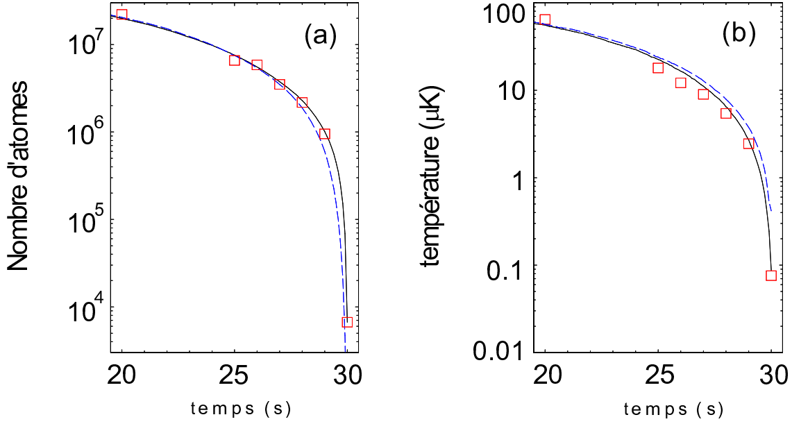
FIG. 5.5 – Evolution en (a) du nombre d’atomes et en (b) de la température pour les dix dernières secondes de la rampe d’évaporation. Les points expérimentaux sont représentés par les carrés, les lignes correspondent aux simulations numériques : la ligne continue correspond à |a| = 1000 \text{ \AA} , et la ligne en traits pointillés à |a| = 100 \text{ \AA} .
