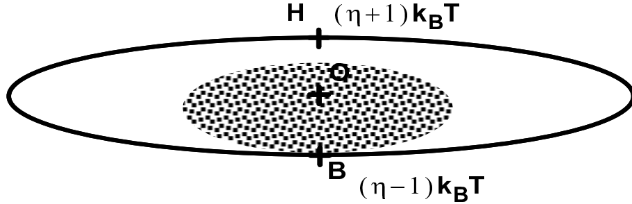
FIG. 5.3 – Modification de la dimensionnalité en présence de gravité pour un piège magnétique de type Ioffe-Pritchard.
