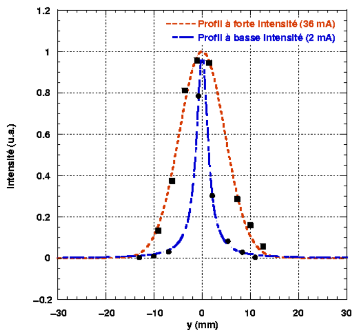
Fig. 5-17 : Profils verticaux à 230 keV
