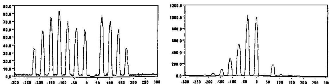
Fig. 5-13 : Profils horizontaux avec l'extraction non reprise (à g.) puis reprise (à d.)
