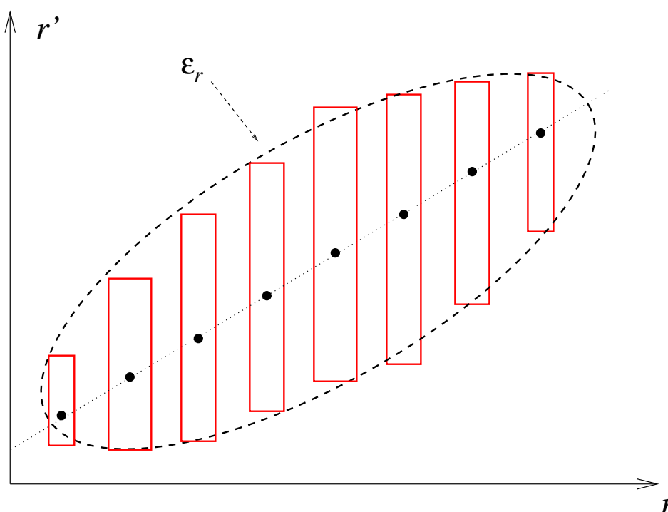
Fig. 5-11 : Émittance reconstituée à partir du faisceau passant par la poivrière.
