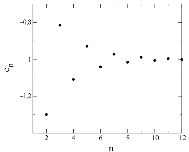
Fig. 2-6 : Coefficients c_n pour la "bibosse"
