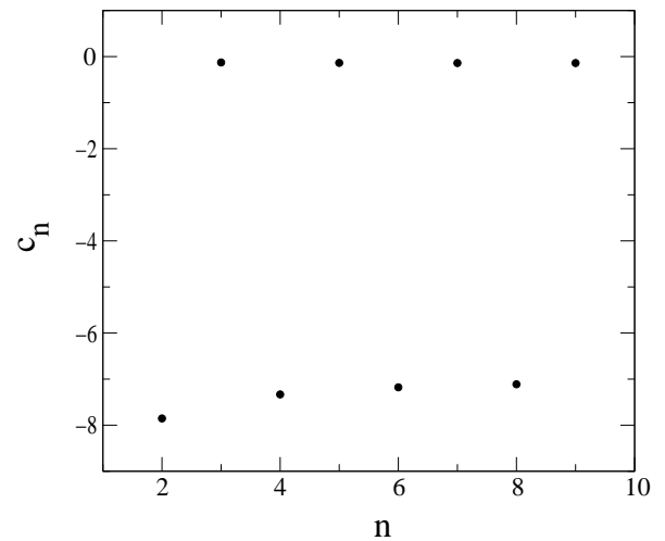
Fig. 2-12 : Coefficients c_n pour la bosse décalée par rapport à l'origine
