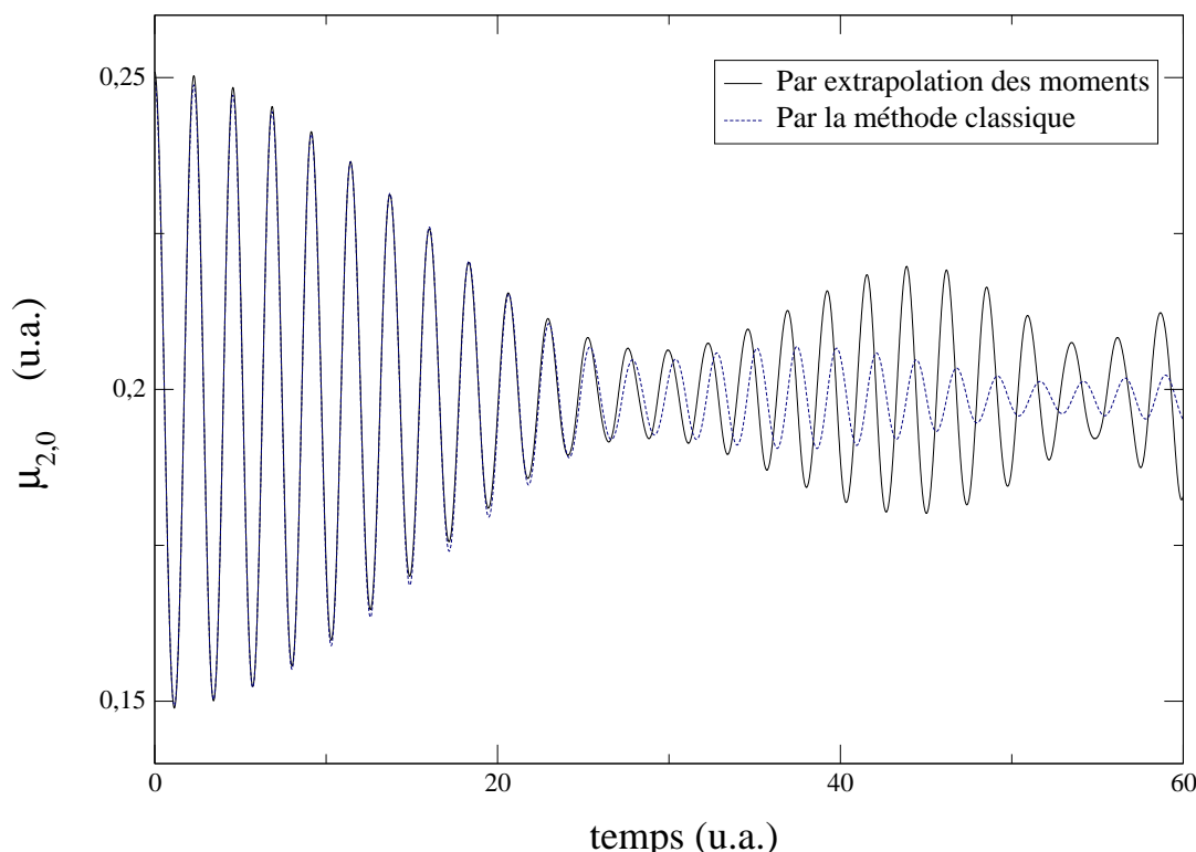
Fig. 4-16 : Moment \mu_{2,0} pour un nuage de 32000 particules de densité uniforme en fonction du temps
