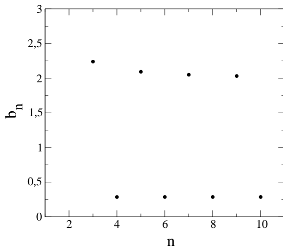
Fig. 2-11 : Coefficients b_n pour la bosse décalée par rapport à l'origine
