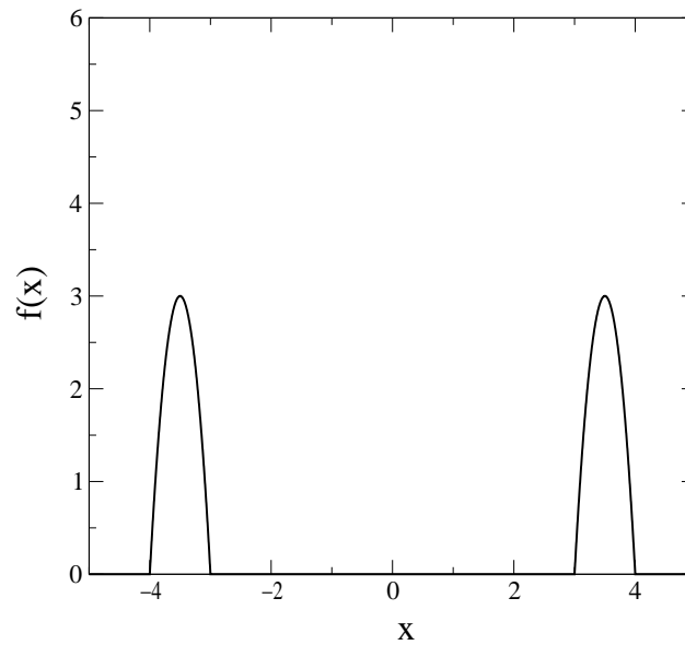
Fig. 2-10 : Densité bosse décalée par rapport à l'origine
