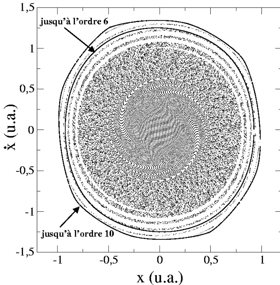
Fig. 4-13 : Enveloppe convexe en fonction du nombre de moments utilisés : jusqu'à l'ordre 6 ou 10 pour un nuage de 32000 particules à l'instant t=100 (u.a.) de densité initiale uniforme
