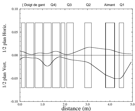
Fig. 5-18 : A 2 mA, réglages standards Mesure avec Q0 en sortie de tube
