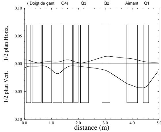
Fig. 5-22 : A 2 mA, réglages standards ; mesure avec Q0 en sortie de tube
