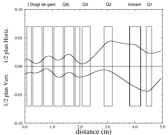
Fig. 5-24 : A 38 mA, réglages standards
