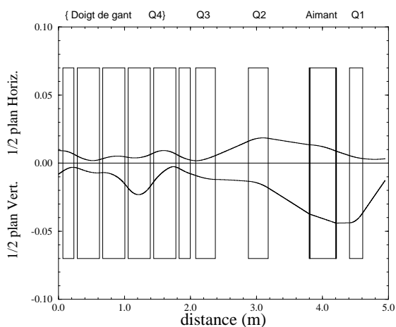
Fig. 5-20 : A 2 mA, réglages standards Mesure avec Q0 en sortie de tube
