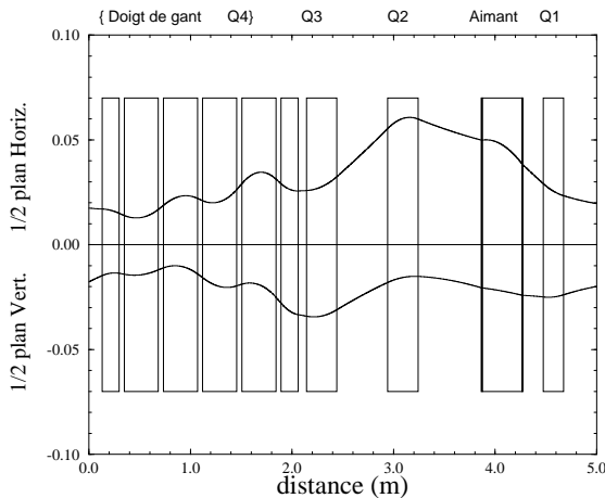
Fig. 5-23 : Réglages théoriques initiaux
