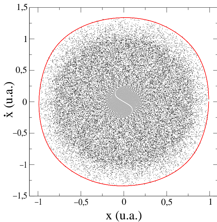
Fig. 4-8 : Comparaison entre le nuage de 32000 particules à l'instant t=2000 (u.a.) de densité initiale uniforme et l'enveloppe convexe calculée à partir de ses moments
