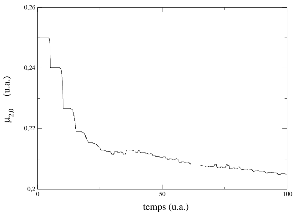
Fig. 3-14 : Evolution du moment \mu_{2,0} moyenné issue des 64 points en fonction du temps
