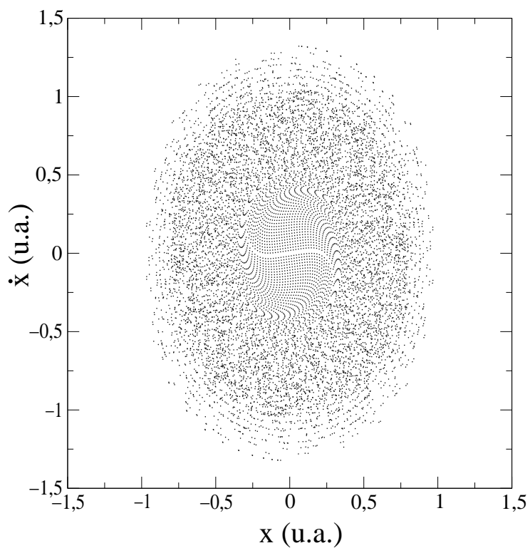
Fig. 3-5 : Distribution du nuage de points à t=200 dans l'espace des phases (x, \dot{x})
