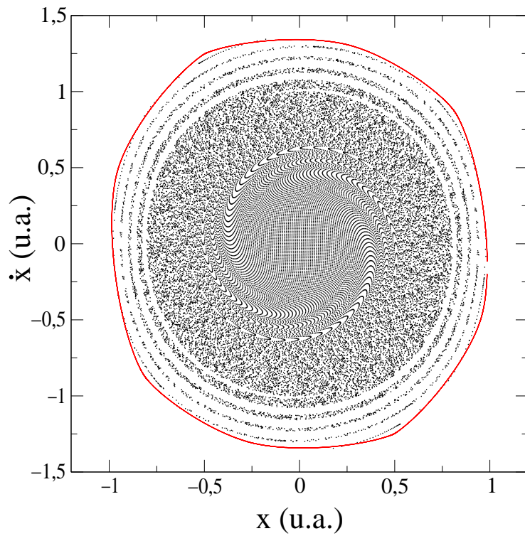
Fig. 4-7 : Comparaison entre le nuage de 32000 particules à l'instant t=100 (u.a.) de densité initiale uniforme et l'enveloppe convexe calculée à partir de ses moments
