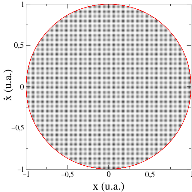
Fig. 4-3 : Comparaison entre le nuage de 32000 particules à l'instant t=0 (u.a.) de densité initiale uniforme et l'enveloppe convexe calculée à partir de ses moments
