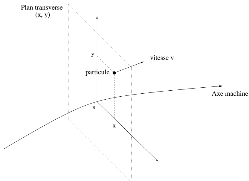
Fig. 1-1 : Référentiel général d'une particule
