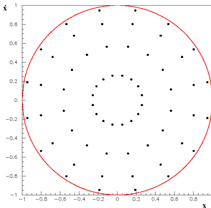
Fig. 3-2 : Réseau circulaire de 64 points adapté à une densité uniforme sur le disque de rayon unité
