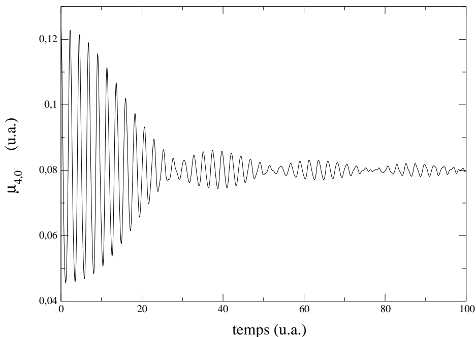
Fig. 3-13 : Evolution du moment \mu_{4,0} calculée à partir du nuage de points en fonction du temps
