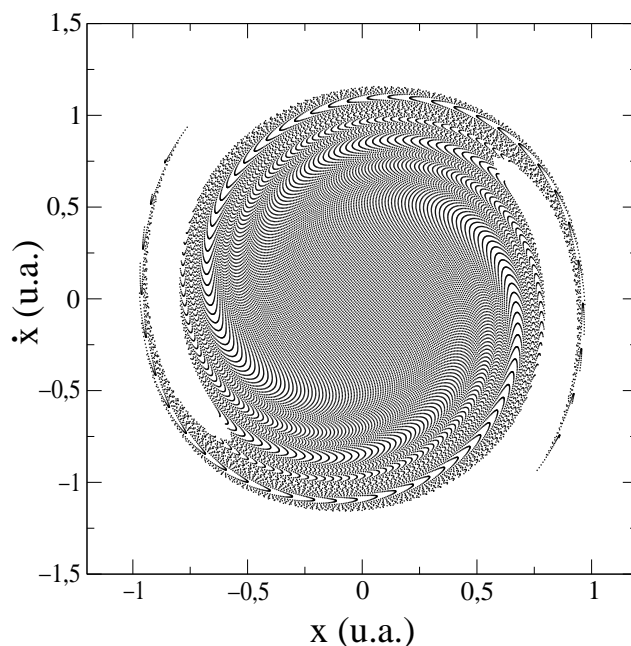
Fig. 4-14 : Nuage de particules dans l'espace de phases à t=20 (u.a.) avec pour densité initiale la densité uniforme sur le disque
