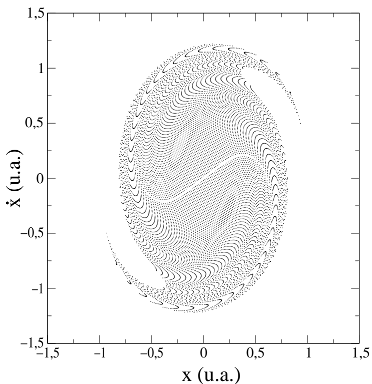
Fig. 3-4 : Distribution du nuage de points à t=15 dans l'espace des phases (x, \dot{x})
