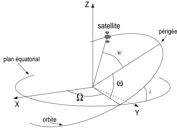
FIG. 1.1 – Éléments orbitaux.
