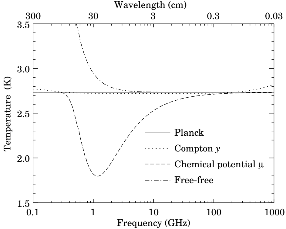
FIG. 1.3 – Écarts au corps noir. Ces écarts n'ont pas été observés jusqu'à présent. Cette figure provient aussi de [Smoot, 1997].
