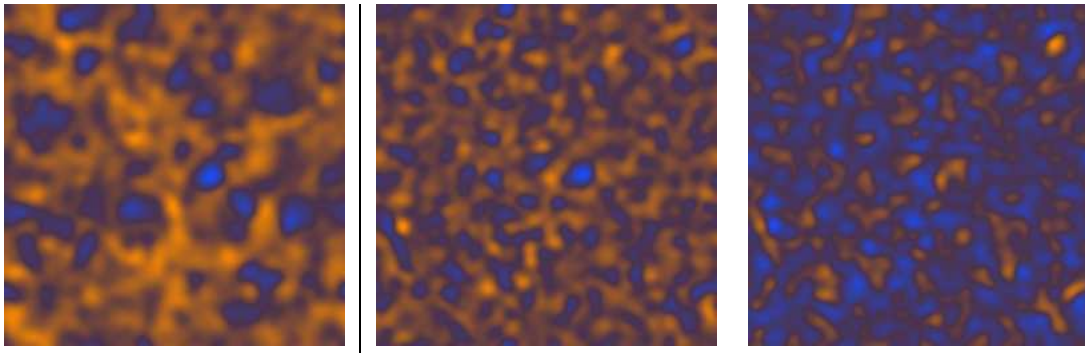
FIG. 9.6 – Des exemples de résultats. À gauche un champ de polarisation magnétique. À droite, les champs b_{\Delta} et b_{\nabla} définis au chapitre 8. Les figures sont filtrées à 5' . On retrouve des éléments caractéristiques entre les champs B et b_{\Delta} . Le champ b_{\nabla} semble présenter moins de structures communes. Ce comportement est tout à fait attendu à cette échelle de filtrage (voir figure 7.2)
