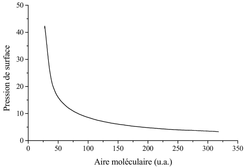
Figure 2.12 – Isotherme du copolymère 375/1730 déposé à partir d'une solution eau/méthanol. L'axe des abscisses représente l'aire moléculaire en \text{Å}^2/\text{molécule} en supposant que tout le copolymère reste à l'interface.
