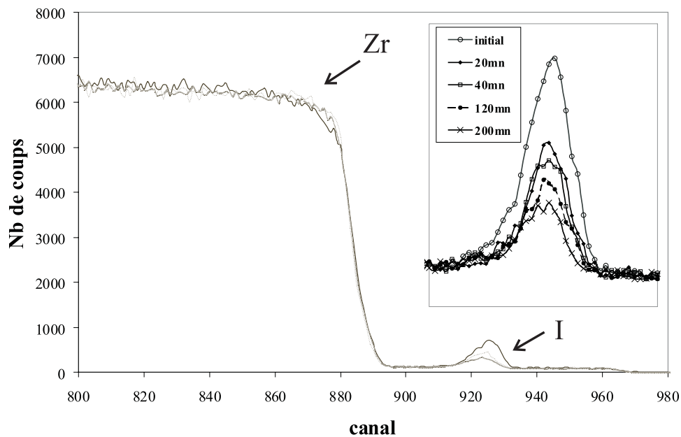
FIG. 3.3: Spectre global RBS ( E_{\alpha} = 3 MeV) d'un échantillon de zirconium implanté en iode stable à une énergie de 100 keV et une fluence de 10^{16} at.cm ^{-2} . L'encart représente l'évolution du profil d'iode à 700°C en fonction de la durée de recuit.
