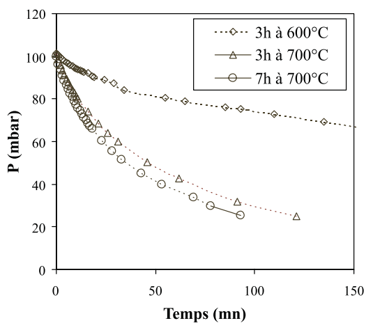
FIG. 2.15: Variations de la pression en hydrogène dans le tube en fonction de la température du recuit préliminaire et en fonction de la durée du recuit préliminaire à 700°C.
