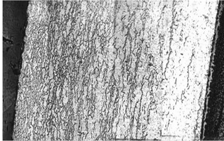
FIG. 1.4: Coupe transversale d'une gaine hydrurée (après cinq cycles annuels d'irradiation en REP). La face externe se trouve à gauche et la face interne à droite [Bailly 96].
