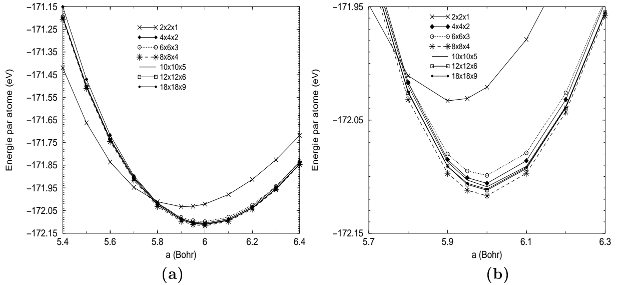
FIG. 5.5: Energie totale par atome (eV) calculée en fonction du paramètre de maille a (bohr) pour différents nombres de points \vec{k} (à E_C = 30 Ry fixée) pour la phase \alpha du zirconium. La figure b est un agrandissement de la figure a.
