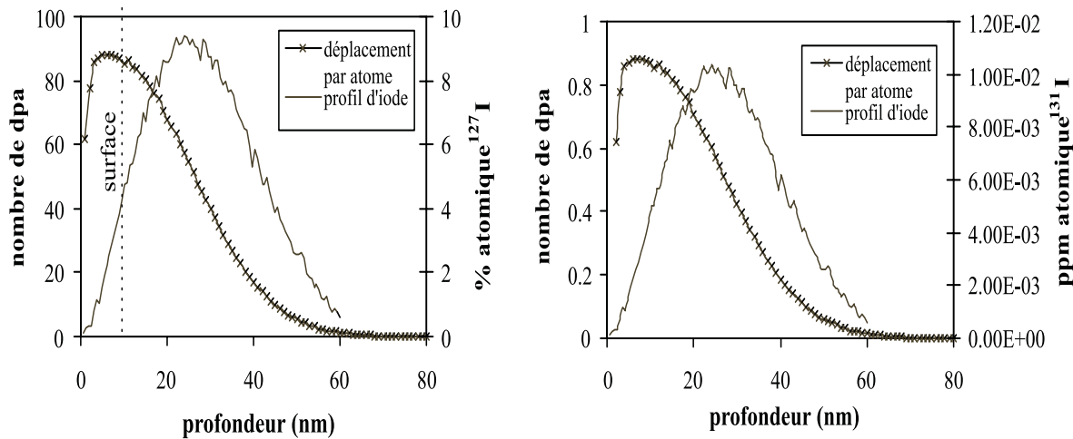
FIG. 3.1: Simulation du profil de distribution de l'iode implanté à 100 keV et du profil de déplacements par atome : a) à une fluence de 1.10^{16} atomes d'iode.cm ^{-2} , b) à une fluence de 1.10^9 atomes d'iode.cm ^{-2} et 1.10^{14} atomes de xénon.cm ^{-2}
