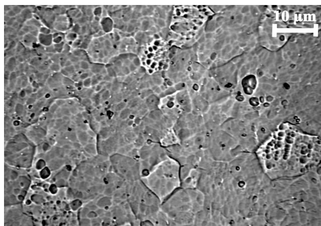
FIG. 2.1: Image obtenue au microscope optique d'un échantillon de zirconium révélation chimique.
