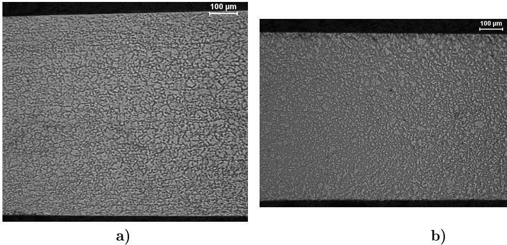
FIG. 2.17: Photos de microscopie optique réalisées sur des échantillons chargés à différents teneurs en hydrogène a) 1250 ppm et b) 3700 ppm.
