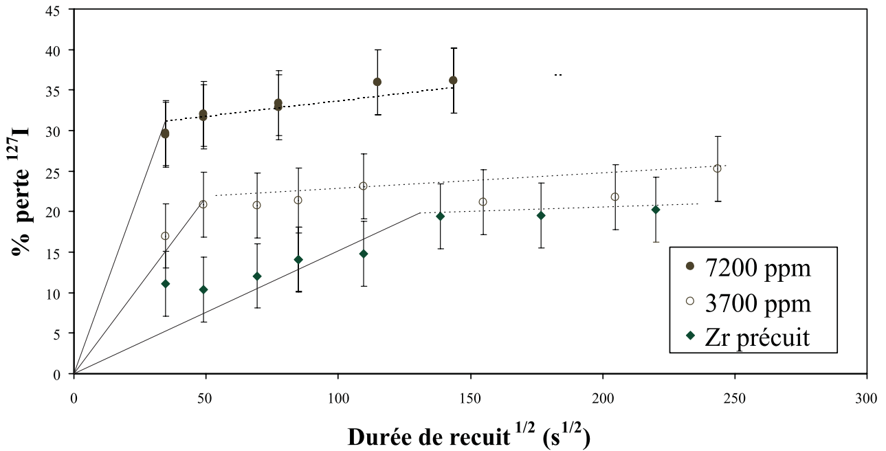
FIG. 4.7: Comparaison des pourcentages de perte en iode stable à 500°C pour des échantillons de zirconium polycristallin comportant différentes teneurs en hydrogène : 0, 3700 et 7200 ppm massique.
