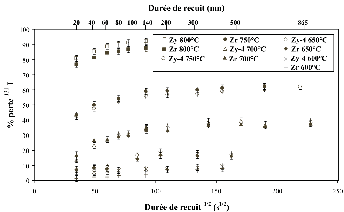
FIG. 4.2: Comparaison des pourcentages de perte en iode radioactif 131 I entre le zirconium et le Zircaloy-4.
