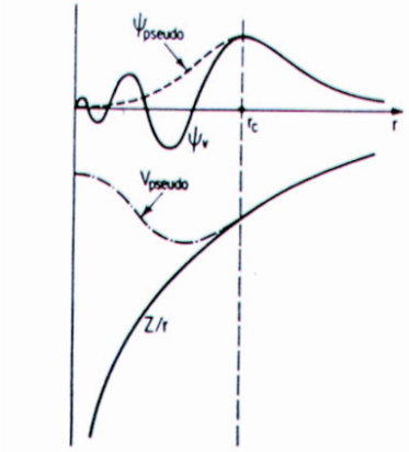
FIG. 5.1: Comparaison entre le potentiel du noyau et le pseudo-potential et leurs fonctions d'onde correspondantes.
