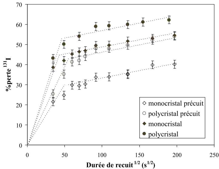
FIG. 4.3: Evolution à 750°C des pourcentages de perte en iode radioactif 131 I dans le zirconium polycristallin et monocristallin non précuits et dans les mêmes matériaux précuits sous vide à 700°C pendant 1 heure.
