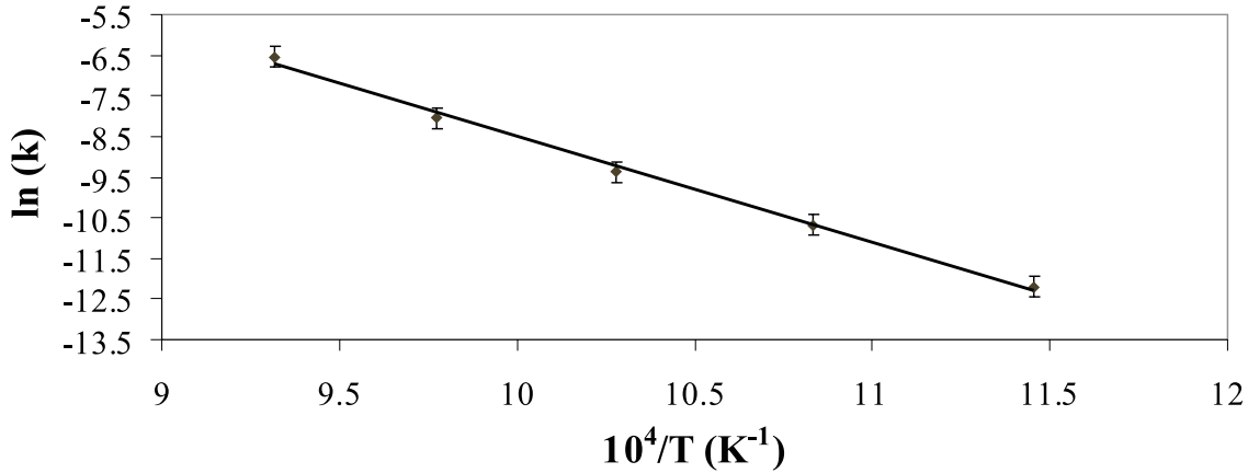
FIG. 3.19: Diagramme d'Arrhenius du relâchement de l'iode dans le zirconium.
