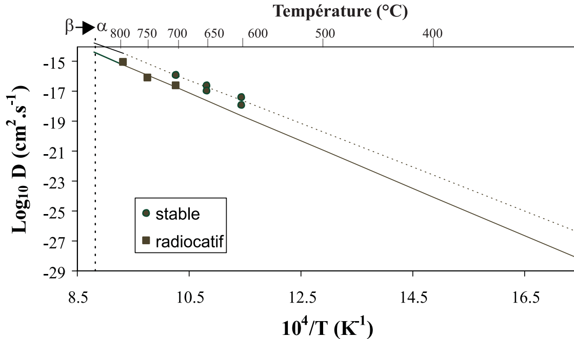
FIG. 6.2: Diagramme d'Arrhenius de la diffusion de l'iode stable et de l'iode radioactif dans le zirconium. Valeurs expérimentales (symboles) et droites d'Arrhenius extrapolées jusqu'à 300°C.
