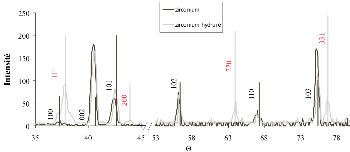
FIG. 2.18: Spectres de diffraction X réalisés sur un échantillon de zirconium vierge (noir) et sur un échantillon de zirconium refroidi à une vitesse de 1^{\circ}\text{C}\cdot\text{mn}^{-1} après chargement en hydrogène (rouge). Les raies caractéristiques du zirconium sont représentées en noir (N° JCPDS : 05-0665) et celles de l'hydrure \delta\text{-ZrH}_{1,66} en rouge (N° JCPDS : 34-0649).
