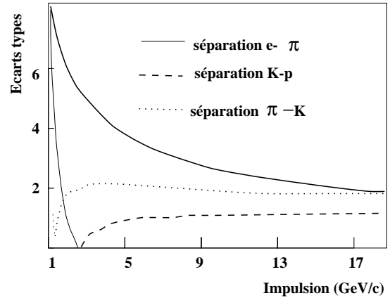
Figure 3.12: Différences attendues de dE/dx , en nombre d'écart types, pour plusieurs couples de particules en fonction de leur impulsion.
