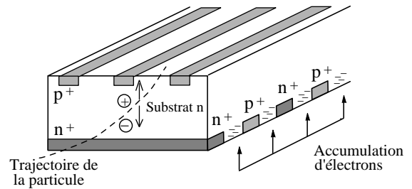
Figure 3.6: Détail de fonctionnement du VDET.
