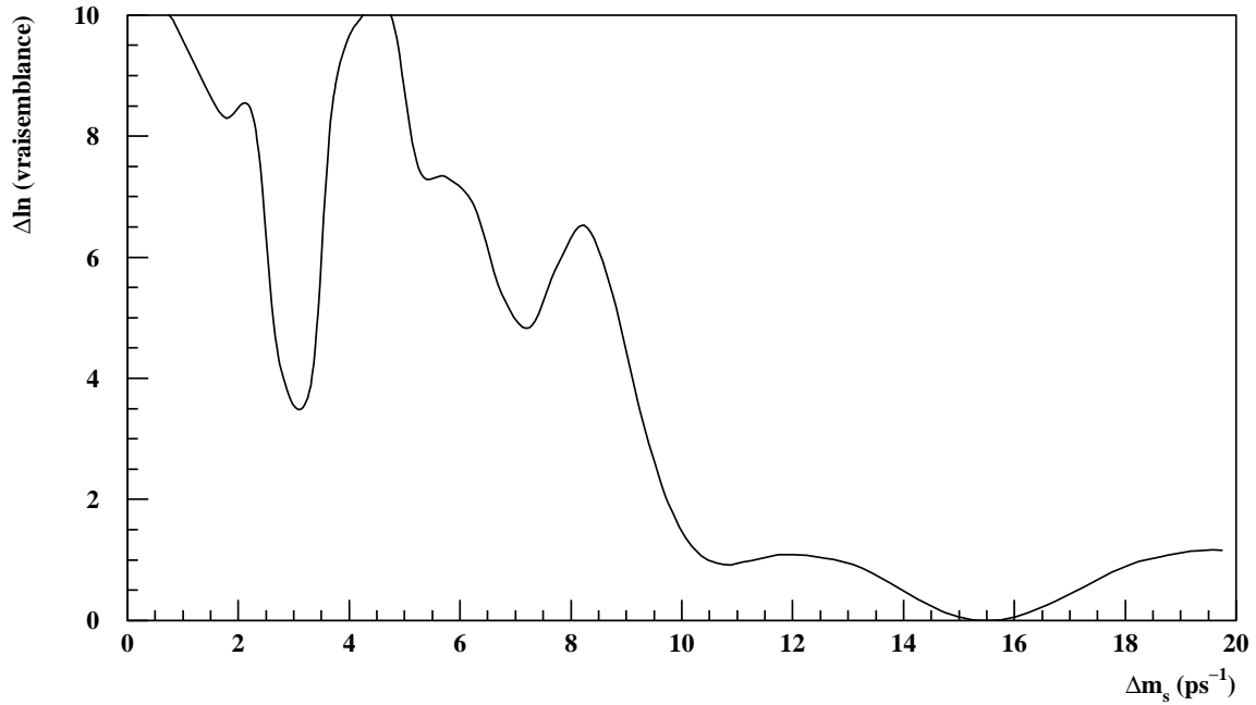
Figure 6.4: \Delta \ln \mathcal{L} en fonction de \Delta m_s , dans les données (voir le texte).
