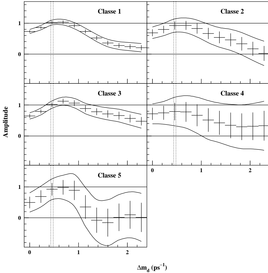
Figure 6.15: Amplitude d'oscillation des B_d^0 mesurée en fonction de \Delta m_d dans les cinq classes d'étiquetages, dans les données. Les lignes pointillées verticales correspondent à la valeur ajustée de \Delta m_d dans tout l'échantillon, par la méthode du maximum de vraisemblance : \Delta m_d = 0.457 \pm 0.024 ps -1 . Les barres d'erreur représentent l'incertitude statistique à 1\sigma et les courbes en trait plein les contours d'exclusion à 95% CL (sans les incertitudes systématiques).
