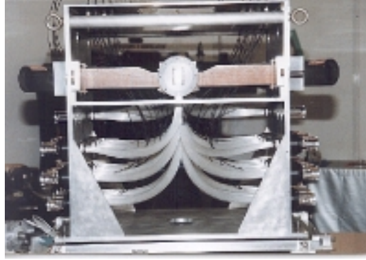
FIG. 1.12: Photographie de la cible active de NA38.
