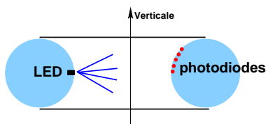
Figure 3.14 : Principe de la ligne de mesure de la salissure.
