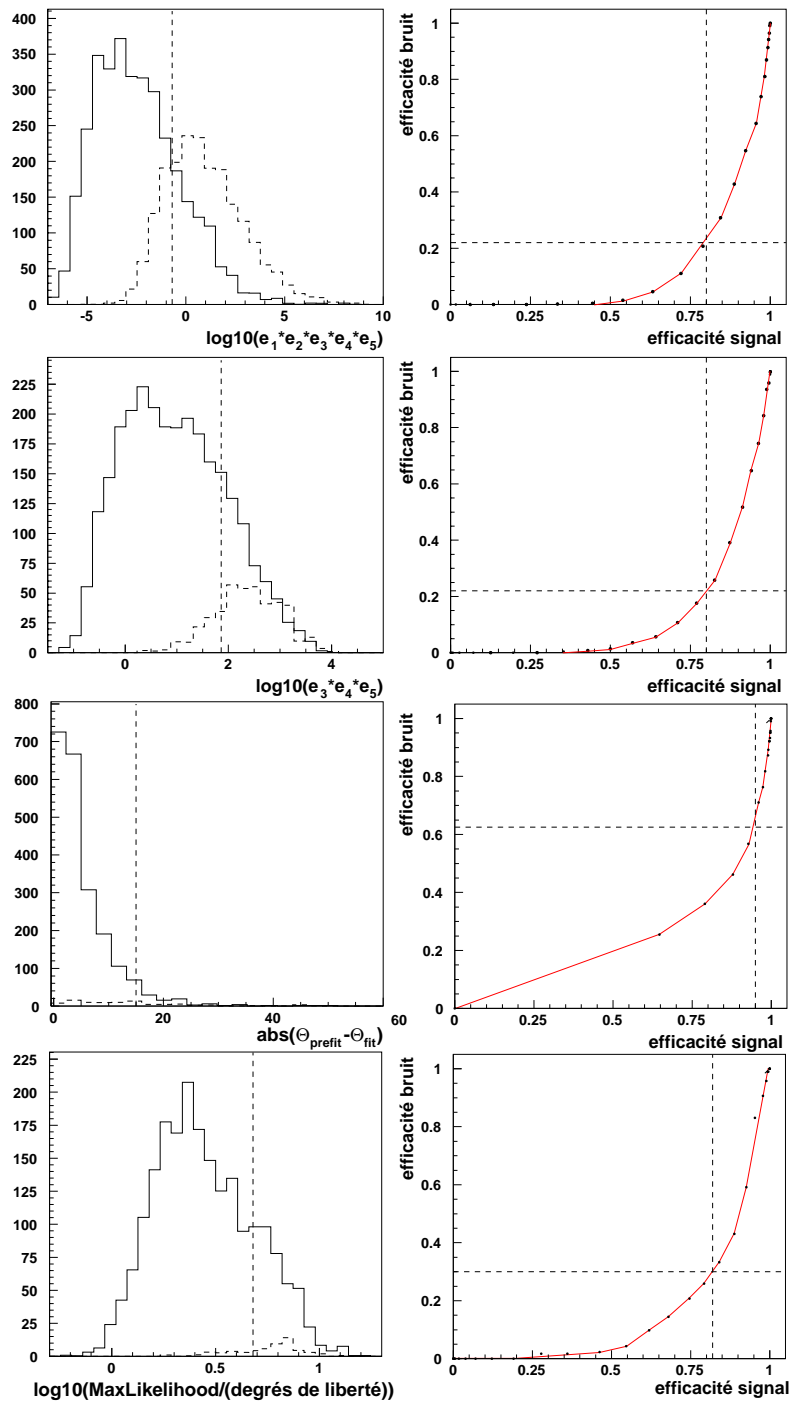
Figure 4.11 : Les distributions des variables discriminantes pour les événements multi-ligne, dans le cas du signal (continu) et du bruit de fond (tirets) sont présentées dans les figures de gauche, ainsi que les coupures appliquées. A droite, les courbes d'efficacité du bruit par rapport au signal, en variant la valeur des coupures.
