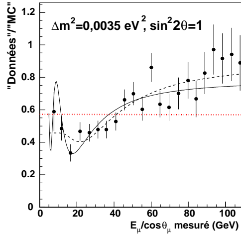
Figure 5.9 : Spectre d'oscillation pour une "expérience" typique avec 3 ans d'acquisition de données et en supposant des oscillations avec \sin^2 2\theta = 1 et \Delta m^2 = 3,5 \cdot 10^{-3} \text{ eV}^2 . La ligne horizontale est le niveau moyen utilisé pour tester la sensibilité aux oscillations et la ligne en tirets \langle \mathcal{P} \rangle (équation 5.3) utilisé pour obtenir les paramètres d'oscillations. La ligne continue est un autre exemple possible pour \langle \mathcal{P} \rangle (équation 5.2).
