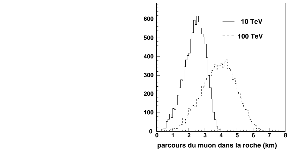
Figure 2.13 : Distribution des parcours des muons de 10 TeV ou 100 TeV dans la roche dite "standard".
