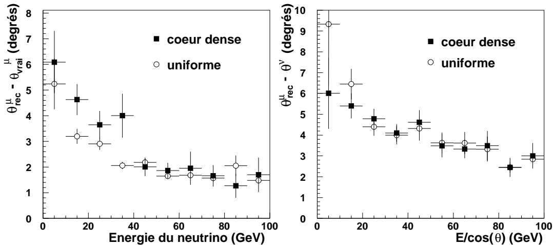
Figure 4.22 : A gauche, |\theta_{\mu}^{vrai} - \theta_{\mu}^{rec}| (la résolution “de reconstruction”) est représentée en fonction de l’énergie du neutrino pour les deux géométries considérées. Toujours pour les deux géométries, la résolution globale sur le zénith du neutrino est représentée à droite en fonction de E/\cos\theta du neutrino.
