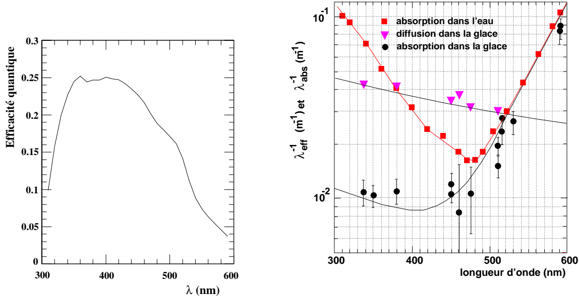
Figure 2.9 : Absorption et diffusion dans la glace, mesurées par la collaboration AMANDA à une profondeur de 1,7 km [61], et absorption dans l'eau de mer, telle qu'elle a été mesurée par les collaborations DUMAND [62] et NESTOR [63].
