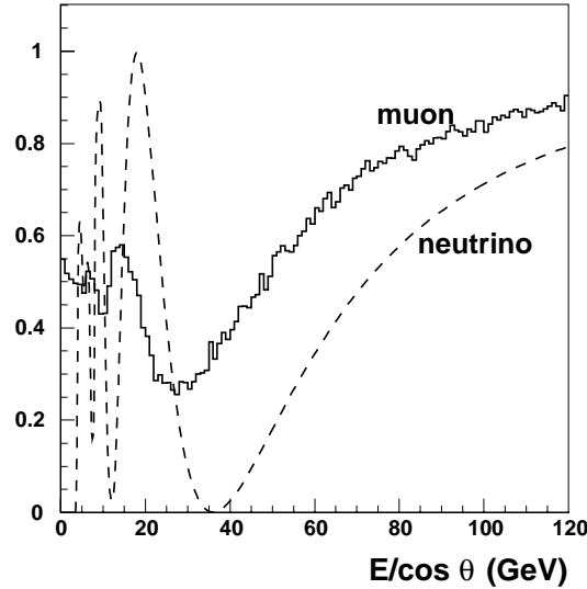
Figure 5.2 : Probabilité de survie de neutrinos ascendants en fonction de x = E/\cos\theta , quand x est donné par les vraies valeurs des neutrinos ou par les valeurs correspondantes des muons qu'ils engendrent.
