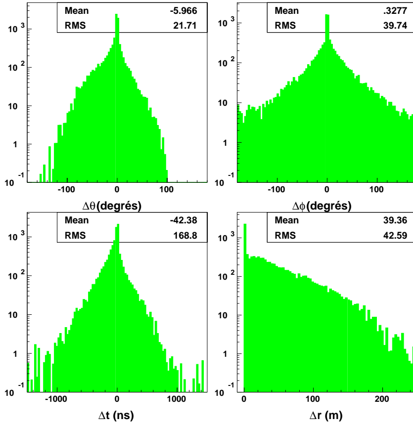
Figure 4.6 : Distributions des erreurs de la procédure de reconstruction multi-ligne sur les angles de la trace (zénith et azimuth), son temps et sa distance d’approche minimale au centre du détecteur.
