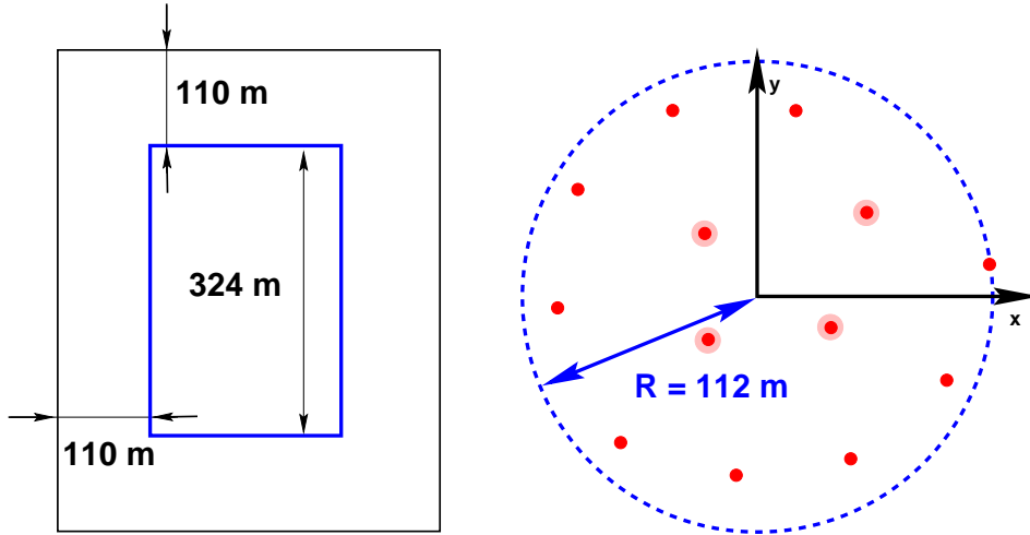
Figure 4.21 : Vue latérale et de haut des géométries envisagées pour le détecteur. A noter que la “canette” de simulation (rectangle extérieur) a un rayon double par rapport au volume instrumenté (rectangle intérieur). A droite, les quatre lignes centrales, qui sont plus denses dans le cas de la géométrie à cœur dense sont soulignées.
