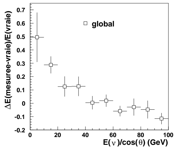
Figure 4.20 : Résolution globale sur l'énergie du muon en fonction de E/\cos\theta du neutrino.
