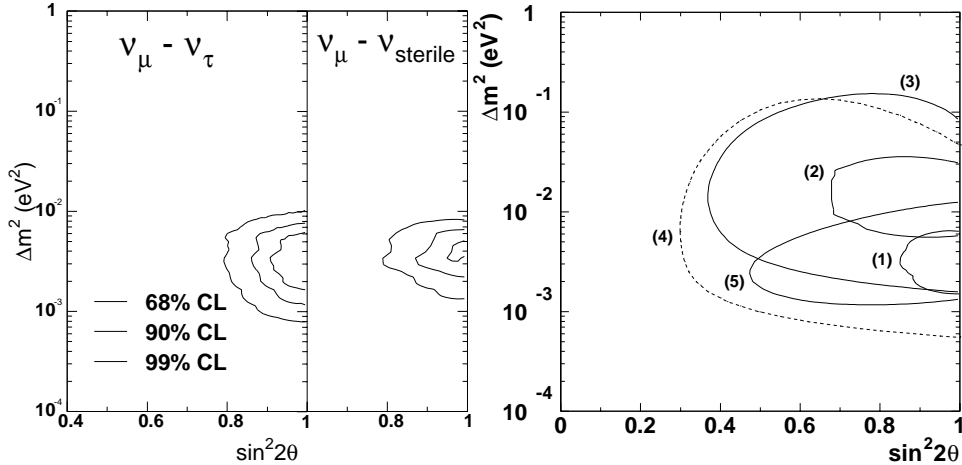
Figure 1.9 : Gauche : régions permises dans l'espace des paramètres d'oscillation, dans l'hypothèse \nu_\mu \rightarrow \nu_\tau et \nu_\mu \rightarrow \nu_s [33]. A droite, les régions permises à 90% de degré de confiance pour l'oscillation \nu_\mu \rightarrow \nu_\tau , telles qu'elles résultent de : l'analyse des événements contenus de SuperKamiokande (1) et Kamiokande (2) ; l'analyse des événements partiellement contenus de SuperKamiokande (3) et Kamiokande (4) ; le rapport des muons contenus et non-contenus dans SuperKamiokande (5).
