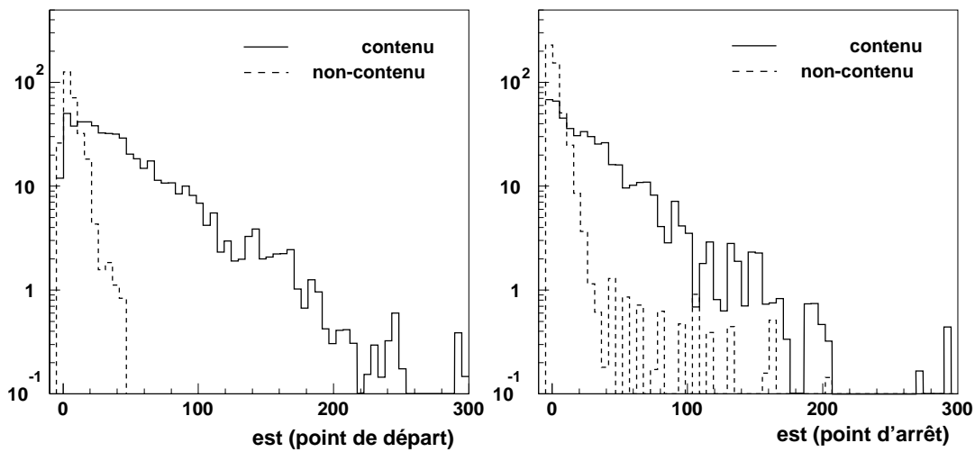
Figure 4.18 : L'estimateur de point contenu pour le point de départ et le point d'arrêt de la trace.
