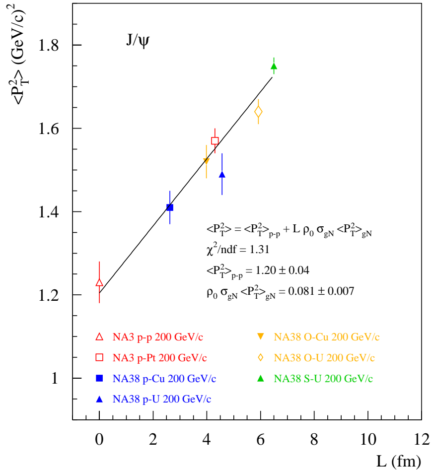
Figure 39: Ajustement des valeurs de \langle P_T^2 \rangle obtenues pour le J/ψ pour une énergie incidente de 200 GeV. Les points p-p et p-Pt n'ont pas été mesurés par NA38, mais par l'expérience NA3 [53].
