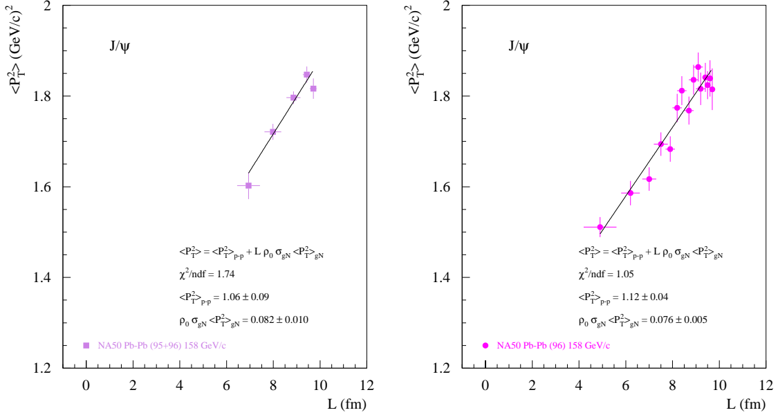
Figure 41: Ajustement des données Pb-Pb réparties en 5 (cumul des données de 1995 et 1996 avec sélection cible) et 15 (données de 1996 sans sélection cible) intervalles de E_T^0 .
