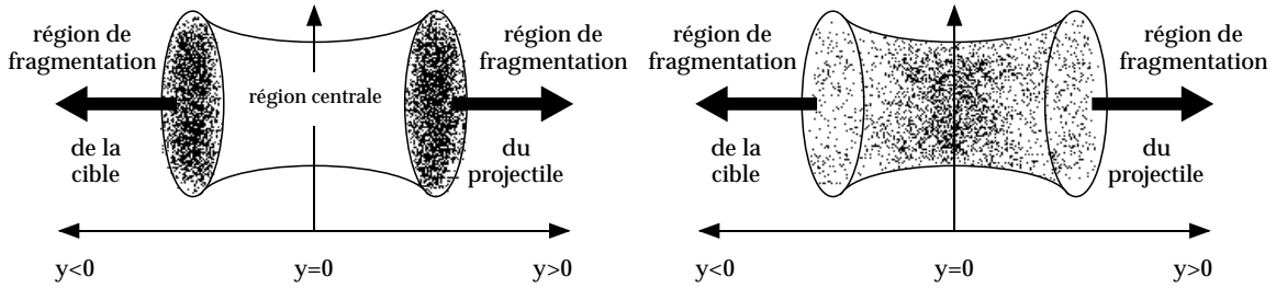
Figure 1: Représentation schématique d'une collision noyau-noyau dans son centre de masse. Après la collision, les deux noyaux laissent derrière eux une zone dite "de rapidité centrale", très excitée. Dans le cas idéal où les noyaux sont transparents l'un à l'autre, tout le nombre baryonique initial se trouve dans les régions de fragmentation de la cible et du projectile (figure de gauche). Aux énergies de l'AGS, et du SPS, une partie du nombre baryonique est déplacé vers la région centrale (figure de droite).
