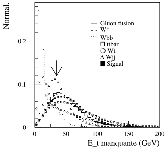
FIG. 4.7 – Distribution de l'énergie transverse manquante. Le signal représenté ici correspond à la production d'un \tilde{s} -quark de masse 300 GeV et de largeur 0.5 GeV. La somme des événements a été normalisée à 1.
