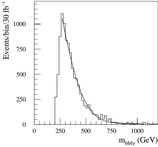
FIG. 4.18 – Fit sur la distribution en masse invariante pour les bruits de fond.
