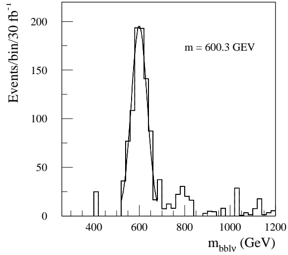
FIG. 4.19 – Signal une fois le bruit de fond retranché.
