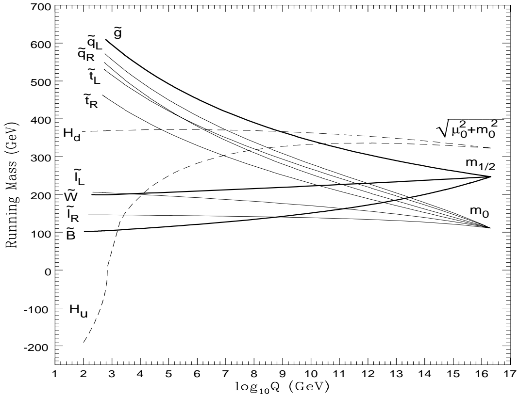
FIG. 1.4 – Évolution des masses des s -particules depuis l'échelle GUT, jusqu'à l'échelle électrofaible, dans un modèle mSUGRA . La brisure de la symétrie électrofaible est obtenue lorsque la masse du champ de Higgs H_u devient négative.
