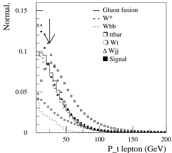
FIG. 4.8 – Distribution de l'impulsion transverse pour le premier lepton. Le signal représenté ici correspond à la production d'un \tilde{s} -quark de masse 300 GeV et de largeur 0.5 GeV. La somme des événements a été normalisée à 1.
