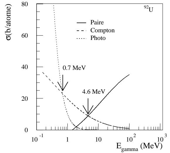
FIG. 3.2 – Dans l'uranium
