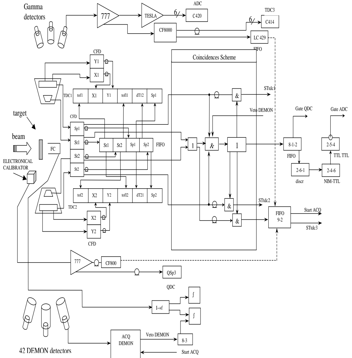
Figure 7.13 : Schéma électronique.
