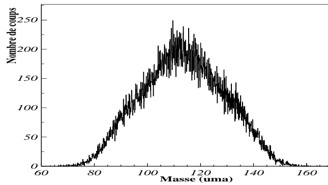
Figure 8.3 : Distribution de masse des fragments de fission du ^{227}\text{Pa} synthétisé par la réaction : ^{18}\text{O} (78\text{MeV}) + ^{209}\text{Bi} \rightarrow ^{227}\text{Pa} .
