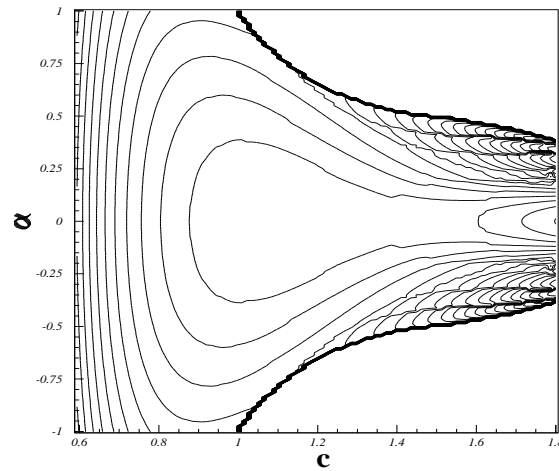
Figure 5.2 : Energie de déformation dans l'espace des paramètres de déformation de Funny-Hills ( c, \alpha, h_{min} ) dans le cadre du modèle de la goutte liquide. La valeur h_{min} est obtenue, pour chaque couple (c, \alpha) , après minimisation de l'énergie par rapport au paramètre de déformation h de Funny-Hills.
