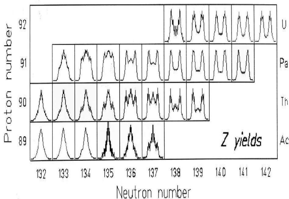
Figure 1.2 : Distributions de charge des fragments de fission de quelques isotopes de l'actinium Ac, du thorium Th, du protactinium Pa et de l'uranium U [12]. Pour un élément donné, on peut noter la transition progressive de la fission symétrique vers la fission bimodale en passant d'un isotope à un autre.
