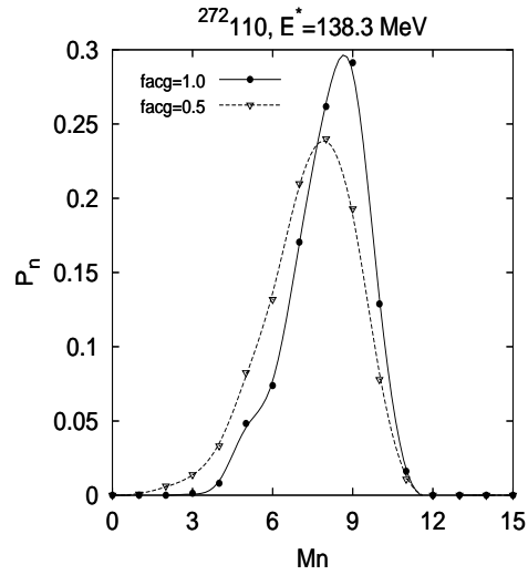
Figure 4.2 : Distributions de multiplicité de neutrons de pré-scission pour le noyau composé ^{272}_{110} pour une friction “complète” ( \text{facg}= 1.0 ) et une friction “réduite” ( \text{facg}= 0.5 ).
