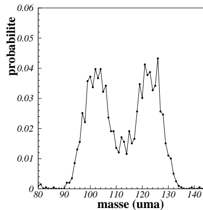
Figure 10.4 : Distribution de masse des fragments de fission obtenue pour un paysage énergétique dans lequel les effets de couche ont été calculés par la méthode d'interpolation entre c = 1.8 et c_{g\acute{e}om} (voir texte).
