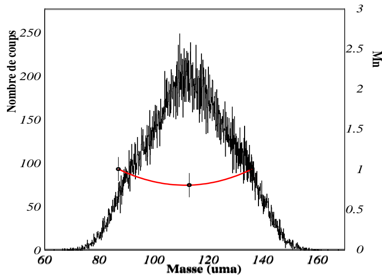
Figure 9.3 : Distribution de masse des fragments de fission (trait fin noir) et multiplicité de neutrons de pré-scission (trait gras rouge).
