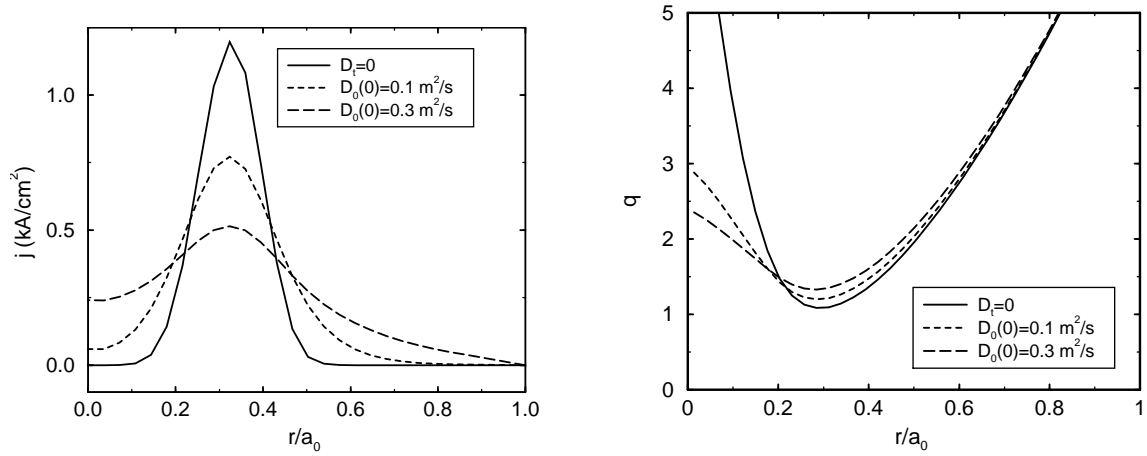
FIG. 7.2 – (a) Profil de courant généré par l'onde hybride basse pour trois valeurs du coefficient de diffusion radiale dans la décharge n° 12975 : D_0(0) = 0 ( trait plein ), D_0(0) = 0.1 m 2 /s ( tirets courts ) et D_0(0) = 0.3 m 2 /s ( tirets longs ). En (b) sont représentés les profils de q correspondants.
