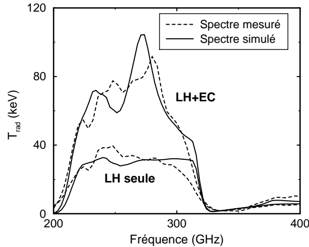
FIG. 7.9 – Comparaison des spectres d'émission mesuré ( tirets ) et simulé ( trait plein ). L'augmentation de température radiative pendant la phase LH+EC est due à l'interaction de l'onde EC avec les électrons suprathermiques de la queue LH.
