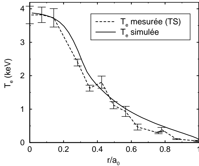
FIG. 7.3 – Comparaison de la température électronique mesurée ( Trait pointillé ) et simulée ( Trait plein ) pour la décharge n° 12975 et pour D_0(0) = 0.1 m 2 /s.
