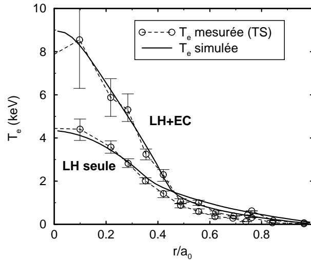
FIG. 7.13 – Comparaison de la température électronique mesurée ( Trait pointillé ) et simulée ( Trait plein ) pour la décharge n° 18369 pendant la phase LH, puis pendant la phase LH+EC après modification du modèle de transport de la chaleur ( voir texte ).
