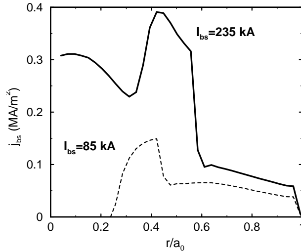
FIG. 6.18 – Profils de courant de bootstrap correspondant aux deux cas de la figure 6.16. Phase LH seule ( tirets ) et phase LH+EC ( trait épais ).
