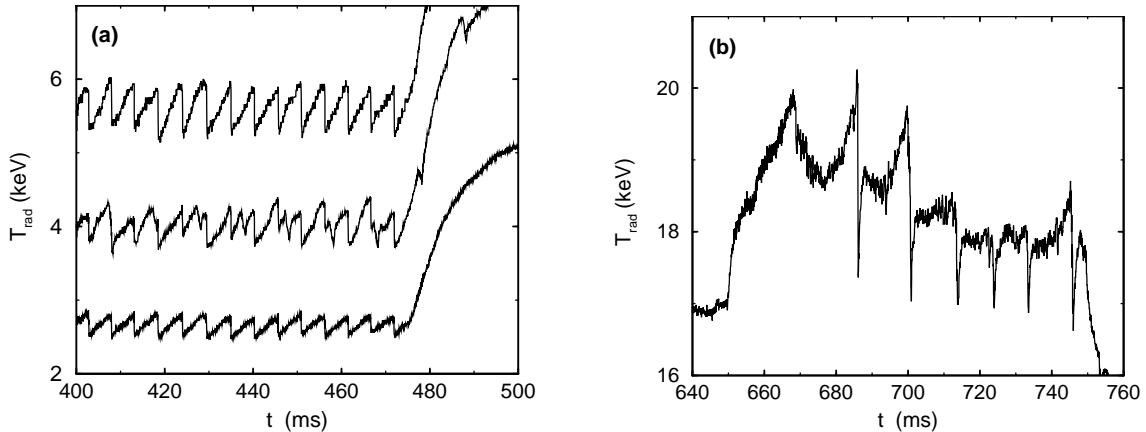
FIG. 7.7 – Agrandissement de la figure 7.6. (a) Phase ohmique : les dents de scie apparaissent très clairement. (b) Phase LH+EC : Relaxations rapides de la température centrale.
