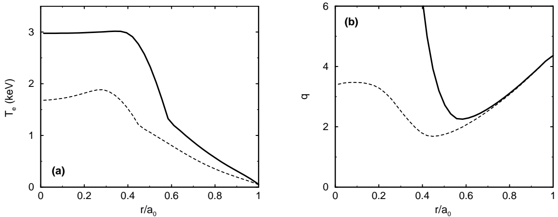
FIG. 6.16 – Résultat des simulations K+T pour le profil de température (a) et de facteur de sécurité (b), dans le cas où l'onde cyclotronique électronique est initialement déposée plus hors de l'axe que l'onde hybride basse ( r_{ec}/a_0 \approx 0.53 > r_{lh}/a_0 \approx 0.39 ). Phase LH seule (tirets) et phase LH+EC (trait épais).
