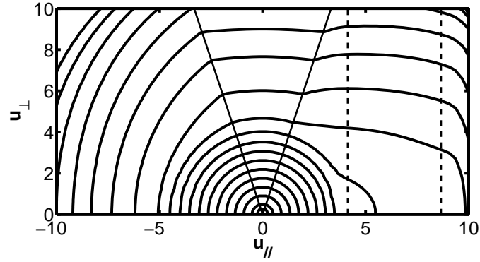
FIG. 4.7 – Contours de la fonction de distribution en présence d'onde hybride ( P_{lh} = 4\text{MW} ) pour r/a_0 \approx 0.1 . Les droites en trait plein délimitent le cône de perte local. Les droites en pointillés représentent les frontières approximatives du coefficient de diffusion quasilinéaire.
