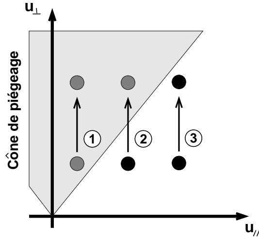
FIG. 2.14 – Effet des électrons piégés. Dans la situation (1), l'électron ne participe pas au courant. A l'inverse, dans la situation (3), il est en mesure de contribuer au courant toroïdal. Dans le cas (2), l'électron est poussé dans le cône de piégeage et perdu pour la génération de courant.
