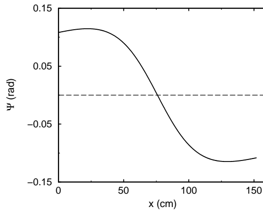
FIG. 3.6 – Angle de cisaillement en fonction de x , dans le cas où q_0 = 1 , q_a = 3 et où le profil de q est parabolique. On a pris ici B_0(0) = 2.1\text{T} .
