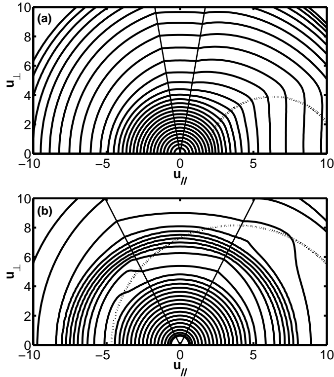
FIG. 4.1 – Contours de la fonction de distribution en présence d'onde cyclotronique électronique ( P_{ec} = 3\text{MW} ). Les droites en trait plein délimitent le cône de perte local. L'ellipse de résonance pour le rayon central figure également. (a) Cas upshift : n\omega_{ce}/\omega \approx 0.9 ( r/a_0 \approx 0.1 ). (b) Cas downshift : n\omega_{ce}/\omega \approx 1.1 ( r/a_0 \approx 0.5 ).
