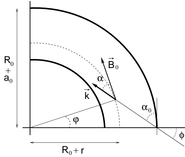
FIG. 3.12 – Modification de n_{\parallel} = \cos(\alpha) au cours de la propagation de l'onde en géométrie toroïdale. L'angle d'injection \phi_t est le complémentaire de \alpha_0 \equiv \alpha(x = 0) .
