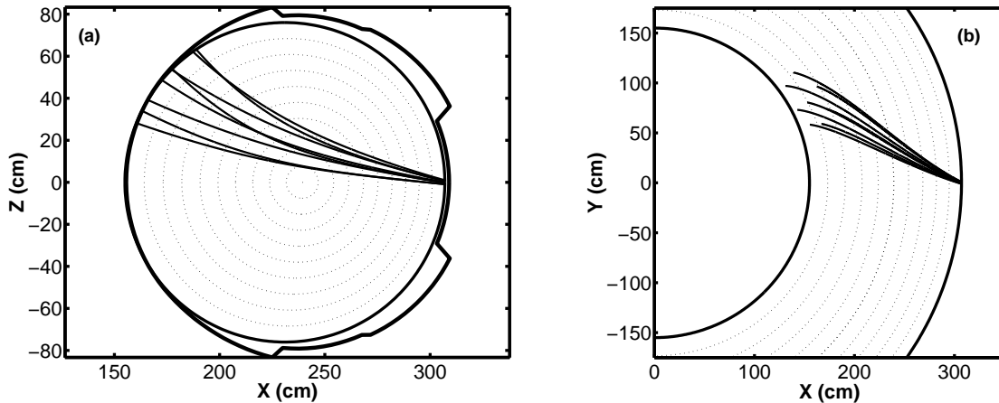
FIG. 2.9 – Exemple de trajectoires de huit rayons : (a) Projection poloïdale (b) Projection toroïdale. Le plasma cible est tel que n_{e0} = 4 \times 10^{13}\text{cm}^{-3} , T_{e0} = 5\text{keV} , B_0 = 2\text{T} . Le faisceau simulé est caractérisé par \phi_t = 20^\circ et \theta_p = 10^\circ . Le mode choisi est extraordinaire et résonne au deuxième harmonique de la résonance cyclotronique électronique.
