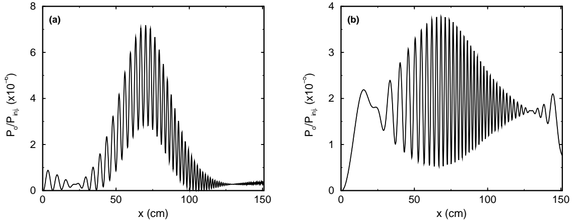
FIG. 3.7 – Fraction de mode ordinaire générée sous l'effet du cisaillement magnétique dans le cas d'un plasma tel que B_0(0) = 2.1\text{T} . (a) Cas d'une densité homogène avec n_e = 5 \times 10^{13}\text{cm}^{-3} . (b) Profil de densité parabolique avec n_e(0) = 5 \times 10^{13}\text{cm}^{-3} .
