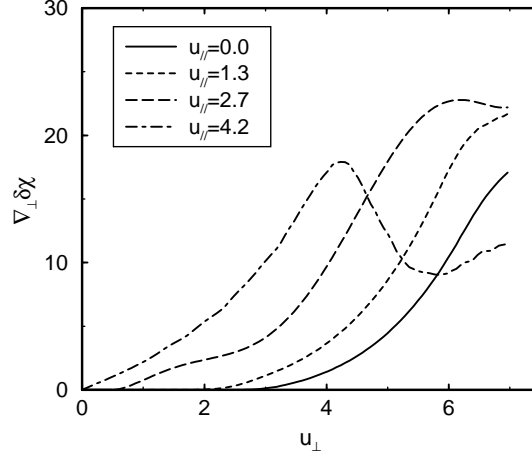
FIG. 5.9 – Coupes de \mathbf{S}_{ec} \cdot \partial \delta \chi / \partial \mathbf{u} \propto \partial \delta \chi / \partial u_{\perp} , en fonction de u_{\perp} pour u_{\parallel} = 0.0 , u_{\parallel} = 1.3 , u_{\parallel} = 2.7 et u_{\parallel} = 4.2 .
