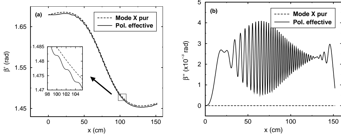
FIG. 3.11 – Caractéristiques de l'ellipse de polarisation. (a) \beta' , angle d'inclinaison du grand axe par rapport à l'axe défini par \hat{\mathbf{e}}_{\parallel} . Sur le même graphique figure cet angle dans le cas où il n'y a pas de couplage ( pointillés ). (b) \beta'' , angle d'ouverture : \tan(\beta'') est le rapport des longueurs des axes de cette ellipse (voir figure 3.3).
