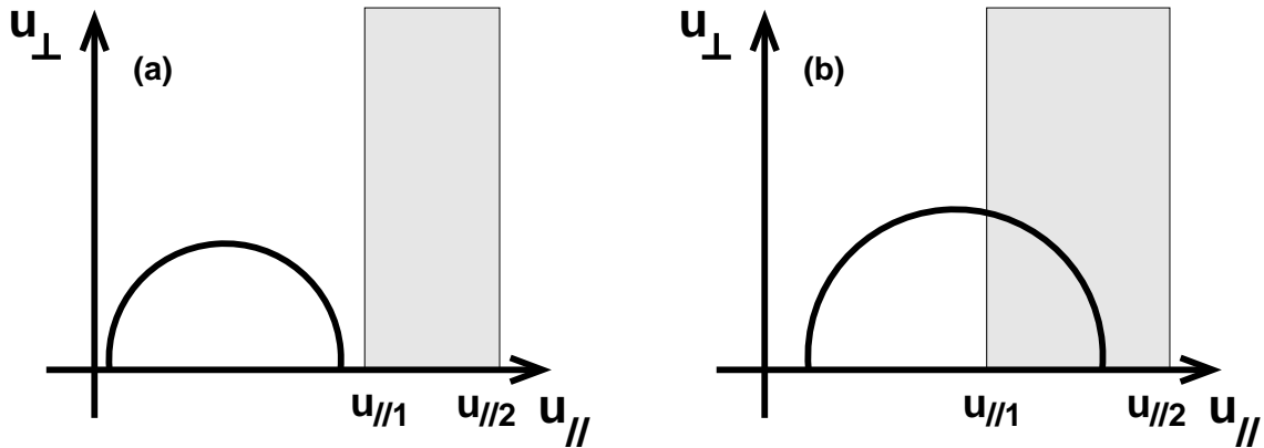
FIG. 5.1 – Illustration schématique de la position respective des domaines correspondant aux coefficients de diffusion quasilinear de l'onde hybride basse et de l'onde cyclotronique électronique dans l'espace des vitesses. (a) Sans recouvrement ; (b) Avec recouvrement des domaines.
