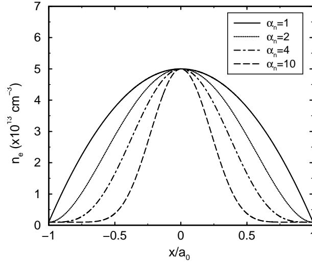
FIG. 3.14 – Profils de densité pour différentes valeur du paramètre \alpha_n . Les autres paramètres sont n_{e_0} = 5 \times 10^{13} \text{ cm}^{-3} et n_{e_a} = 0.1 \times 10^{13} \text{ cm}^{-3} .
