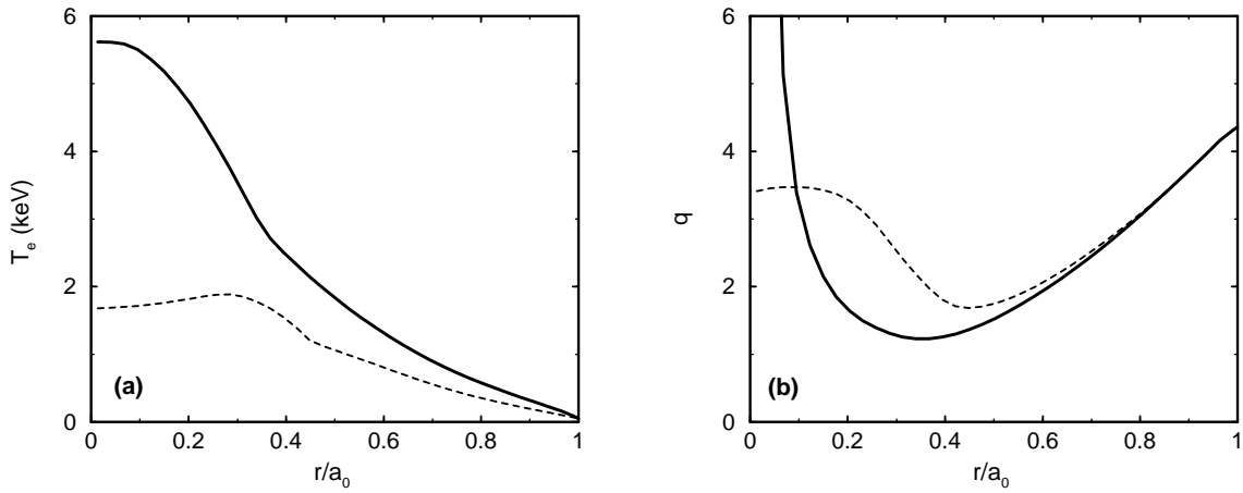
FIG. 6.19 – Idem à la figure 6.16 pour un dépôt EC initialement plus central que le dépôt LH ( r_{ec}/a_0 \approx 0.25 < r_{lh}/a_0 ). L'angle d'injection toroïdal vaut \phi_t = -15^\circ (contre-courant).
