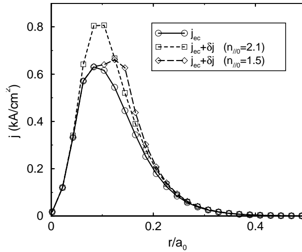
FIG. 5.13 – Profil de courant généré par l'onde cyclotronique électronique ( P_{ec} = 3 \text{MW} ) en l'absence d'onde hybride basse ( trait continu ), en présence d'onde hybride basse lancée à n_{||0} = 2.1 ( tirets courts ) et n_{||0} = 1.5 ( tirets longs ).
