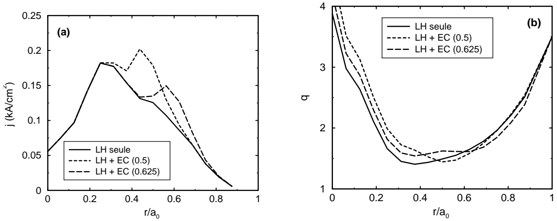
FIG. 6.1 – (a) Profils de courant généré et (b) de facteur de sécurité. Phase LH seule ( Trait plein ), phase LH+EC absorbée à r_{ec}/a_0 \approx 0.5 ( Tirets courts ). LH+EC absorbée à r_{ec}/a_0 \approx 0.625 . Sur cette figure P_{ec} = 2.4\text{MW} , P_h = 2.5\text{MW} , n_{e0} = 3 \times 10^{13}\text{cm}^{-3} et T_{e0} = 6\text{keV} .
