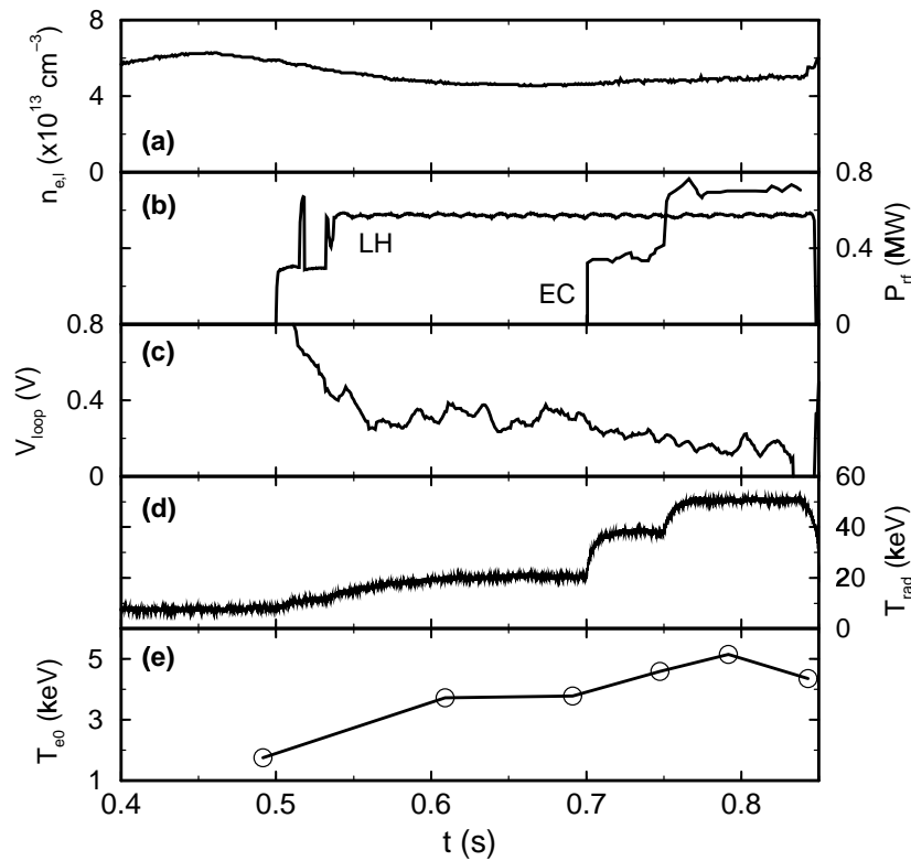
FIG. 7.8 – Evolution des différents paramètres de la décharge n° 18181. Les différentes quantités représentées sont : (a) Densité linéique moyenne (DCN); (b) Puissance hybride et cyclotronique électronique; (c) Tension par tour; (d) Température radiative (polychromateur ECE; R = 94.4\text{cm} ); (e) Température électronique centrale (TS).
