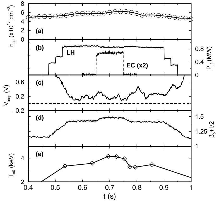
FIG. 7.4 – Evolution temporelle des différents paramètres de la décharge n° 12685. Les différentes quantités représentées sont : (a) densité linéique moyenne (DCN) ; (b) puissance hybride et cyclotronique électronique ( \times 2 ) ; (c) tension par tour ; (d) \beta_p + l_i/2 ; (e) température centrale (TS).
