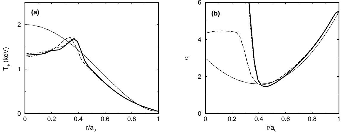
FIG. 6.4 – Profils de température électronique (a) et de facteur de sécurité (b) obtenus à l'aide du modèle K+T pour une puissance hybride P_{lh} = 3\text{MW} (2MW injectés à n_{\parallel 0} = 1.8 et 1MW injecté dans le lobe secondaire). Ici B_0(0) = 2\text{T} , I_p = 0.46\text{MA} , \tilde{b} = 0 . Les conditions initiales sont fixées arbitrairement ( voir texte ). Trait pointillé fin : Conditions initiales; Tirets longs : première itération; Tirets courts : deuxième itération (difficilement visible); Trait épais : troisième itération, correspondant à l'état stationnaire.
