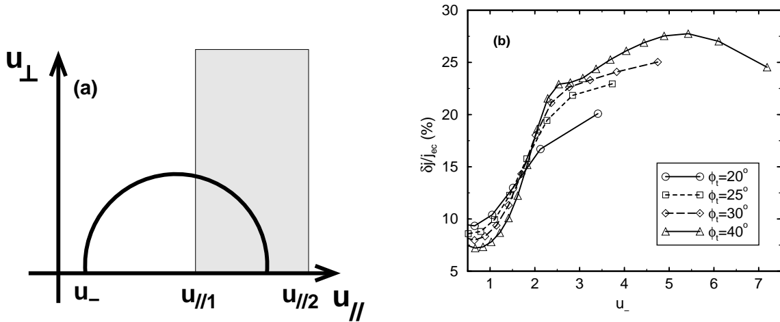
FIG. 5.11 – Amélioration de l'efficacité de génération de courant (b) pour plusieurs valeurs de l'angle toroïdal local, tel que \phi_t \equiv \arcsin(n_{||}) en fonction de la position de l'extrémité basse vitesse de l'ellipse (voir (a)).
