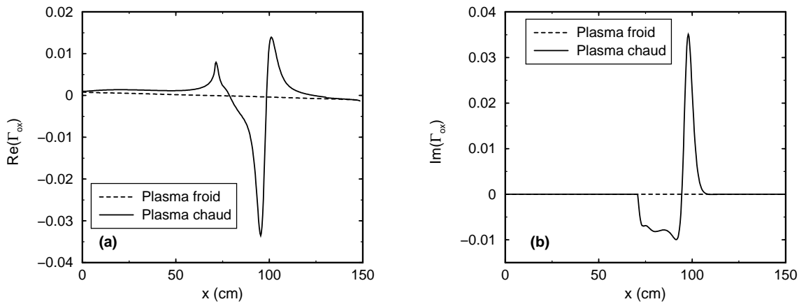
FIG. 3.15 – Exemple de coefficient de couplage \Gamma_{ox} : partie réelle (a), partie imaginaire (b). On a choisi ici n_{e_0} = 5 \times 10^{13} \text{ cm}^{-3} , T_{e_0} = 5 \text{ keV} , \phi_t = 10^\circ , \alpha_n = 1 et \alpha_T = 2 . Sur cette figure, la résonance cyclotronique électronique se trouve sensiblement au centre du plasma.
