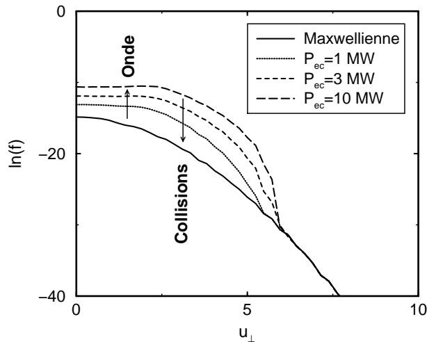
FIG. 2.2 – Fonction de distribution maxwellienne ( ligne continue ) et déformation quasilinear pour P_{ec} = 1\text{MW} ( pointillés ), P_{ec} = 3\text{MW} ( tirets courts ) et P_{ec} = 10\text{MW} ( tirets longs ), pour \varepsilon_{\parallel} = 60\text{keV} ( u_{\parallel} = 5 ). Les principaux paramètres du plasma sont n_{e0} = 3 \times 10^{13}\text{cm}^{-3} , T_{e0} = 5\text{keV} et B_0 = 3.8\text{T} . L'onde est lancée avec un angle de 15^\circ dans la direction toroïdale.
