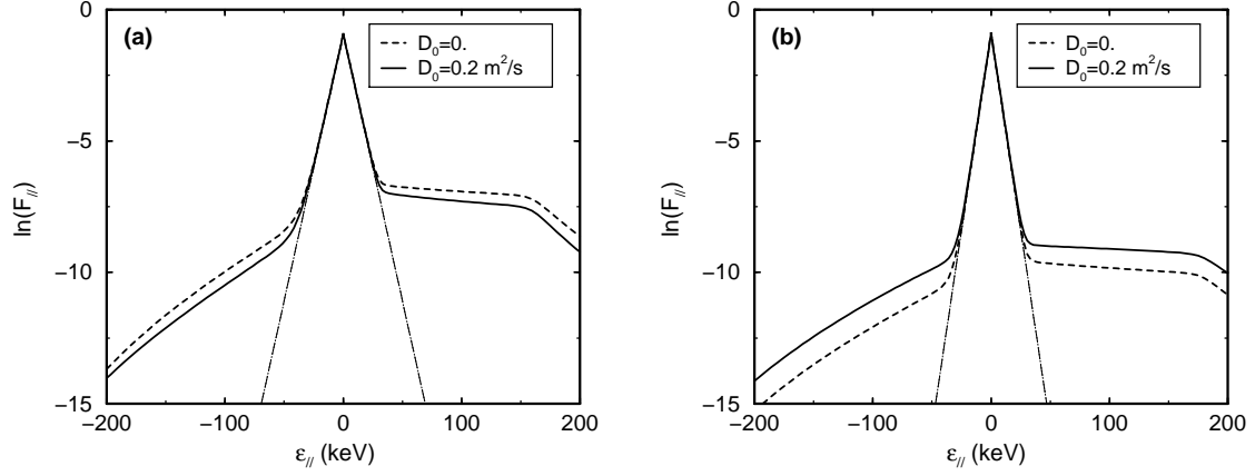
FIG. 4.15 – Fonction de distribution parallèle en fonction de l'énergie parallèle des électrons pour r/a_0 \approx 0.1 (a) et r/a_0 \approx 0.4 (b). Les niveaux de turbulence magnétique sont ici \tilde{b} = 0 (tirets) et \tilde{b} = 0.2 \times 10^{-4} (trait plein). La maxwellienne figure en pointillés.
