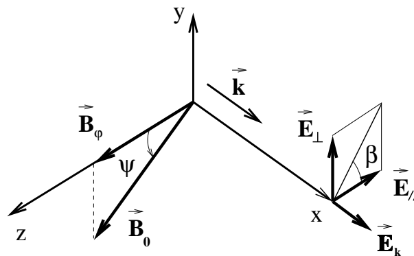
FIG. 3.9 – Configuration g om trique pour l' tude des effets du cisaillement magn tique.
