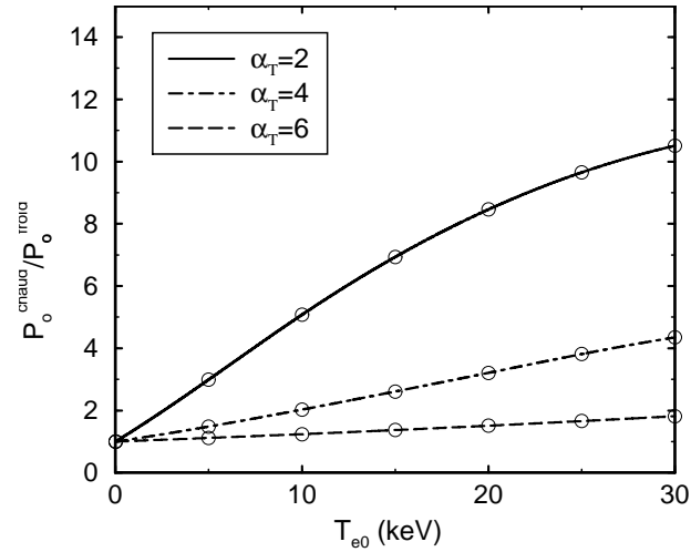
FIG. 3.21 – Variation du rapport entre la puissance ordinaire dans le cas chaud et dans le cas froid, en fonction de la température centrale T_{e0} , pour différentes formes du profil de température. On a ici n_{e0} = 5 \times 10^{13} \text{cm}^{-3} , \alpha_n = 2 et B_0(0) = 2.1 \text{T} .
