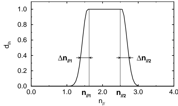
FIG. 5.6 – Forme du coefficient de diffusion quasilinear associé à l'onde hybride basse. Ce coefficient est constant entre n_{\parallel 1} et n_{\parallel 2} et décroît exponentiellement en dehors de l'intervalle [n_{\parallel 1}, n_{\parallel 2}] .
