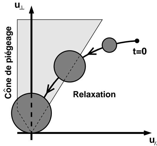
FIG. 2.15 – Illustration des effets d’électrons piégés au cours de la relaxation des électrons excités. Les disques grisés schématisent l’élargissement du nuage électronique au cours de la relaxation collisionnelle.
