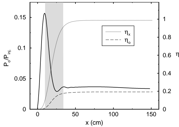
FIG. 3.23 – Rapport de la puissance ordinaire générée sur la puissance injectée, dans le cadre d'une absorption périphérique. On a ici n_{e0} = 5 \times 10^{13}\text{cm}^{-3} , T_{e0} = 10\text{keV} , B_0(0) = 2.8\text{T} . Sur cette figure, on a également fait figurer la fraction de puissance absorbée ( \eta ) des deux modes ( échelle de droite ). La partie grisée représente la zone d'absorption.
