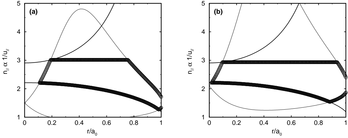
FIG. 5.12 – Domaine de propagation de l'onde hybride basse pour n_{||0} = 1.5 (a) et n_{||0} = 2.1 (b). Les conditions de plasma sont telles que n_{e0} = 3 \times 10^{13} \text{cm}^{-3} , T_{e0} = 5 \text{keV} et q_0 = 1 .
