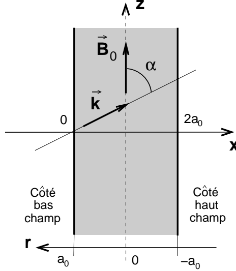
FIG. 3.1 – Configuration slab. Le champ magnétique est selon \hat{\mathbf{e}}_z et le rayon se propage dans le plan (\hat{\mathbf{e}}_x, \hat{\mathbf{e}}_z) . L'axe \hat{\mathbf{e}}_y est perpendiculaire à la page, dirigé vers le bas. Le côté haut champ est à droite de cette figure et l'onde est injectée du côté bas champ.
