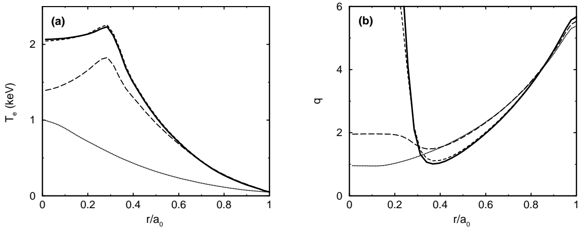
FIG. 6.6 – Idem à la figure 6.4, avec des conditions initiales correspondant à un plasma ohmique simulé par le code ASTRA ( voir texte ). Trait pointillé fin : condition initiale; Tirets longs : première itération; Tirets courts : deuxième itération (difficilement visible); Trait plein épais : troisième itération, correspondant à l'état final.
