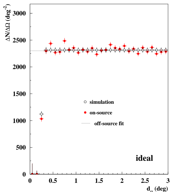
FIG. 6.12: Densité d'événements du signal (points pleins) et d'une simulation à partir d'une distribution plate (points ouverts) en fonction de d_\alpha pour \sigma_{in} = 0^\circ .
