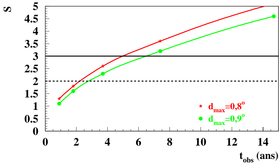
FIG. 6.16: Significence de détection de l'effet de l'ombre de la Lune en fonction du temps pour deux intervalles d'intégration (voir le texte).
