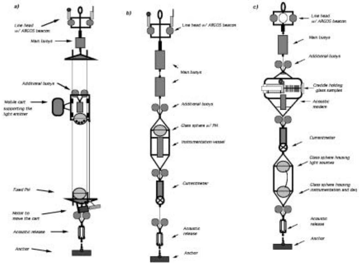
FIG. 3.2: Lignes de test pour l'étude de : (a) l'atténuation de la lumière dans l'eau, (b) le bruit de fond optique et (c) la bioalissure (de [63]).
