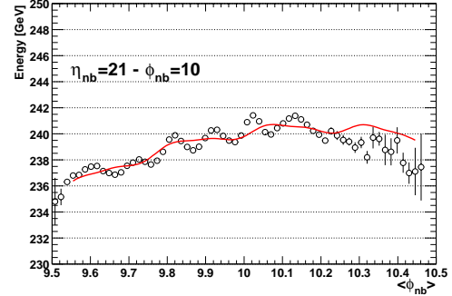
FIG. 5.4 – Energie reconstruite en fonction du barycentre \bar{\phi} dans la cellule ( \eta_{nb} = 21, \phi_{nb} = 10 ).
