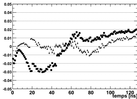
FIG. 4.40 – Résidus de l'ajustement de la forme prédite (valeur de LC fixées par les mesures) avec la méthode de la convolution pour la cellule \eta_{nb} = 19 , \phi_{nb} = 10 avec les données des tests en faisceau du module M10 dans le cas où le temps t_0^{phy} est ajusté (triangles) ou en avance de 1 ns sur la valeur ajustée (carrés).
