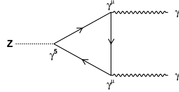
FIG. 1.6 – Boucle triangulaire fermionique qui peut causer des anomalies.
