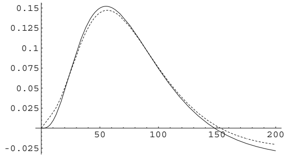
FIG. 4.2 – Réponses théoriques à un signal de physique (trait plein) et d'étalonnage (pointillés) après mise en forme. Les paramètres utilisés sont C_d = 1.5 \text{ nF} , L_d = 20 \text{ nH} , \tau_s = 15 \text{ ns} , t_d = 400 \text{ ns} et \tau_{exp} = 365 \text{ ns} .
