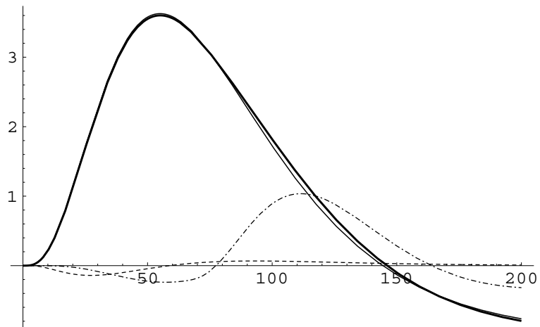
FIG. 4.14 – Composantes des différents termes de réflexions dans la ligne de lecture pour le signal de physique. La ligne fine est la forme sans réflexions U_{\text{phy}}^0(t) , la ligne en tirets est le terme A(t) ( \times 10 ), la ligne tiret-pointillé est la composante B(t) ( \times 10 ). La ligne en gras est la somme de toutes les composantes, U_{\text{phy}}(t) .
