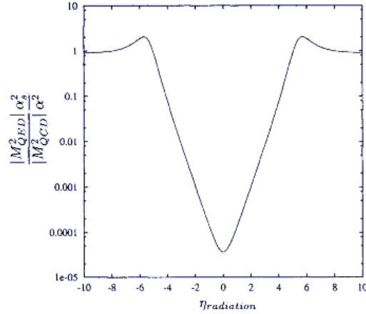
FIG. 6.8 – Rapport du carré des éléments de matrices, pour le processus qq' \rightarrow qq'g en fonction de la pseudo-rapidité du gluon radié et pour des quarks diffusés à \eta = \pm 5 , pour un échange de photon et gluon [74].
