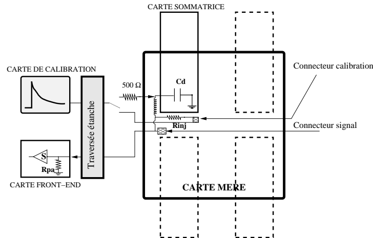
FIG. 4.8 – Schéma de principe des tests électriques réalisés sur la maquette. Les deux voies d'injection du signal sont représentés: par le circuit d'injection d'étalonnage ou directement au niveau de la capacité C_d .
