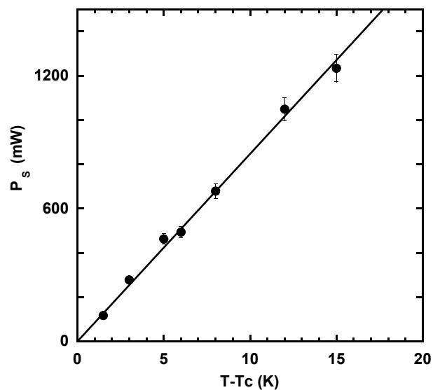
FIG. 6.21 – Puissance seuil P_S en fonction de l'écart à la température critique T - T_C pour un faisceau de rayon au col \omega_0 = 3.5\mu\text{m} . La variation est linéaire en T - T_C comme le montre la régression effectuée sur les données (droite en trait plein).
