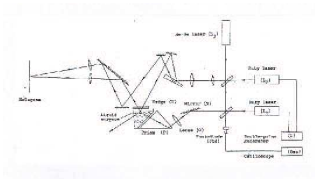
FIG. 2.14 – Schéma de principe des expériences de déformations d'une interface eau/air réalisées par Ostrovskaia et al. [159]. On notera que, comme dans les expériences de la référence [157], l'interface est illuminée en réflexion totale afin de maximiser les effets de la pression de radiation.
