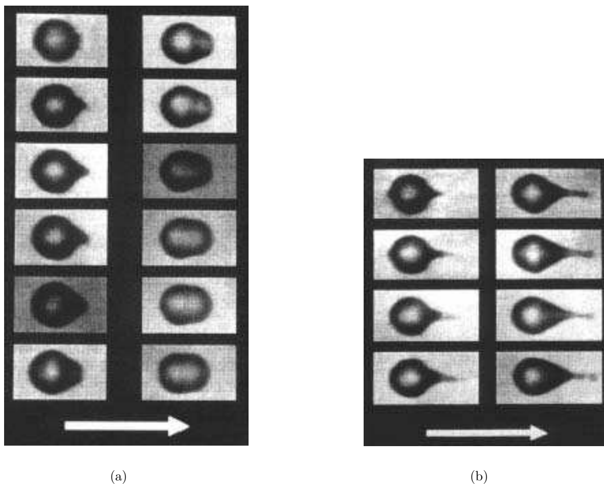
FIG. 2.16 – (a) Evolution temporelle de la déformation d'une gouttelette d'eau de rayon a = 50\mu\text{m} (milieu environnant:air) après passage d'une impulsion d'énergie 100 mJ et de durée 400 ns issue d'un laser à colorant. L'impulsion se propage de gauche à droite comme indiqué par la flèche. La première image en haut à gauche correspond à l'instant t=0 , la dernière en bas à droite à t = 22\ \mu\text{s} après le passage de l'impulsion. (b) Déformations observées pour une impulsion d'énergie 200 mJ. La première image correspond à l'instant t = 1\ \mu\text{s} , la dernière à t = 15\ \mu\text{s} . On notera la formation d'un filament et l'éjection de matière en face avant de la goutte. Les images sont issues de la référence [161].
