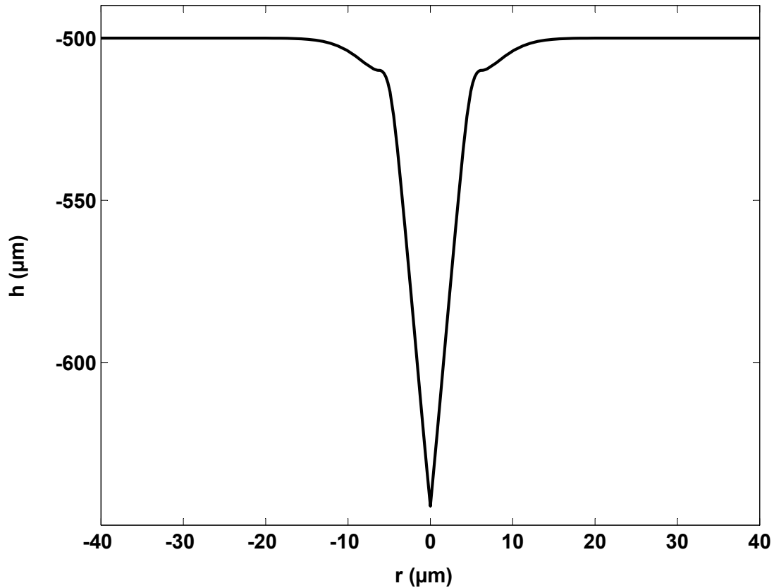
FIG. 6.13 – Zoom sur le profil de déformation simulé à la puissance laser P = 480 \text{ mW} sur la figure (6.12)). L'épaule caractéristique de part et d'autre de la pointe centrale de la déformation est clairement visible. On pourra comparer avec le profil expérimental correspondant de la figure (6.4).
