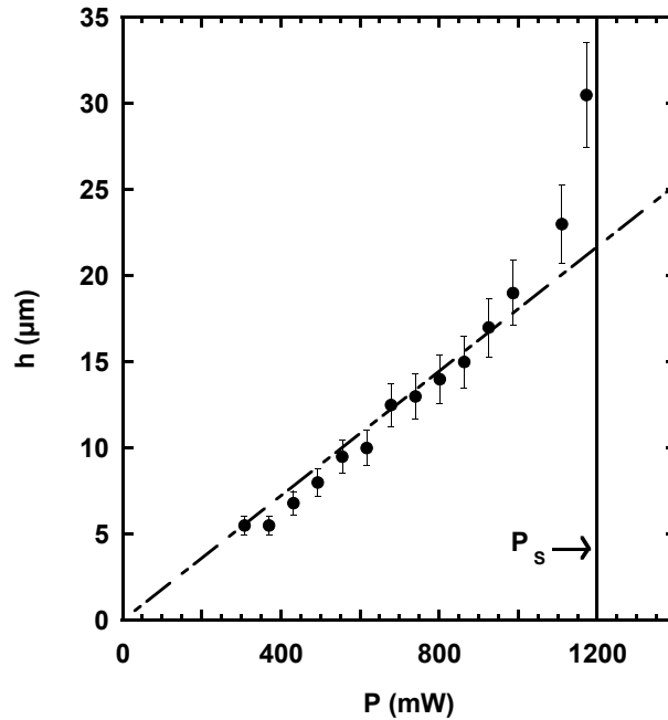
FIG. 6.17 – Evolution de la hauteur stationnaire de la déformation en fonction de la puissance laser P , pour les profils de la figure (6.16): T - T_C = 15K et \omega_0 = 3.5\mu m . La courbe en pointillés indique la régression linéaire effectuée pour les puissances les plus basses: l'évolution de la hauteur est bien linéaire en fonction de la puissance et la pente correspondante a été exploitée dans les résultats du paragraphe (5.3). On constate que la hauteur s'écarte du comportement linéaire aux hautes puissances pour finalement diverger. Le trait vertical marque le seuil en puissance P_S au-delà duquel l'interface devient instable et conduit à la formation du long filament présenté sur la figure (6.15).
