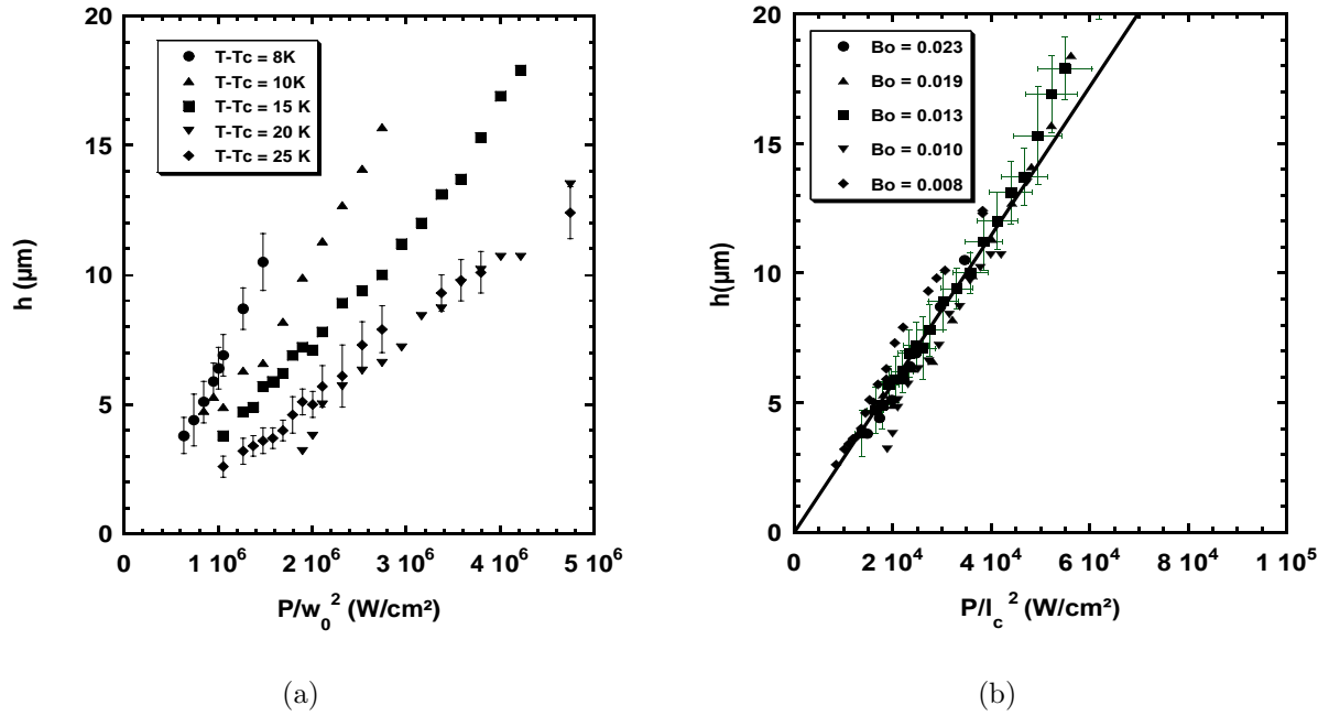
FIG. 5.4 – (a) Variation expérimentale de la hauteur de la déformation sur l'axe en fonction de \frac{P}{\omega_0^2} dans le régime Bo \ll 1 . Le rayon du faisceau vaut \omega_0 = 5.3\mu\text{m} et les écarts à la température critique (T - T_C) = 8\text{K}(\bullet), 10\text{K}(\blacktriangle), 15\text{K}(\blacksquare), 20\text{K}(\blacktriangledown), 25\text{K}(\blacklozenge) . (b) Mêmes données qu'en (a), mais reportées en fonction de \frac{P}{I_c^2} . Les nombres de Bond correspondants aux différentes températures sont donnés en encart. La droite est un ajustement linéaire des données validant la loi théorique (5.40).
