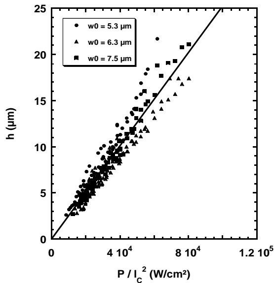
FIG. 5.7 – Loi d'échelle en \frac{P}{l_c^2} dans le régime Bo \ll 1 , pour les rayons de faisceau \omega_0 = 5.3, 6.3 et 7.5\mu\text{m} . Conformément à l'équation (5.40) la pente est, aux incertitudes expérimentales près, indépendante du rayon du faisceau, comme illustré par la droite obtenue par une régression linéaire sur l'ensemble des données.
