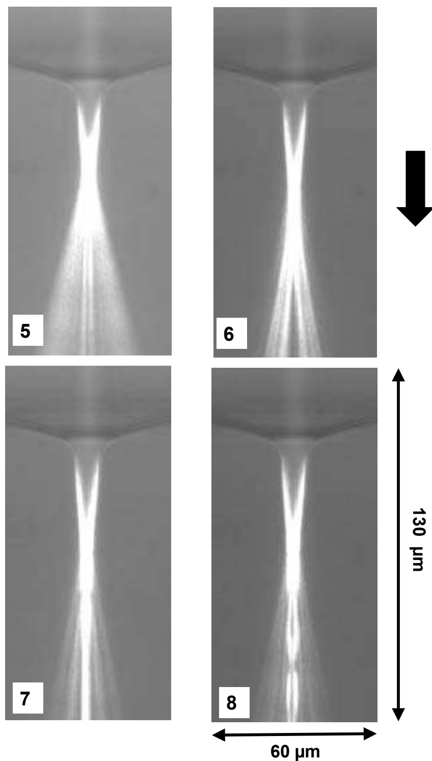
FIG. 6.25 – Suite de la série temporelle d'images de la figure (6.24): 5) t = 2.8s , 6) t=3.6s , 7) t=4s et 8) t=7.2 s après le début de l'illumination. On observe la forte focalisation du faisceau laser incident à l'intérieur du filament liquide.
