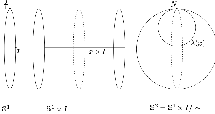
FIG. IV.1 – Le lacet \lambda(x) .
