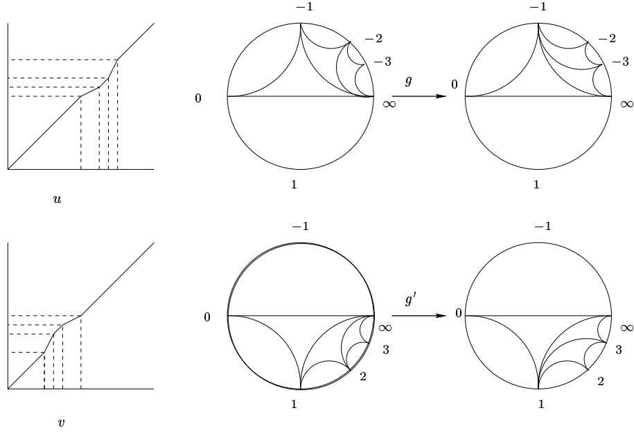
FIG. IV.2 – Le cycle générateur de H_2(\tilde{T}) .
