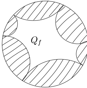
FIG. I.3 – Prolongement d'un élément de CPP .
