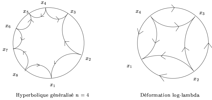
FIG. I.4 – Hyperboliques généralisés pour n = 4 et n = 2 .
