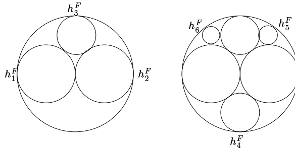
FIG. I.2 – Bracelet de Ford partiel.
