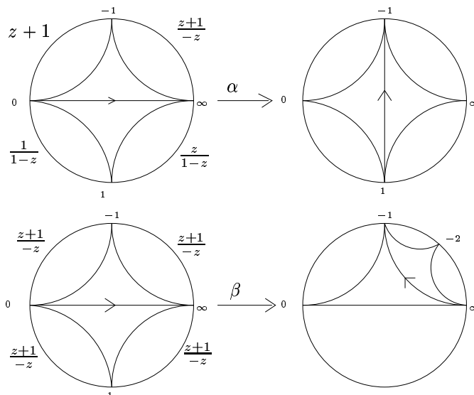
FIG. 2 – Deux éléments version CPP.
