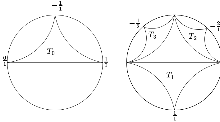
FIG. I.1 - Triangulation de Farey partielle.
