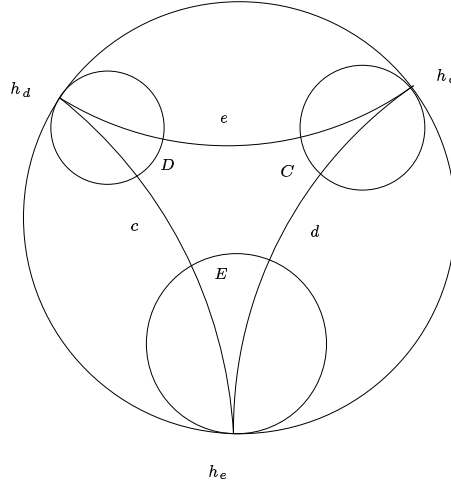
FIG. II.4 – Triangle géodésique décoré.
