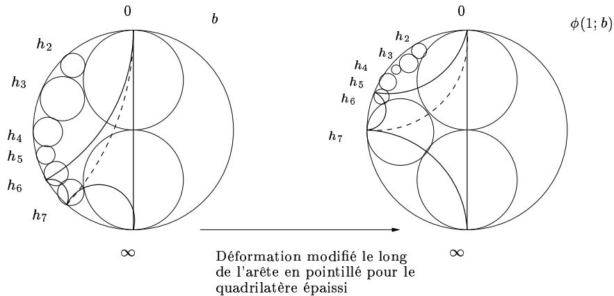
FIG. II.3 – Déformation log-lambda modifié.
