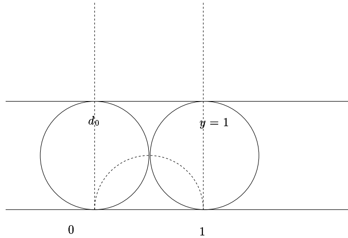
FIG. II.5 – Un triplet d'horocycles tangents deux à deux.
