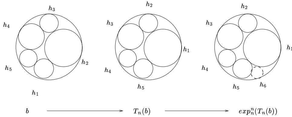
FIG. III.2 – Une rotation de bracelet suivie d'une extension.
