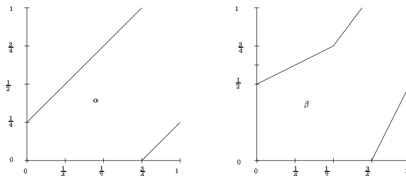
FIG. 1 – Deux éléments version PL.
