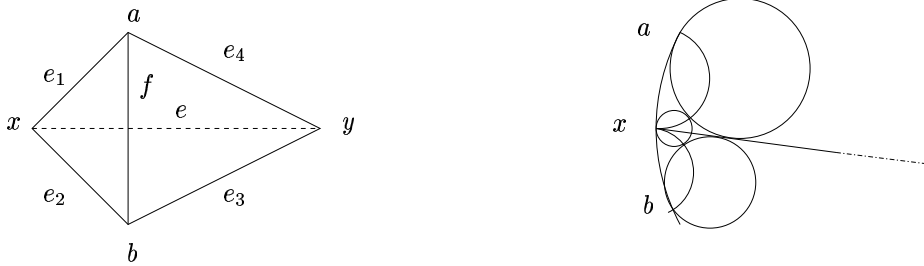
FIG. III.1 – Formule de Ptolémée.
