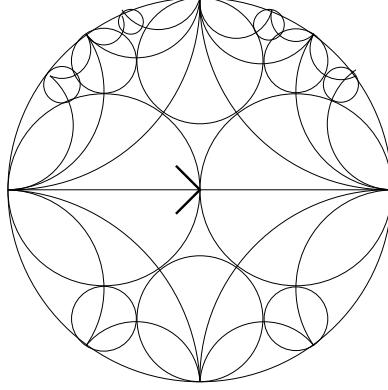
FIG. I.7 – Tessellation décorée de Farey-Ford.
