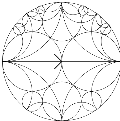
FIG. 3 – Tessellation décorée de Farey-Ford.
