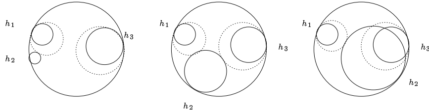
FIG. II.1 – Unicité de h_2 .
