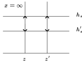
FIG. I.5 – Distance de deux horocycles.
