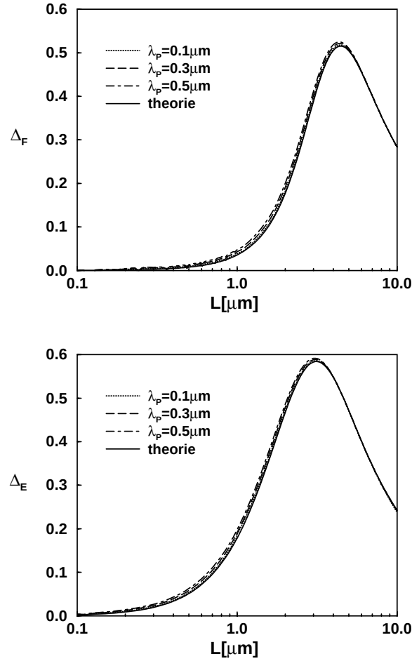
FIG. 4.5 – Les facteurs de corrélation représentés pour la force (courbes du haut) et pour l'énergie (courbes du bas) après le rééchantillonnage décrit par l'équation (4-26). Différentes longueurs plasma correspondent à des courbes quasiment identiques, représentées en traits plein, tiret et pointillés. Ces courbes coïncident presque parfaitement avec les expressions analytiques dérivées en (4-45) et représentées ici par les courbes en trait gras.
