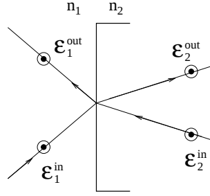
FIG. 1.3 – Diffusion sur une interface entre deux milieux.
