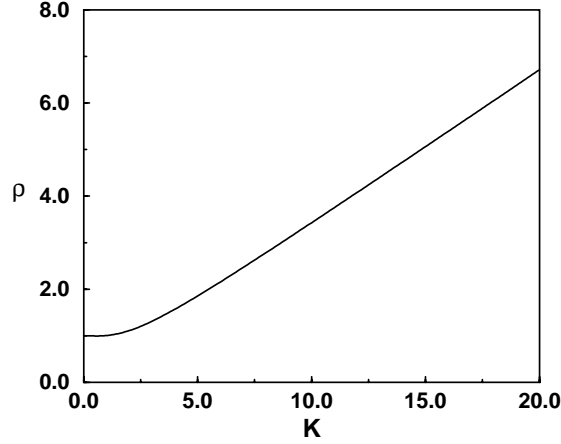
FIG. 6.3 – Fonction \rho[K] en fonction de K = |\mathbf{k}|L , caractérisant la sensibilité de l'énergie de Casimir vis-à-vis de la longueur d'onde du spectre de rugosité de surface. On distingue clairement deux régimes de comportement à petit et grand K .
