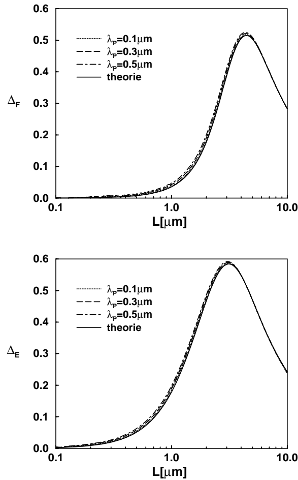
FIG. 4.5 – Les facteurs de corrélation représentés pour la force (courbes du haut) et pour l'énergie (courbes du bas) après le rééchelonnement décrit par l'équation (4-26). Différentes longueurs plasma correspondent à des courbes quasiment identiques, représentées en traits plein, tiret et pointillés. Ces courbes coïncident presque parfaitement avec les expressions analytiques dérivées en (4-45) et représentées ici par les courbes en trait gras.
