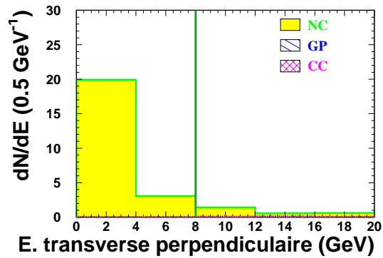
FIG. 5.8 – Distribution prédite de l'énergie transverse perpendiculaire au jet du photon identifié comme tel (deux lignes du haut) ou identifié comme un électron (deux lignes du bas) pour les événements des échantillons de contrôle passant les critères de sélection sur l'énergie transverse manquante et l'angle du photon. Les figures de gauche montrent la distribution globale, celle de droite ont une échelle plus petite permettant de mieux voir l'effet du critère de sélection sur l'énergie transverse du photon. Pour chaque paire de lignes, les figures de la ligne du haut montrent le signal à différentes masses, celles de la ligne du bas, les bruits de fond prédits par le modèle standard.
