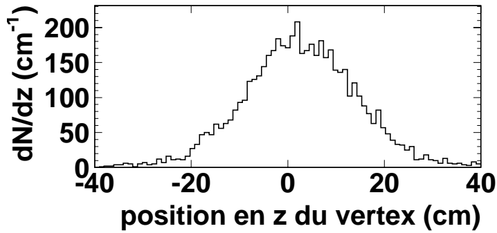
FIG. 3.13 – Distribution suivant z du vertex d'un échantillon de données de la préselection H1 France.
