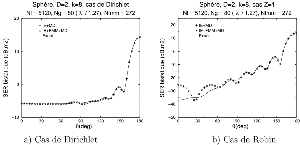
FIG. 8.2 – \mathcal{C}(\text{IE}+\text{MD}) - \mathcal{C}(\text{IE}+\text{MD}+\text{FMM}) , pour k = 8
