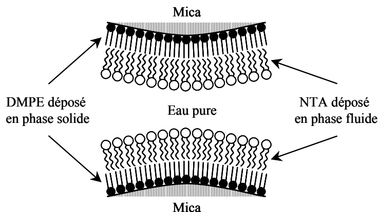
Figure III-5 : Configuration expérimentale permettant l'étude en SFA de l'énergie d'interaction entre deux monocouches de lipide NTA plongées dans l'eau pure. Le lipide DMPE est déposé en phase solide à 38 mN/m et le lipide NTA est déposé en phase fluide à 35 mN/m. La bicouche est supportée par une surface de mica moléculairement plane.
