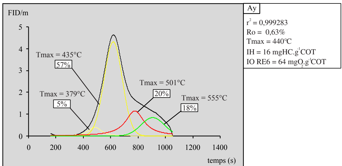
Figure VII.4 : décompositions de pyrogrammes de 3 échantillons du Détroit de Rodez présentant des degrés d'oxydation croissant
