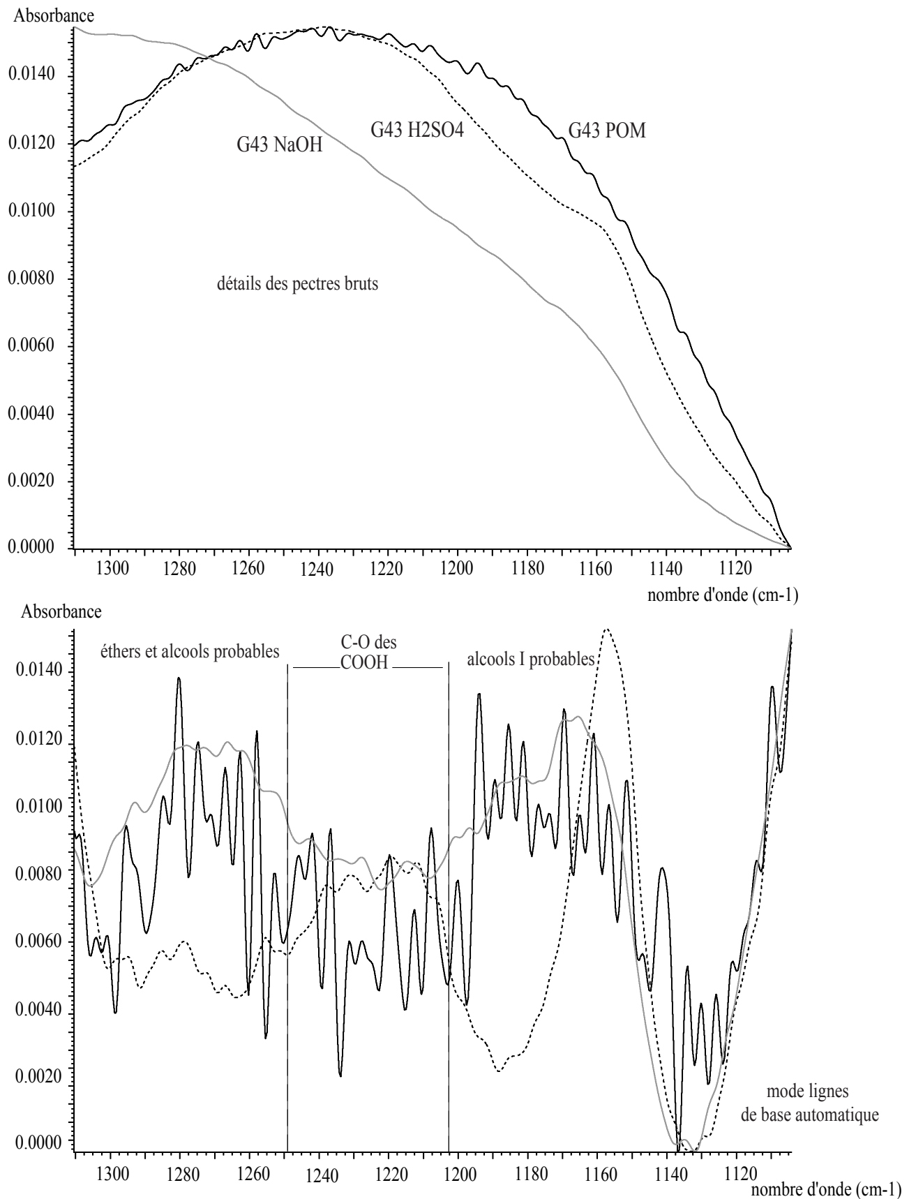
Figure V.29 : détails du massif 1300-1130 \text{cm}^{-1} des fractions POM, NaOH et H 2 SO 4 de l'échantillon G43
