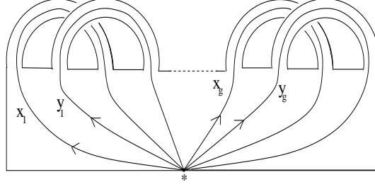
FIG. 2.1 – Les courbes (x_i, y_i)_{i=1}^g sur \Sigma_{g,1}
