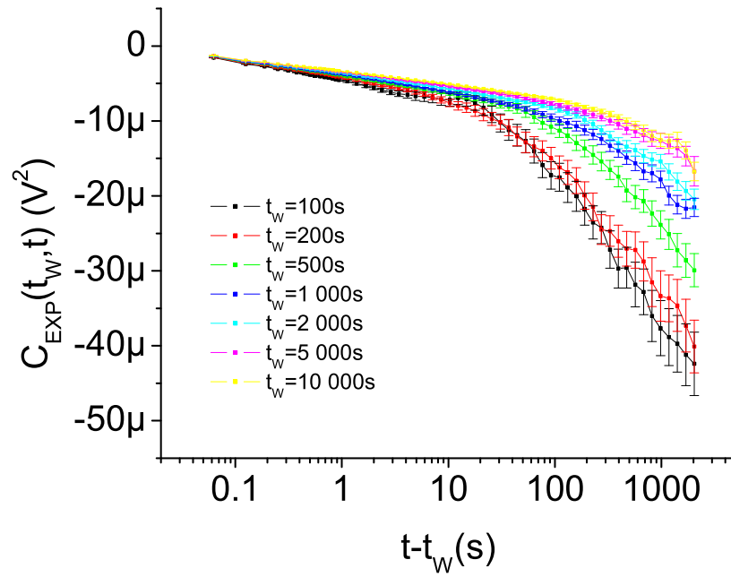
FIG. 4.4: Fonctions d'autocorrélation expérimentales avec un offset commun à tous les t_w , C_0 : C_{exp}(t_w, t) - C_0 = \langle v(t_w)v(t) \rangle - \langle v^2(t_w) \rangle . L'étalement des courbes est comparable à celui de l'aimantation thermo-rémanente (cf. figure 4.2). Les barres d'erreur représentées dénotent de l'incertitude statistique résiduelle, après l'ensemble des moyennes.
