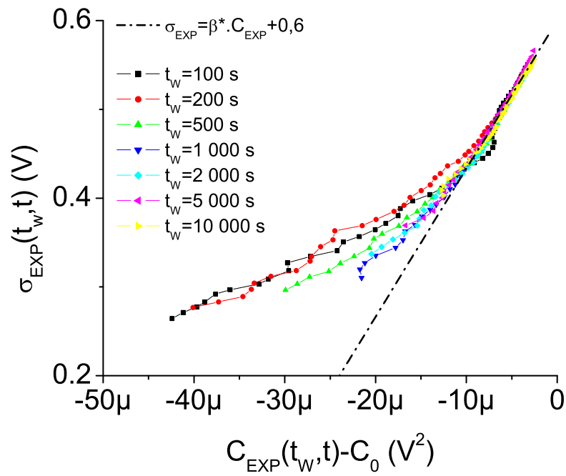
FIG. 4.5: Plot FDT en grandeurs expérimentales. La pente de la droite en trait mixte est calculée à partir de l'étalonnage par le barreau de cuivre pour une température de 13,3 K, la température de travail. Le régime linéaire correspond aux différences de temps les plus courtes, et sur ces échelles de temps, la relation linéaire prédite par le théorème de fluctuation-dissipation est recouverte, en parfait accord avec un scénario à faible brisure d'ergodicité.
