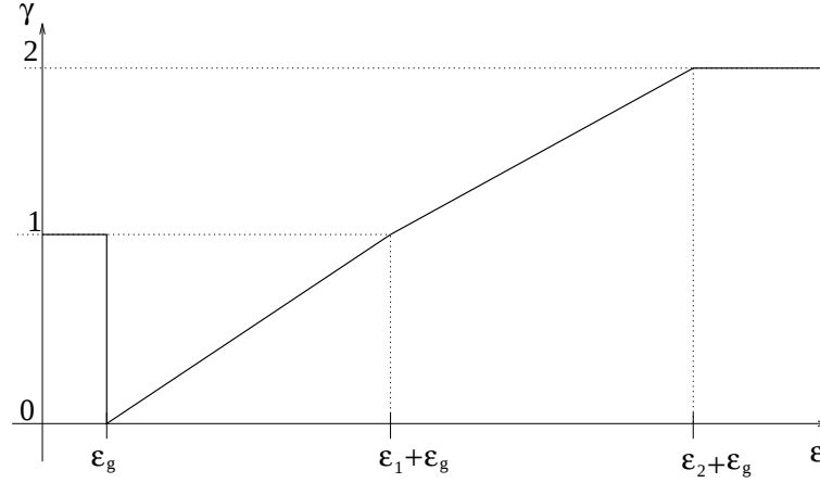
FIG. 1.4 – Nombre moyen d'électrons réémis par la paroi. Dans notre modèle nous avons approximé les données expérimentales par une fonction affine par morceaux. \varepsilon_g , \varepsilon_1 et \varepsilon_2 suffisent à représenter cette fonction.
