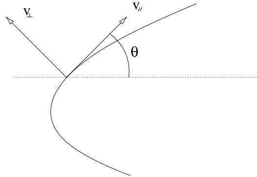
FIG. 5.1 – Base naturelle le long d'une ligne de champ magnétique
