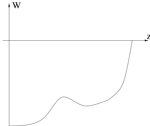
FIG. 1.11 – Minima locaux de l'énergie totale dans le cas où le champ électrique présente des rebroussements.
