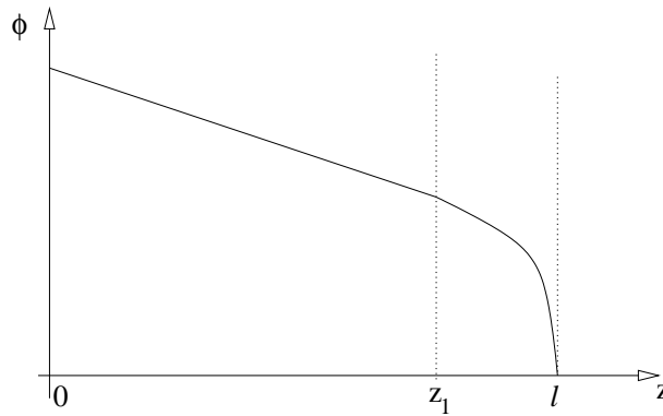
FIG. 1.9 – Représentation du potentiel électrique tel que le champ électrique E = -\frac{\partial\phi}{\partial z} a l'allure donnée par la figure 1.8. Pour z \in [0, z_1] , le potentiel électrique est une fonction affine, puis est donné par un arc de parabole pour z \in [z_1, l] . Par convention, \phi(l) = 0 , aussi \phi(0) = \phi_{max} le potentiel total appliqué.
