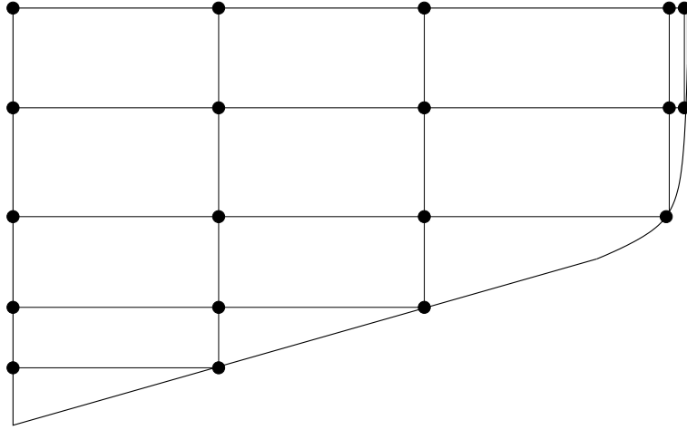
FIG. 1.13 – Maillage défini par les intersections \tilde{x}_{W_i} des droites W = W_i et de la courbe W = -\phi(z) .
