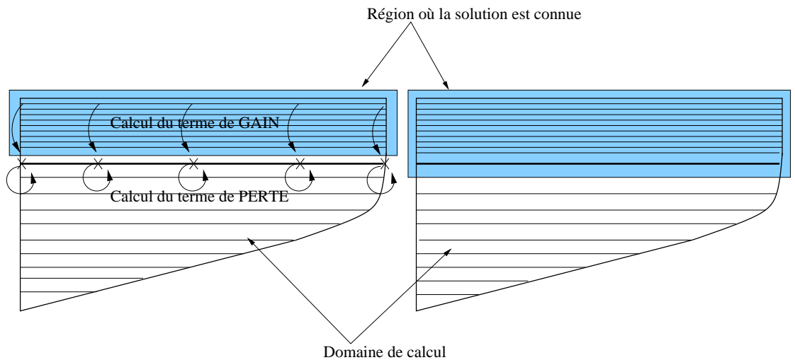
(b) résolution (calcul de la solution sur le niveau)
