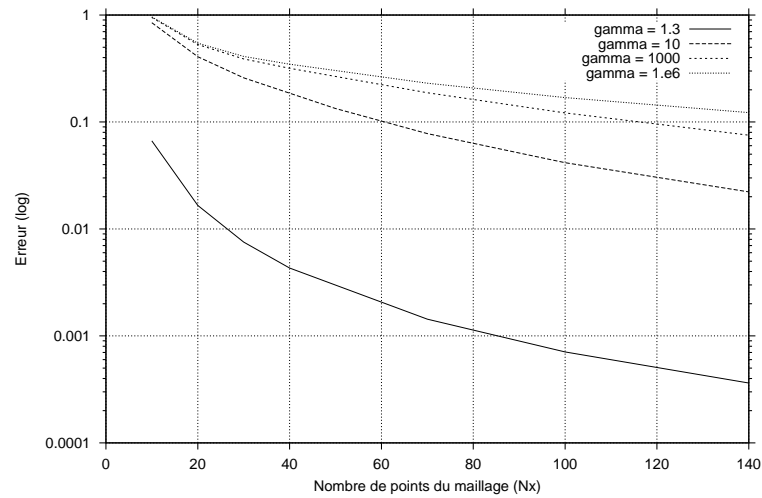
FIG. 5.8 – Décroissance de la norme l^\infty de l'erreur entre la solution théorique W_0 et la solution calculée. Les ordonnées sont en échelle logarithmique.
