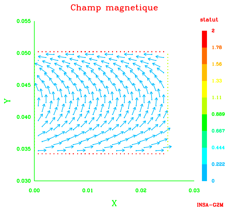
FIG. 5.6 – Champ magnétique choisi pour les tests. Sa norme est constante et il est aligné avec l'axe des x le long des bords où l'on impose une condition de Neumann. La variable en couleurs statut indique si un sommet fait partie du maillage, d'un bord Dirichlet ou d'un bord Neumann.
