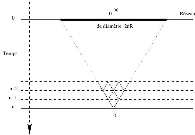
FIG. 2.1 – Ensemble \overline{\{0\}}^{(n)} des sites de \mathbb{Z}^d à l'instant 0 ayant une influence potentielle sur la valeur du spin à l'origine au temps n
