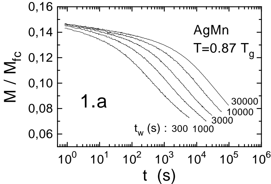
FIG. -7 – Aimantation thermorémanente en fonction du temps pour différents temps d'attente t_w pour un échantillon d'AgMn 2.6%, d'après (Vincent et al., 1997).
