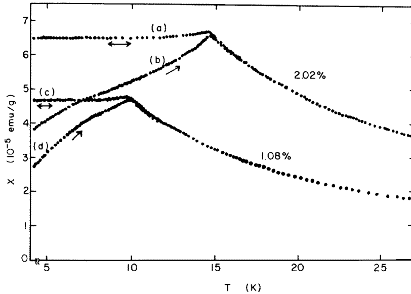
FIG. -6 – Mesure de susceptibilité pour deux alliages CuMn avec 1.08 et 2.02 % de Mn. Les courbes (a) et (c) ont été obtenues en refroidissant avec le champ magnétique appliqué (FC) alors que (b) et (d) sont obtenues en refroidissant puis en appliquant le champ (ZFC) (Nagata et al., 1979)
