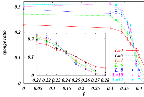
FIG. V-9 – Fraction d'excitation spongieuse en fonction de \rho dans le FNM. (l'insertion montre les données pour le SNM), indiquant \rho_{RSB}^{FNM} = 0.380 \pm 0.005 ( \rho_{RSB}^{SNM} = 0.235 \pm 0.005 ).
