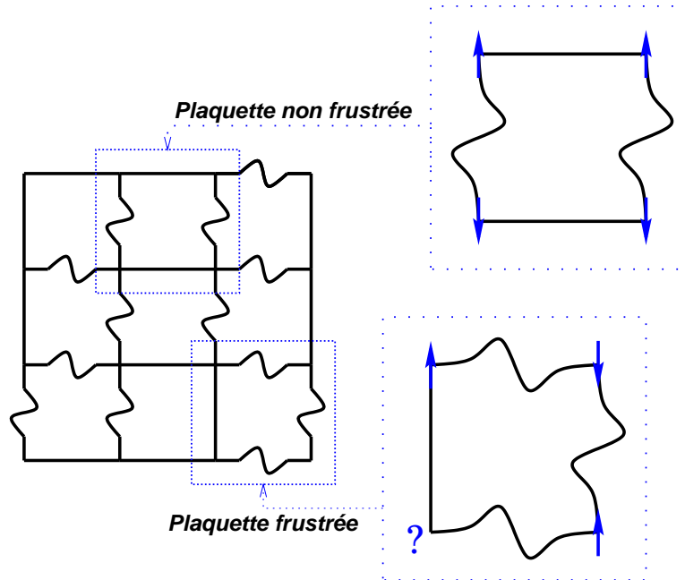
FIG. -5 – Exemple de système frustré par le désordre des interactions: le réseau carré avec interactions \pm J aléatoires. Les liens tordus sont des (-) et les liens droits des (+).
