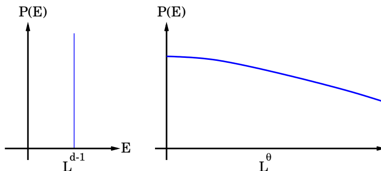
FIG. I-8 – Probabilité d'obtenir une excitation d'énergie E à une taille l donnée dans les ferromagnétiques et dans les verres de spins selon le modèle des gouttelettes. Dans le cas d'un verre de spins, la probabilité d'obtenir une excitation d'énergie nulle décroît en L^{-\theta} , contrairement au cas ferromagnétique, même désordonné, où cette probabilité est nulle.
