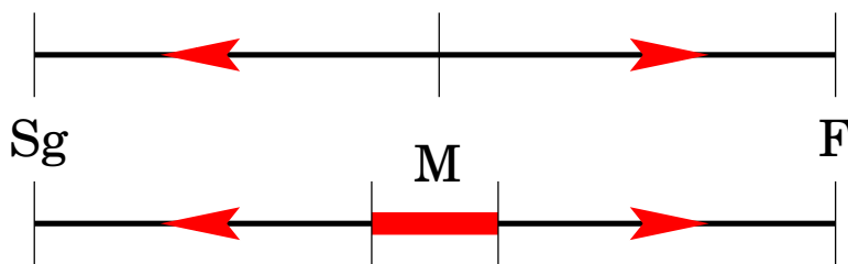
FIG. V-1 – Haut: flot de renormalisation dans l'hypothèse où il y a deux points fixes attractifs verre de spins et ferromagnétique et un point fixe instable. Bas: une phase mixte entraîne ainsi l'existence d'une ligne de points critiques dans le diagramme de phase, comme dans le modèle XY en 2d .
