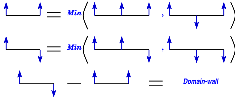
FIG. II-5 – Lors d'une itération, on calcule la nouvelle énergie pour le lien effectif parallèle et anti-parallèle. La différence entre ces deux énergies représente l'énergie de domaine à cette échelle.
