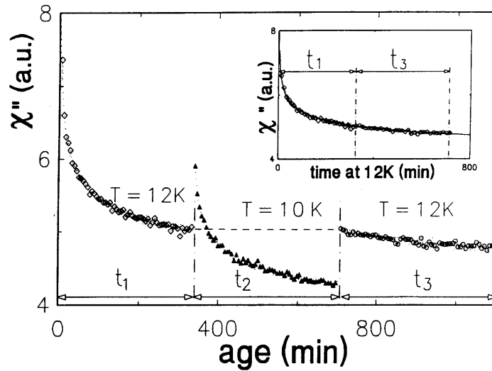
FIG. -9 – Effet d'un cycle négatif en température \Delta T = 2K sur la susceptibilité \chi'' du CdCr_{1.7}In_{0.3}S_4 , d'après (J.Hammann et al., 2000).
