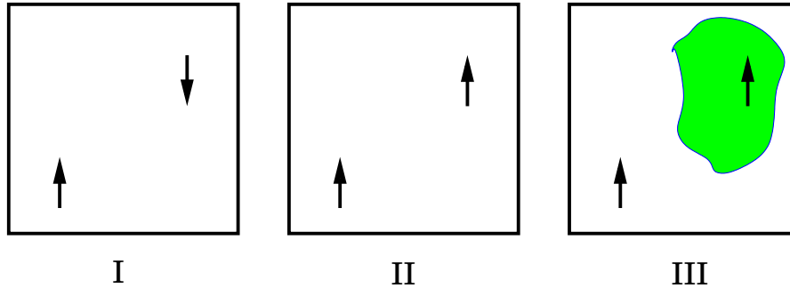
FIG. IV-1 – Représentation de la méthode utilisée pour trouver les états excités.
