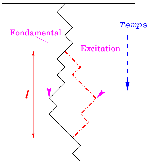
FIG. II-2 – Une marche aléatoire dirigée vers le bas dans un milieu désordonné est une bonne représentation du DPRM. Une fois que le meilleur chemin est trouvé, les excitations de taille l ont une énergie en l^{1/3} .
