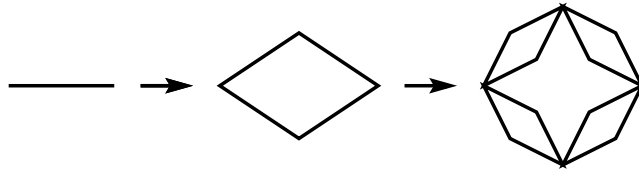
FIG. II-4 – Si l'on définit un réseau hiérarchique de la façon suivante, en transformant 1 lien en b branches de \ell segments, le calcul de la fonction de partition est équivalent à l'approximation de Migdal-Kadanoff pour un réseau hyper cubique. Ici le cas correspondant à d=2 .
