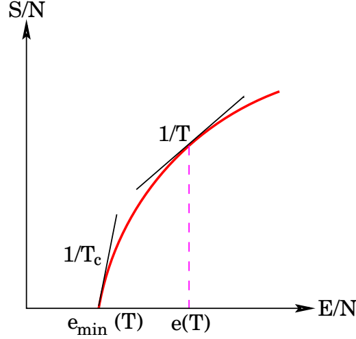
FIG. II-1 – Logarithme du nombre de configurations (entropie configurationnelle) en fonction de l'énergie dans le REM. En dessous d'une valeur critique, il n'y a plus d'états et le système reste piégé dans l'état d'énergie la plus basse. La tangente donne l'inverse de la température. Ce scénario qui apparaît dans le REM est la transition vitreuse idéale
