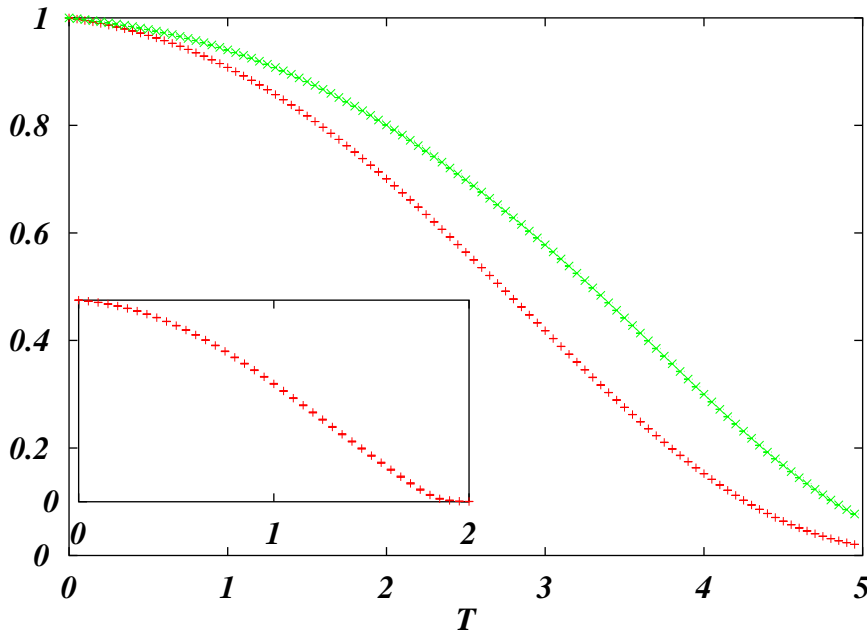
FIG. III-5 – q_{EA} et q_T, T = 0 (au dessus) pour un état issu d'un fondamental à L = 10 en 3 - d . On a alors T_c \approx 5 tandis que le même genre de plot est trouvé en SK avec cette fois T_c \approx 2 (l'inset montre q_{EA} dans le modèle SK)
