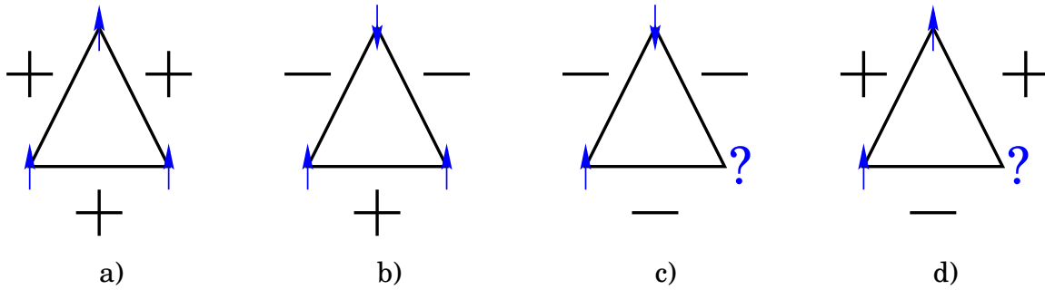
FIG. -2 – Quelques solutions possibles aux problèmes posés. Dans les cas c) et d), il est impossible de satisfaire les trois personnes à la fois, et l'une d'elle se retrouve frustrée.
