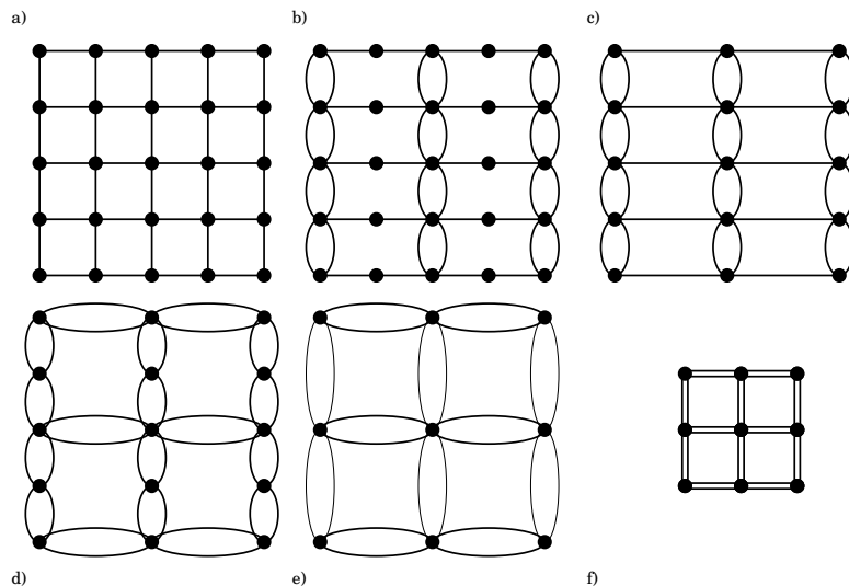
FIG. II-3 – La procédure de renormalisation de Migdal-Kadanoff pour un réseau carré. D'abord (a) b-1 liens parallèles à l'axe y sont cassés et déplacés vers la droite (b) pour créer des nouveaux liens effectifs avec une nouvelle valeur de couplage. Ensuite (c) les b-1 sites non connectés avec les nouveaux liens sont décimées. Le processus est ensuite répété pour l'axe des x (d et e) et enfin on change l'échelle de longueur pour revenir à un problème équivalent à celui considéré initialement, mais avec des valeurs de couplages renormalisées (f).
