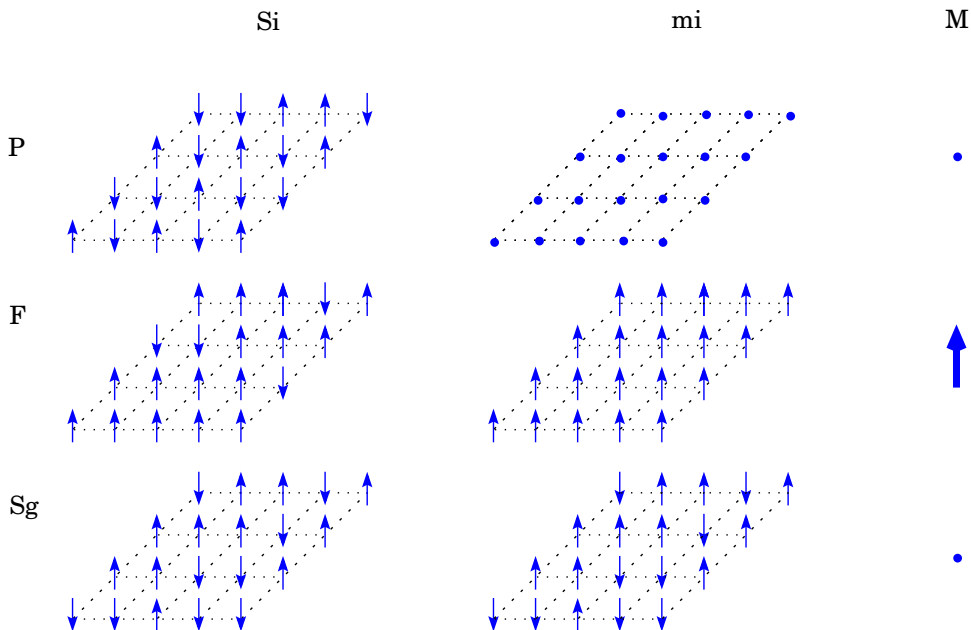
FIG. I-1 – De gauche à droite : états des spins à un instant t , aimantation moyenne par spin et aimantation globale moyenne pour, de haut en bas) un paramagnétique, un ferromagnétique et un verre de spins. Dans ce dernier, l'aimantation moyenne d'un spin donné est non nulle, bien qu'elle soit différente d'un spin à un autre.
