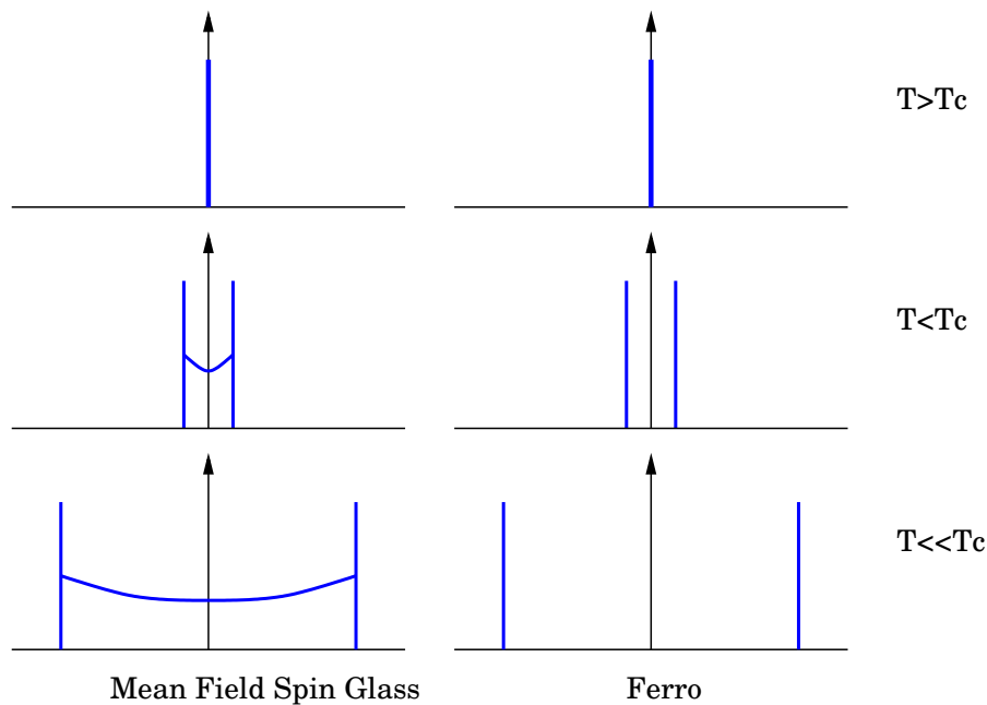
FIG. I-4 – Représentation de la fonction P(q) pour différentes températures dans un verre de spins SK (à gauche) et dans un ferromagnétique (à droite).
