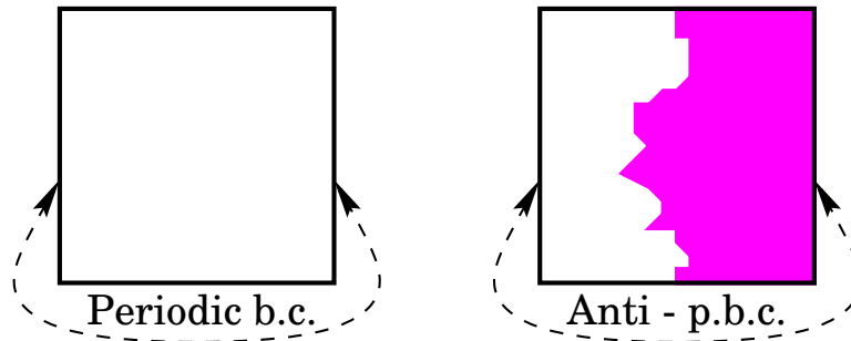
FIG. I-7 – Principe des calculs numériques “Periodic-AntiPeriodic” pour generer une paroi de domaine.
