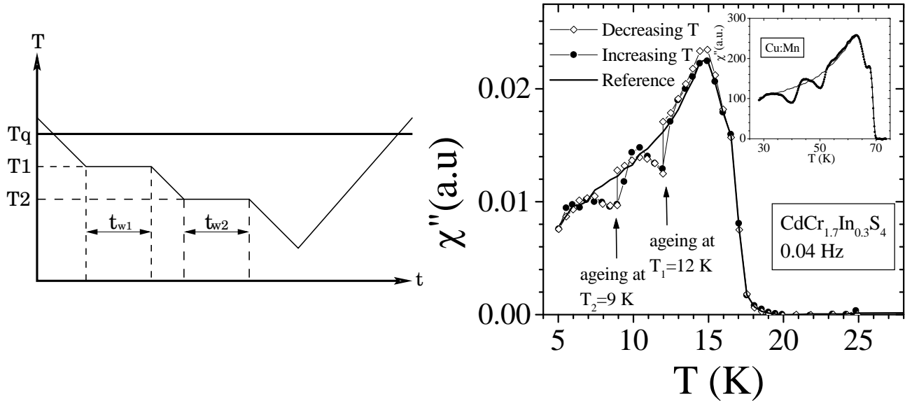
FIG. -10 – A droite : mesure de \chi'' en fonction de la température pour le \text{CdCr}_{1.7}\text{In}_{0.3}\text{S}_4 en suivant la procédure décrite à gauche, avec T_1 = 12\text{K} , T_{w1} = 7\text{h} , T_2 = 9\text{K} , t_{w2} = 40\text{h} , d'après (Jonason et al., 1998).
