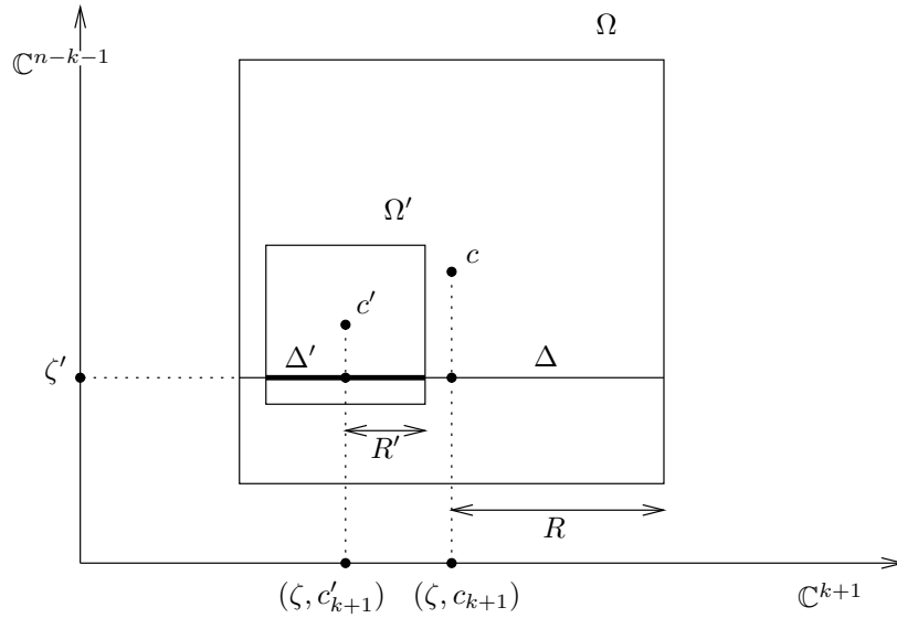
FIGURE 7. Cas 2 : \Omega' et \Omega sont des polydisques de \mathbb{C}^n
