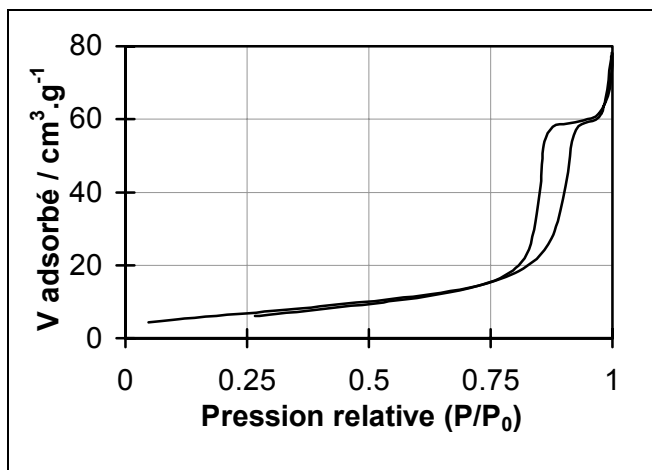
Figure II-8 : Isotherme d'adsorption-désorption pour l'échantillon SnO 2 -HNO 3 calciné à 600°C.
