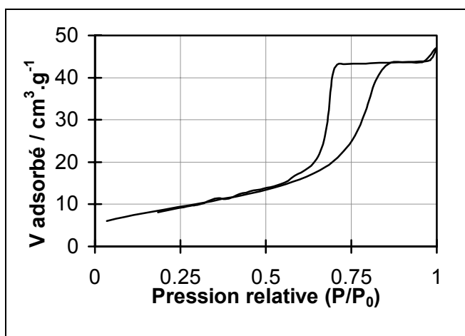
Figure II-2 : Isotherme d'adsorption-désorption pour l'échantillon SnO 2 -NH 3 calciné à 600°C.
